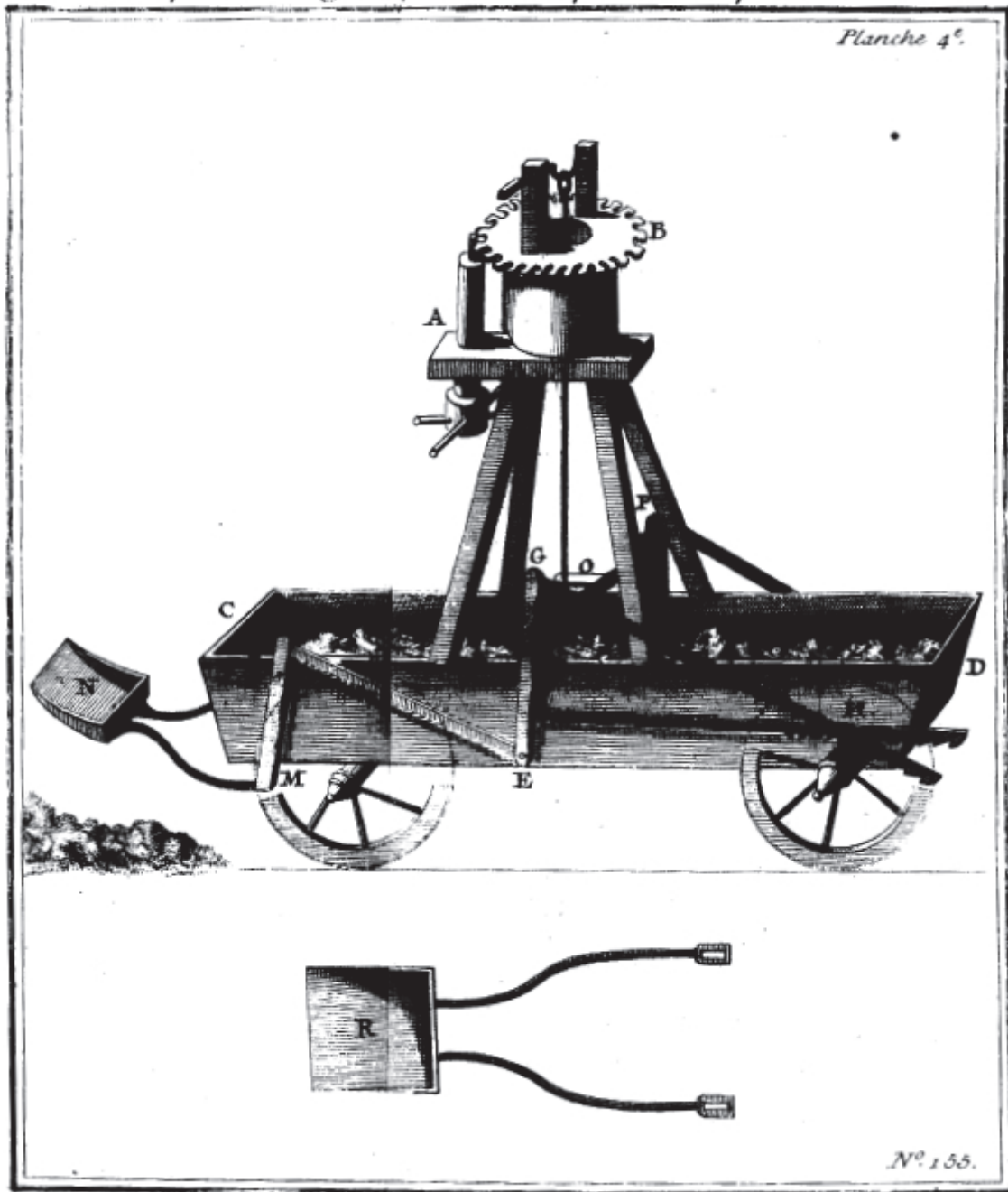
Figure 73 : Tombereau qui se charge et qui marche par le moyen du vent approuvé en 1714 à l'Académie (figure tiré du tome III des Machines, p. 45)
