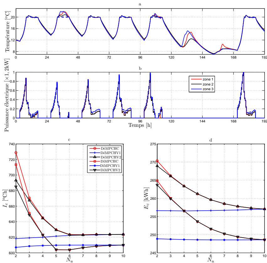
FIGURE 3.14 – Scénario 3 : signaux de sortie (a) et de commande (b) pour les huit premiers jours de l'année et indicateurs de performance (c et d) pour N_{u,i} = \underline{N}_{2,i} \in \mathbb{N}_2^{10} , \bar{N}_{2,i} = 10 , \lambda_i = 1 , \forall i \in \mathbb{N}_1^3
