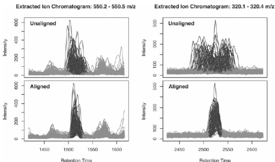
Figure 81 : EIBPC de deux groupes avant et après alignement des temps de rétention [150].
