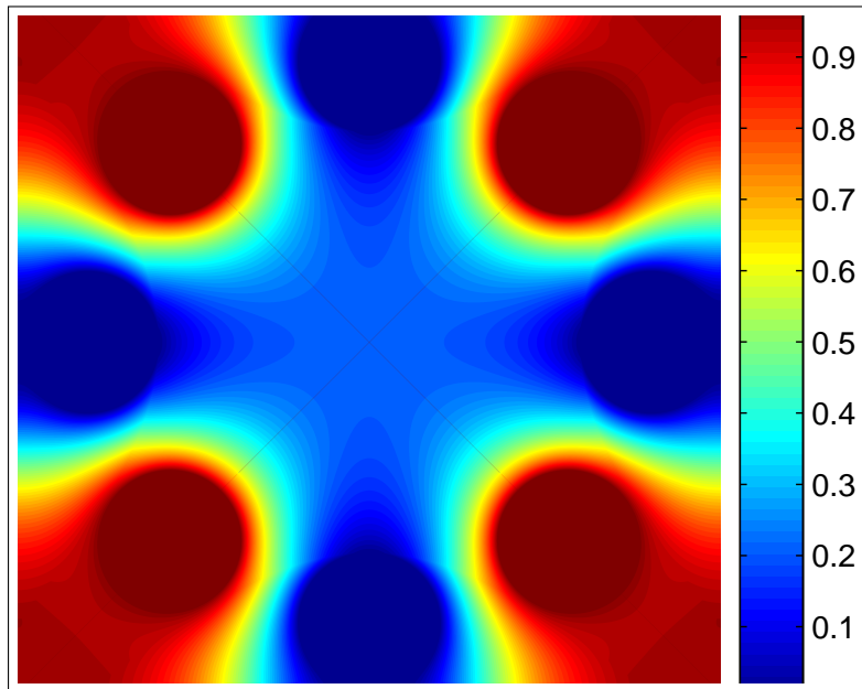
Figure 5.11 – Différence relative (U_4 - \tilde{U}_4)/\tilde{U}_4 entre le potentiel électrique généré par l'octupôle U_4 et celui généré en l'absence des quatre barreaux non connectés, \tilde{U}_4 ; les barreaux non connectés étant situés dans les diagonales de l'image. Calculs réalisés au moyen du logiciel SIMION par J. Pedregosa-Gutierrez.
