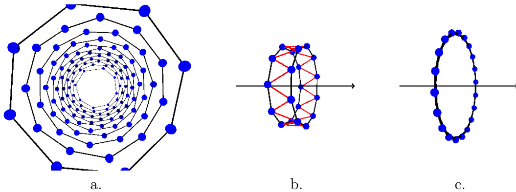
Figure 4.2 – (a) Vue en perspective selon l'axe z d'une structure de 126 ions calculée à l'aide d'un thermostat à 10 mK dans le pseudo-potential d'un octupôle linéaire. Avec le potentiel choisi, la structure obtenue est un tube d'ions formé de 12 anneaux. Tous les anneaux comportent onze ions, à l'exception des anneaux formant les deux extrémités du tube qui en comptent huit. (b) Tube formé de 2 anneaux, les traits rouges permettent de mieux visualiser la position relative des ions. (c) Un unique anneau d'ions. L'axe noir représente la direction longitudinale du piège ( z )
