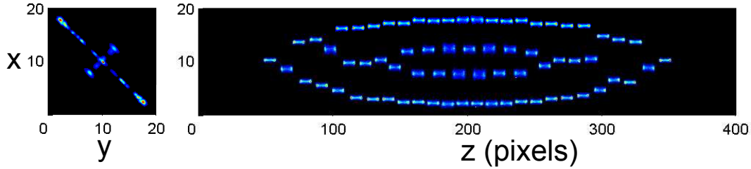
Figure 3.11 – Simulation d'image CCD d'un système de 70 ions confinés par un pseudo-potential asymétrique défini par \alpha = 4 \times 10^{-2} et a_u = 7,805 \times 10^{-3} . Les ions subissent un refroidissement Doppler par un laser dirigé selon -\hat{x} . La structure obtenue est constituée de deux zig-zag orthogonaux, disposés dans les plans (z, u) pour le plus petit et (z, v) pour le plus grand. Le mouvement du centre de masse dans la direction z produit une élongation de la tache de fluorescence dans cette direction.
