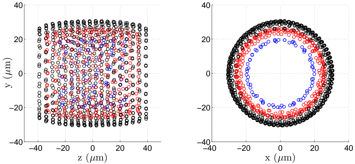
Figure 4.1 – Ensemble de 1000 ions calcium dans le pseudo-potentiel d'un octupôle linéaire. L'ensemble des ions est soumis au refroidissement Doppler, et la température atteint la limite Doppler selon chaque direction de l'espace. La structure est formée de trois tubes concentriques. Les couleurs permettent de différencier chaque tube.
