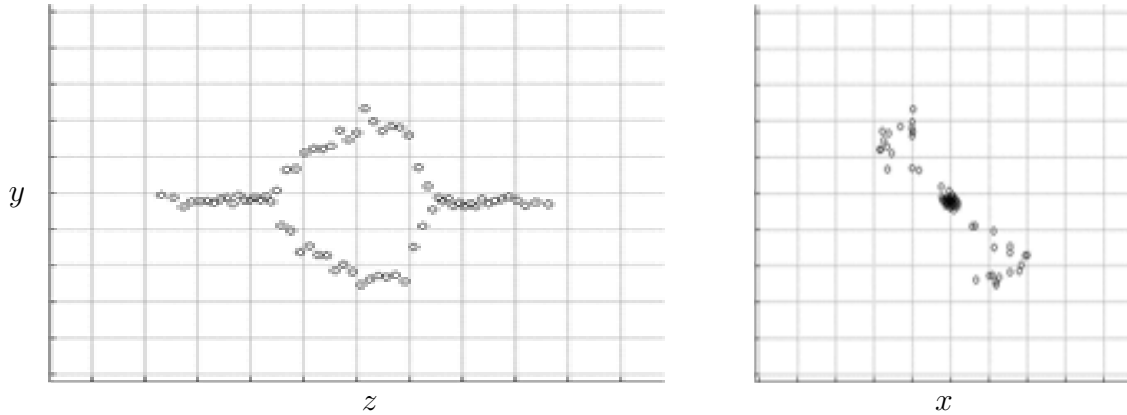
Figure 3.7 – Images de la dynamique instantanée d'un ensemble de 70 ions dans un pseudo-potentiellel défini par \alpha = 2.17 \times 10^{-3} et refroidis par un laser aligné sur l'axe x . L'image montre une zone d'étendue spatiale de 10 \mu\text{m} selon x et y , et de 1200 \mu\text{m} selon z .
