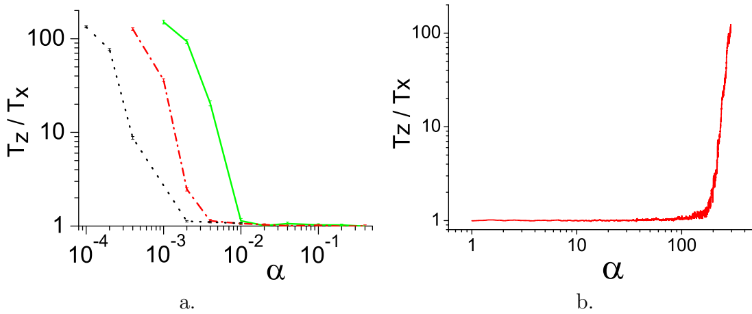
Figure 3.16 – (a) Rapport des températures T_z/T_x pour 35 ions (ligne verte), 70 ions (points-tirets rouges) et 140 ions (pointillés noirs) dans un potentiel rf anisotrope dont a_u = 7,805 \times 10^{-3} . (b) Rapport des températures T_z/T_x d'un système particulier de 70 ions obtenu en augmentant continûment \alpha au cours du temps.
