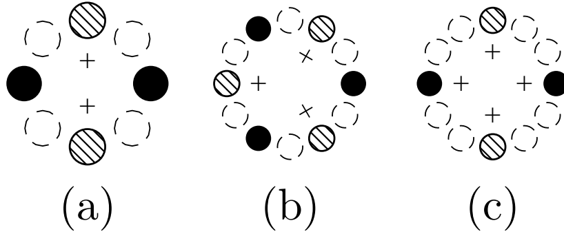
Figure 5.10 – Schéma des barreaux cylindriques de différents multipôles, pour lesquels les barreaux pleins et hachurés représentent respectivement les potentiels additionnels -V_{2p} et +V_{2p} à l'instant t = 0 . Les croix intérieures marquent les positions supplémentaires de champ rf nul d'un (a) piège octupolaire avec un potentiel quadrupolaire additionnel, (b) dodécapôle avec un potentiel hexapolaire, and (c) dodécapôle avec un potentiel quadrupolaire.
