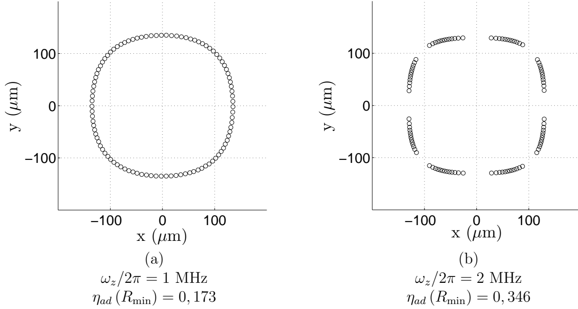
Figure 4.14 – Vue dans le plan radial de structures composées de 100 ions, obtenues dans le potentiel radio-fréquence d'un octupôle linéaire.
