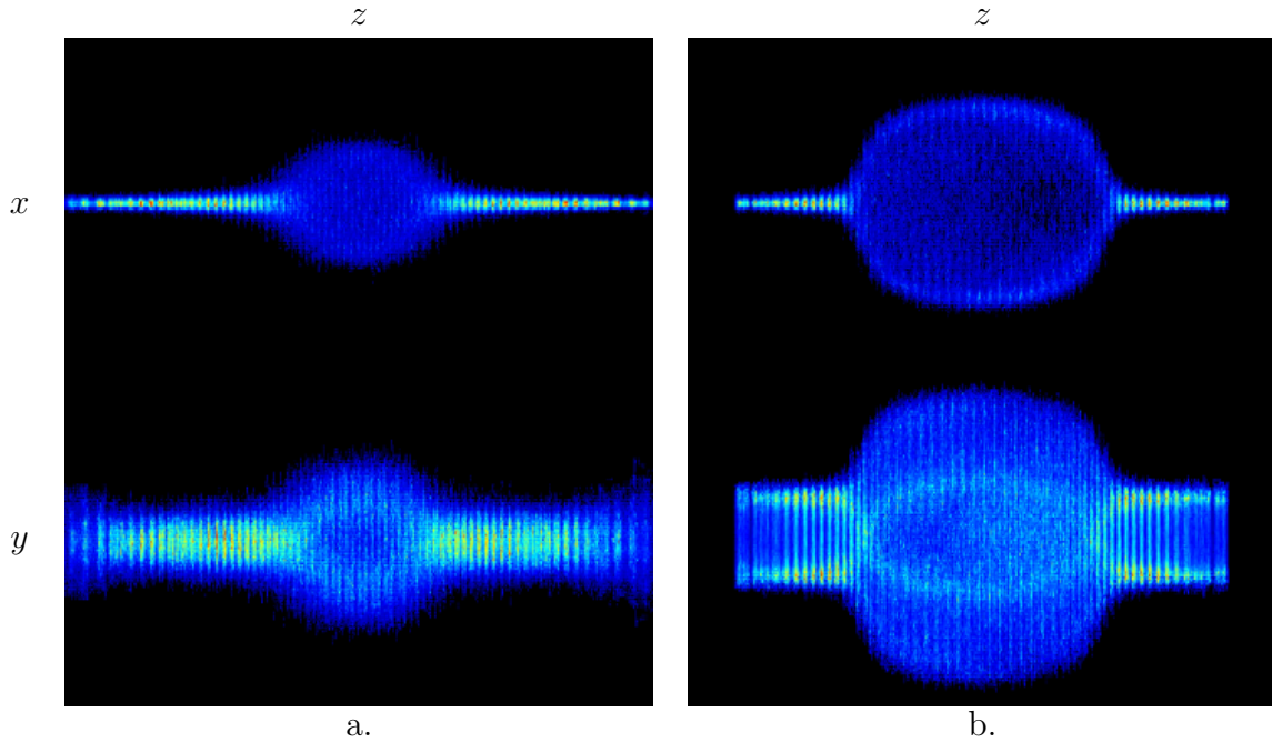
Figure 3.8 – Simulations d’images CCD d’un ensemble de 70 ions dans un pseudo-potential radial isotrope pour : (a) \alpha = 1,8 \times 10^{-3} , la longueur de la structure est \Delta z \simeq 800 \mu\text{m} et la distance maximale entre les bras du zig-zag est \Delta r \simeq 4 \mu\text{m} et (b) \alpha = 2,5 \times 10^{-3} , \Delta z \simeq 700 \mu\text{m} , \Delta r \simeq 6 \mu\text{m} . Bien qu’existent dans la direction z , le mouvement du centre de masse est uniquement visible dans le plan (y, z) du fait de la différence d’échelle.
