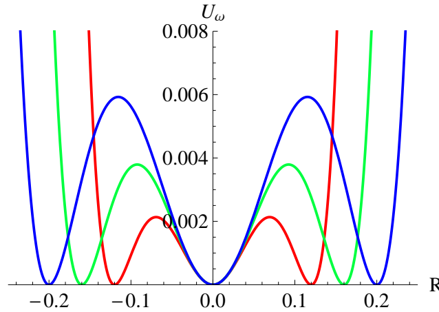
Figure 5.4 – Pseudo-potential normalisé U_\omega = \Psi / \psi_4 dans la direction \phi_{\pm 1} pour trois valeurs de \mathcal{R}_{of} . Les courbes de couleur rouge, verte et bleue correspondent respectivement à \mathcal{R}_{of} = 0,12 ; 0,16 et 0,2 .
