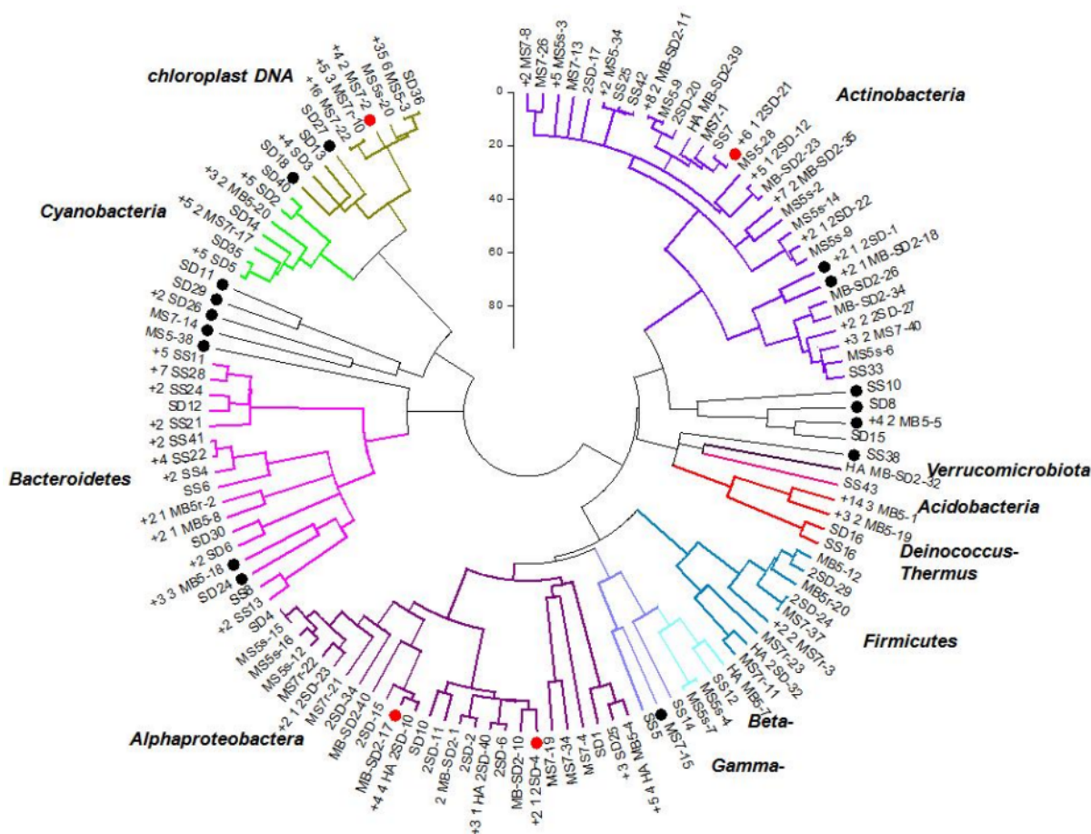
Рисунок 18. Филогенетическое дерево для 123 фило типов (без учета фило типа MS7-29 - мтДНК), выявленных в ходе настоящего исследования путем амплификации V3-V5 области гена 16S рРНК (метод Maximum Parsimony для 494 н.п., из которых 303 н.п. филогенетически информативны). Красными заполненными кругами обозначены фило типы, встреченные более чем в одной библиотеке, а черными заполненными кругами – неидентифицированные фило типы
