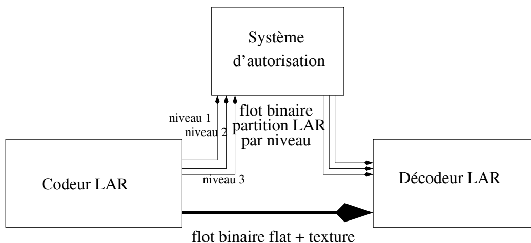
FIG. 6.1: Proposition de schéma de masquage d'image par niveaux
