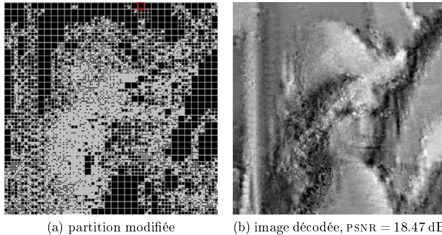
FIG. 3.6: Première étape du codage de la partition : remplacement d'un bloc 2 \times 2 , 4 \times 4 ou 8 \times 8 par un bloc 16 \times 16 aux deux tiers de la première ligne de blocs.
