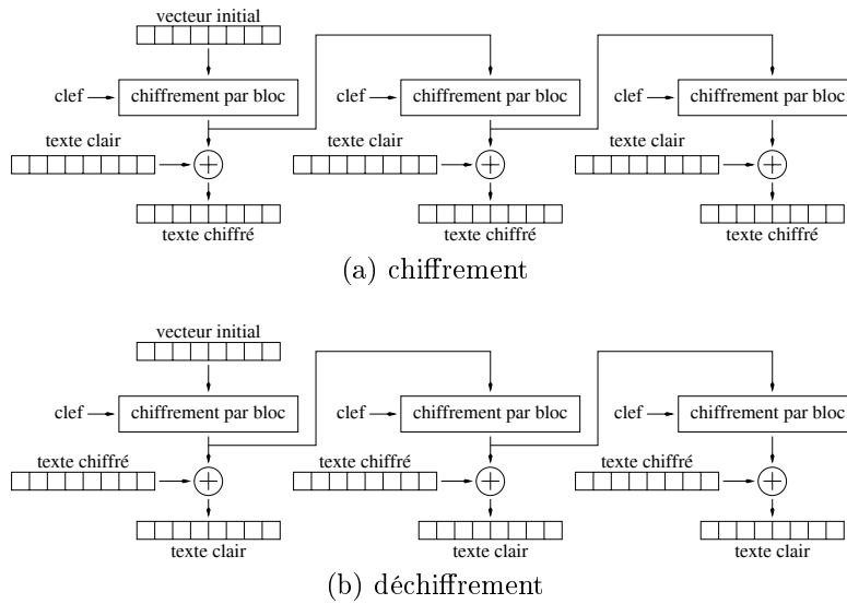
FIG. 4.7: Chiffrement et déchiffrement par bloc, mode OFB.
