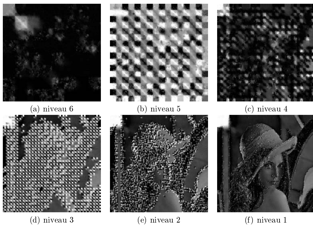
FIG. 7.12: Chiffrement RC4 combiné partition, flat et vecteur d'initialisation sur image lena pour différents niveaux
