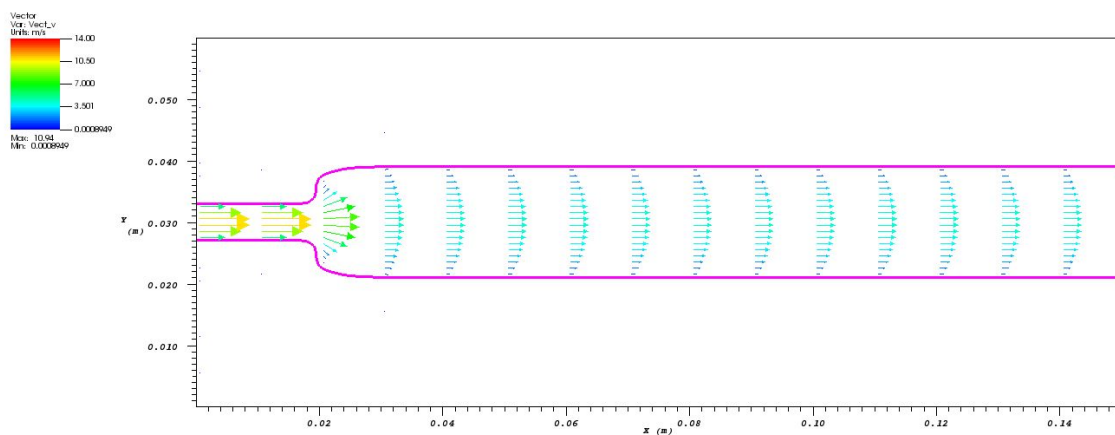
FIGURE 6.4 – Résultat 2D à t = 14225s
