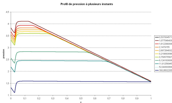
FIGURE 1.16 – Profils de pression suivant x pour k = 1
