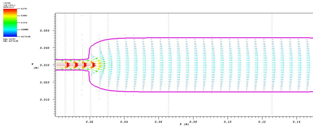
FIGURE 6.11 – Résultat 2D à t = 125749s
