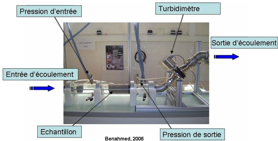
FIGURE 6.24 – Photo du banc d'essai d'érosion interne de Nadia Benahmed
