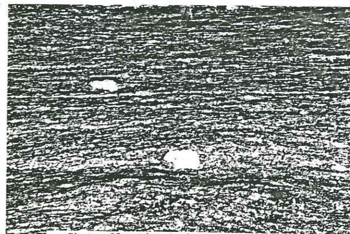
Photo. 25 : Dissolution sous pression à la base de la nappe du Mont-Joly. (nicols ouverts)
