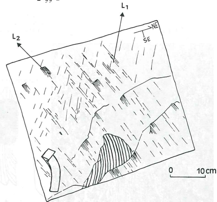
Fig. 31 : Placage de quartz fibreux indiquant une rotation antihoraire du cisaillement chevauchant, dans les mylonites de la bordure occidentale du Mont-Blanc.
