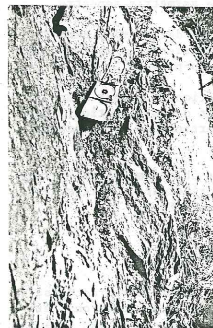
Photo. 16 : Lentille faiblement asymétrique résultant de la déformation alpine, ductile et hétérogène, des anciens gneiss métamorphiques du couloir du Bon Nant. (Sud des Aig. Rouges)
