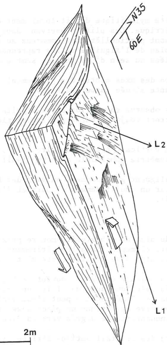
Fig . 8 : Déformations superposées de la bordure mylonitique nord-occidentale du Mont-Blanc.
