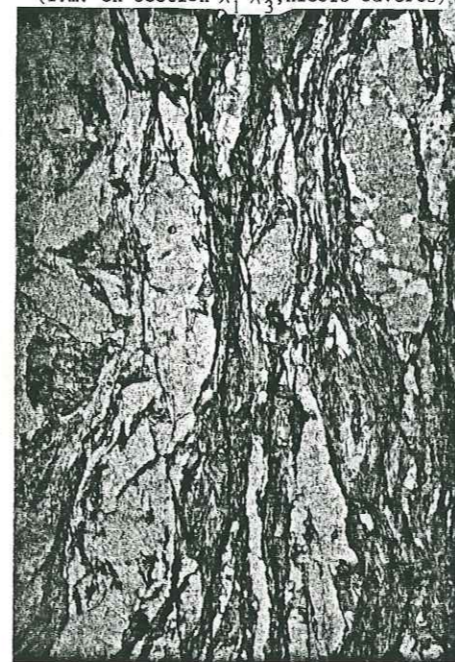
Photo. 14a : Caractère faiblement non coaxial de la déformation alpine des anciens gneiss métamorphiques du Brévent. (Aiguilles Rouges) (l.m. en section \lambda_1, \lambda_3 ; nicols ouverts)
