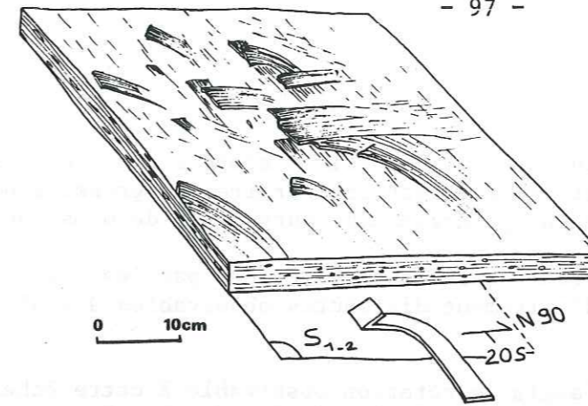
Fig. 29 : Rotation antihoraire du glissement tangentielle au toit du massif du Prarion (sud des Aiguilles rouges)
