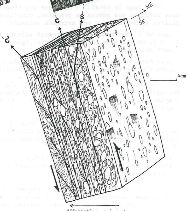
Fig. 24 : Organisation géométrique de la déformation, à l'échelle décimétrique à centimétrique, dans le granite mylonitisé du Tour. (bordure nord-occidentale du Mont-Blanc)
