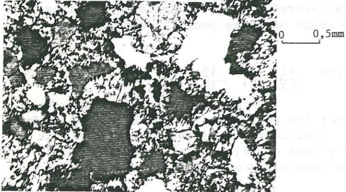
Photo. 9 : Étirement omnidirectionnel dans le plan de schistosité du Trias autochtone du sommet du massif du Prarion (Aig. Rouges) (1.m. en section λ1λ2; nicols croisés)
