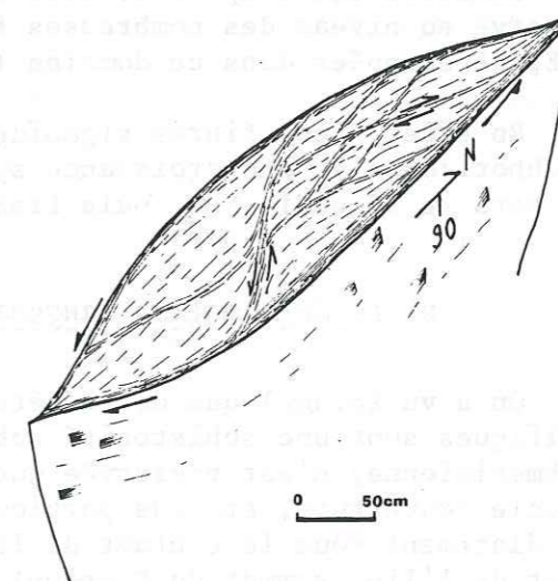
Fig. 28 : Déformation hétérogène associée au raccourcissement EW faiblement non-coaxial dans les anciens paragneiss du couloir du Bon Nant. (socle Aiguilles Rouges-Belledonne)
