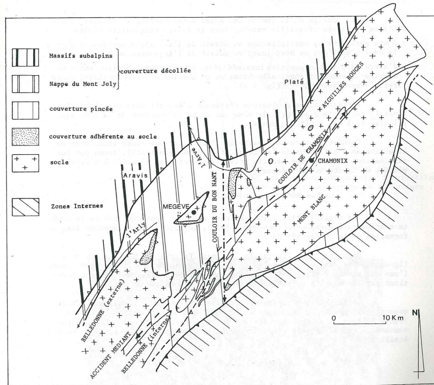
Fig. 1 b: Les grands ensembles géologiques et structuraux de la région étudiée.
