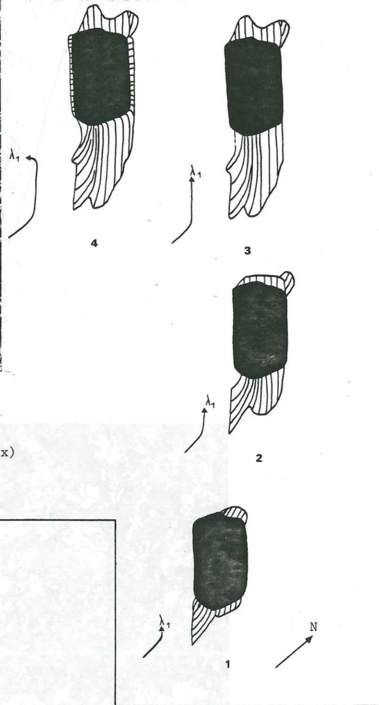
Fig . 33 : Rotation antihoraire de l'étirement principal subhorizontal \lambda_1 dans le socle Aiguilles Rouges-Belledonne. (croissance syntaxiale courbe des fibres de quartz dans les fentes de tension)
