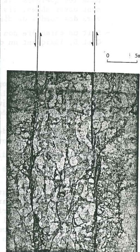
Photo. 15 : Bandes de cisaillement senestres parallèles à l'étirement minéralogique de la roche (gneiss du Brévent). (l.m. en section \lambda_1, \lambda_3 ; nicols ouverts)
