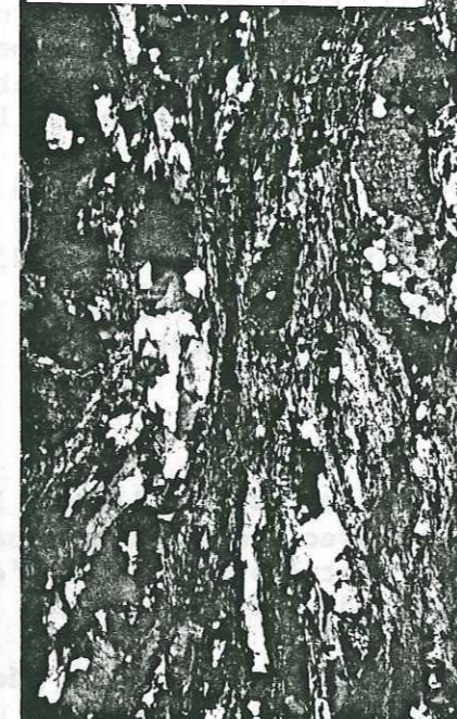
Photo. 14b : idem, nicols croisés.
