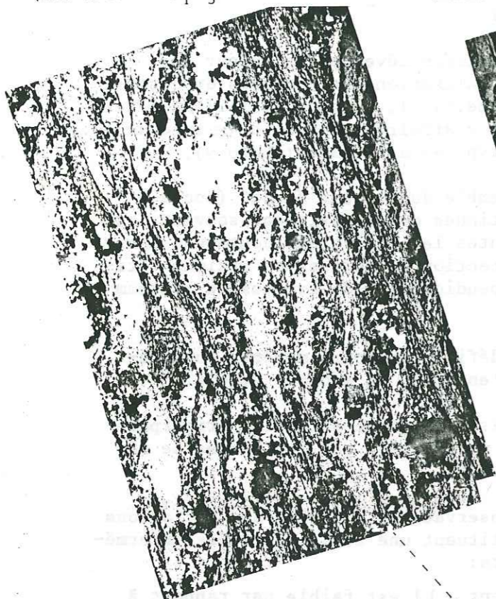
Photo. 11 : Plans (C) et (S) presque confondus + plan secondaire (C') (1.m. en section \lambda_1 \lambda_3 , nicols croisés).
