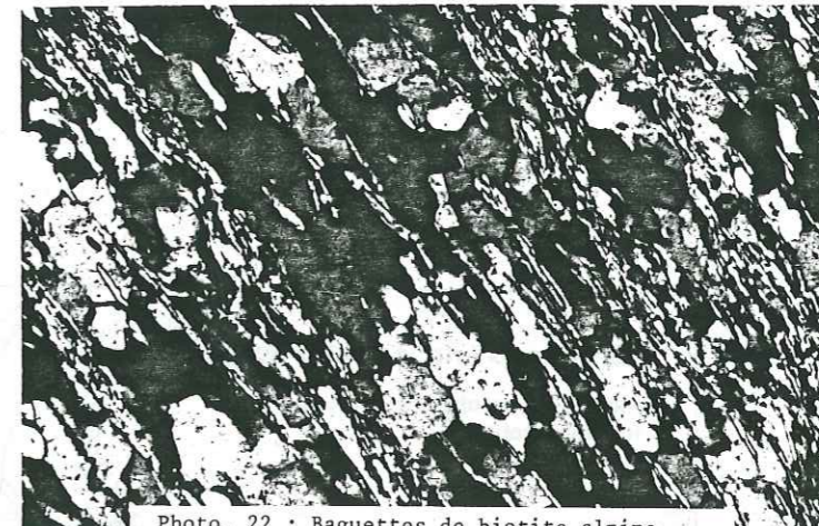
Photo. 22 : Baguettes de biotite alpine développées dans la direction de flux des ultra-mylonites de la bordure nord-occidentale du Mont-Blanc. (1.m. en section \lambda_1 \lambda_3 ; nicols croisés)
