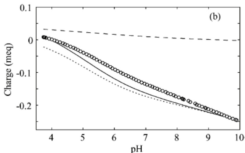
Figure 9. Charge d'une suspension d'acide humique et de goethite en fonction du pH ( I = 0.01 M KNO_3 ). Les cercles correspondent aux résultats obtenus pour le mélange ( 0.22 g HA /g goethite ), les tirets à ceux de la goethite, les pointillés à ceux de l'AH, et la ligne pleine à ceux d'un mélange sans interaction (Saito et al. 2004).
