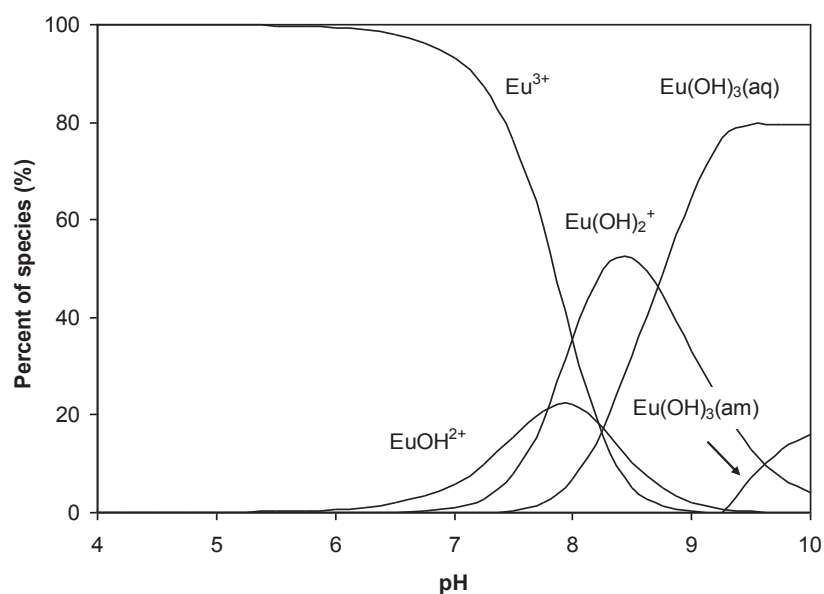
Figure 12. Spéciation de l'Euporium en solution en fonction du pH, dans le cas d'une absence de carbonates. [Eu(III)] = 10^{-6} mol/L, I = 0.1 mol/L NaClO_4 . Calcul à partir des données de Hummel et al. (2002).
