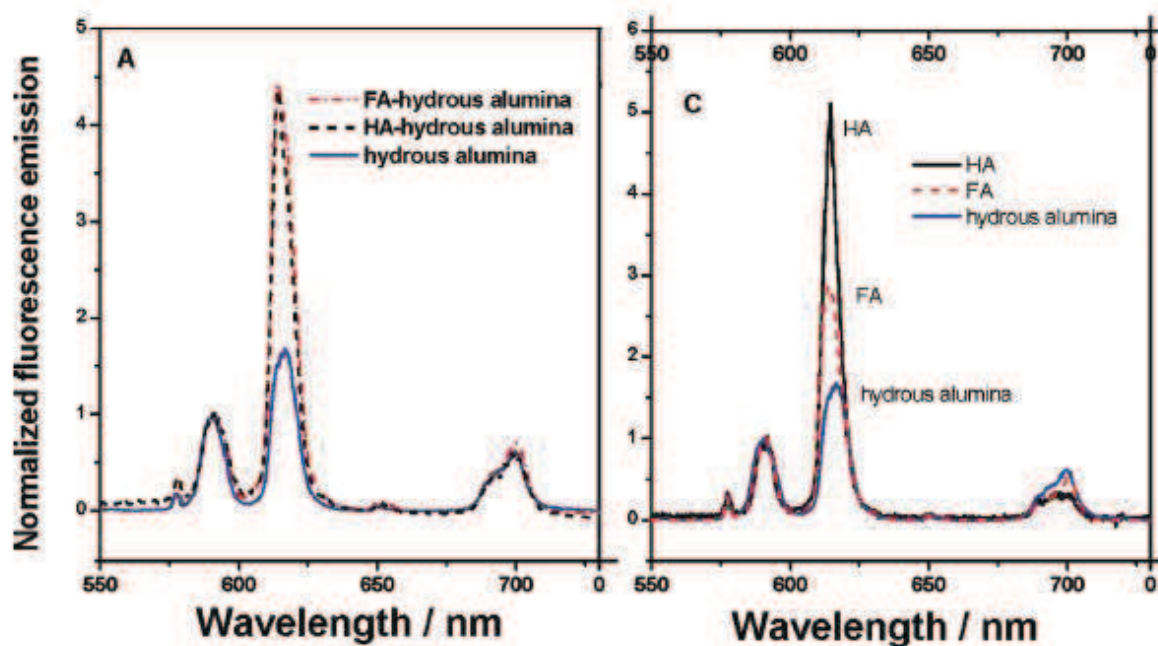
Figure 17. Spectre de luminescence de l'euprécium en présence d'alumine, d'acide humique ou fulvique ou dans un système ternaire à pH 6.3 (Tan et al. 2008).
