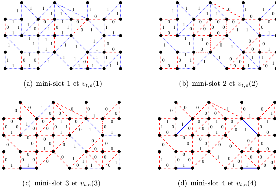
FIG. 4.6 – Mini-slots 1, 2, 3 et 4 de la sous-phase 1 d’Algorithme Log pour un graphe aléatoire avec le modèle d’interférence à distance d = 1 .
