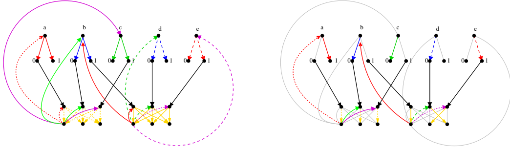
(a) Réduction de la formule (a \vee b \vee \neg c) \wedge (\neg b \vee d \vee \neg e) .
