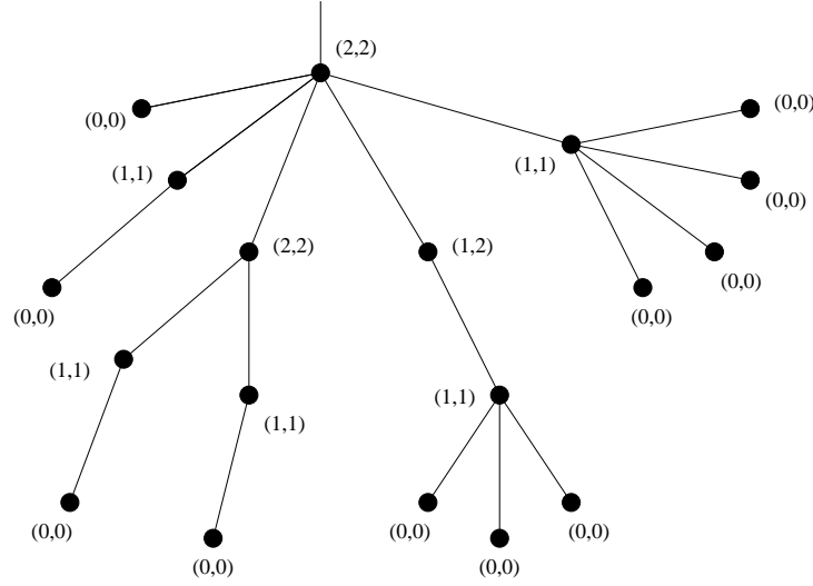
FIG. 2.8 – Exemples de différents cas d’initialisation pour le calcul de l’indice de traitement. Les paires sur les sommets représentent les entiers (p, p') correspondant aux différents sous-arbres.
