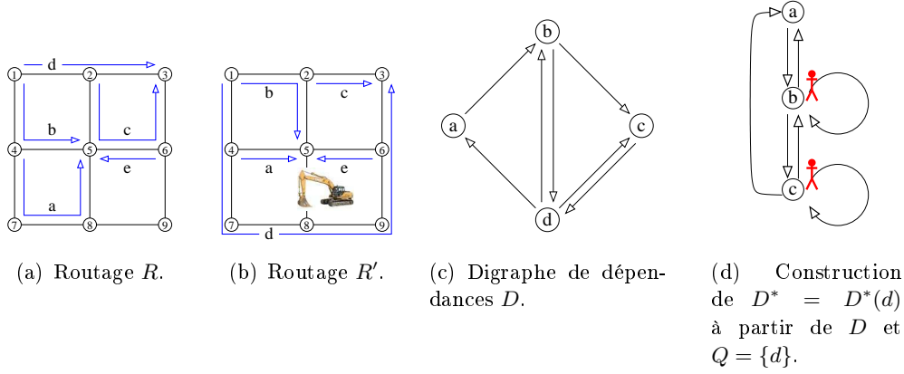
FIG. 2.16 – Le réseau est une grille 3 \times 3 avec des liens symétriques de capacité 1 (c'est-à-dire composé d'une longueur d'onde). Les figures 2.16(a) et 2.16(b) représentent le routage courant R et le routage final R' pour l'ensemble de connexions \{a, b, c, d, e\} , respectivement. L'ensemble des requêtes prioritaires est Q = \{d\} . La figure 2.16(c) est le digraphe de dépendances associé et la figure 2.16(d) représente D^* = D^*(v) construit à partir de D (Définition 24).
