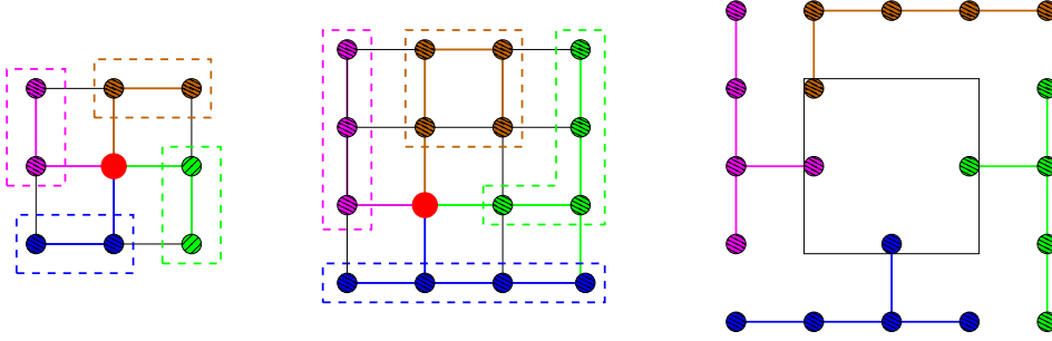
FIG. 3.11 – Partition de la grille en 4 sous-ensembles connexes de tailles presque identiques. Gauche : grille 3 \times 3 . Milieu : grille 4 \times 4 . Droite : induction de la preuve du Lemme 20.
