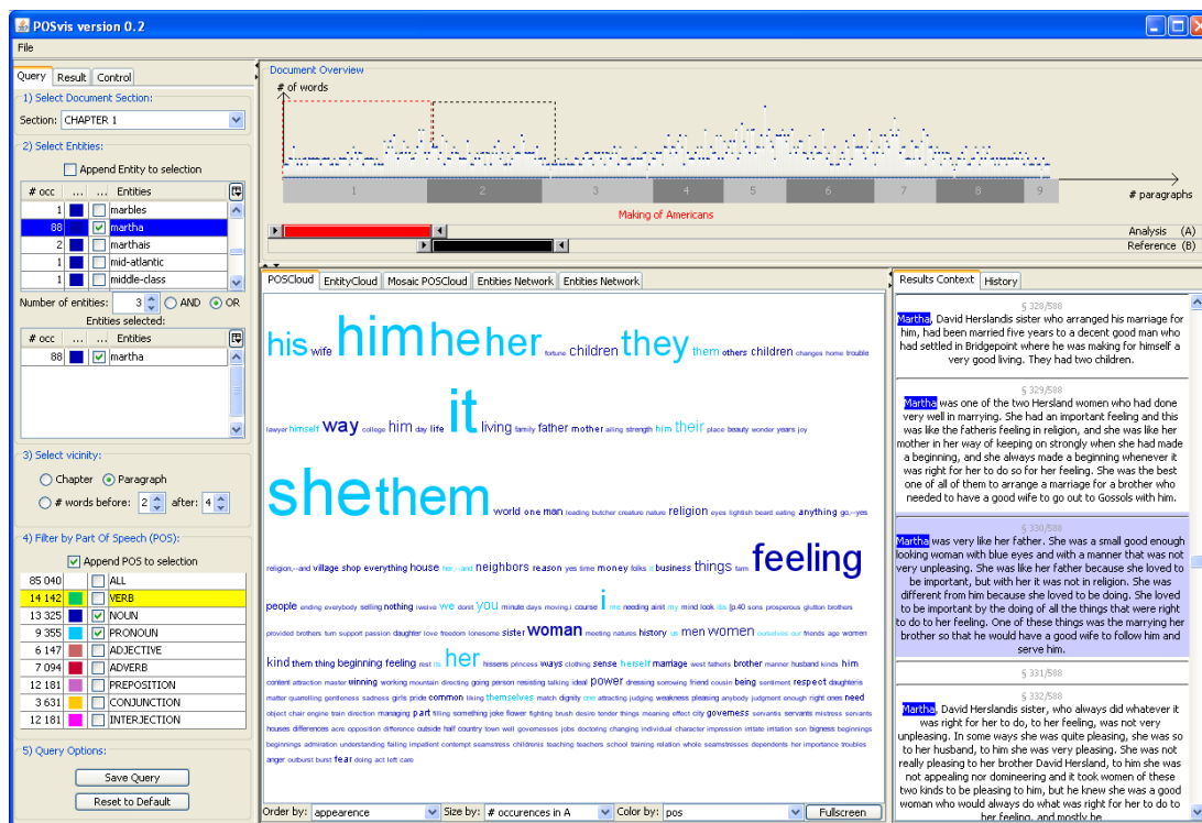
FIGURE 6.14 – Capture d'écran de l'interface principale de POSvis.
