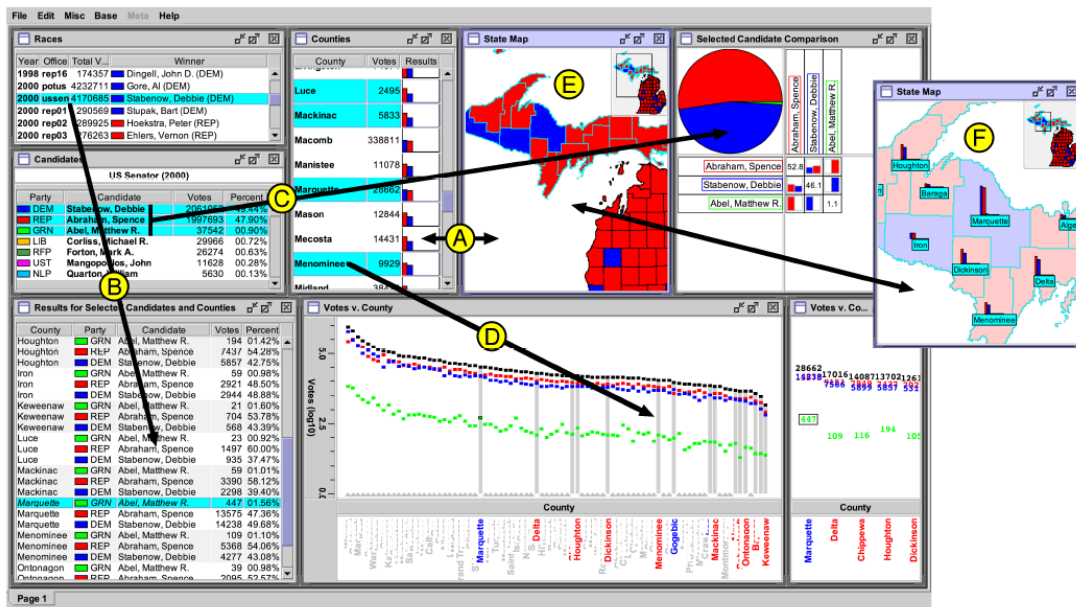
FIGURE 3.8 – Improvise [Wea04] permet la coordination entre différents points de vue sur les données.
