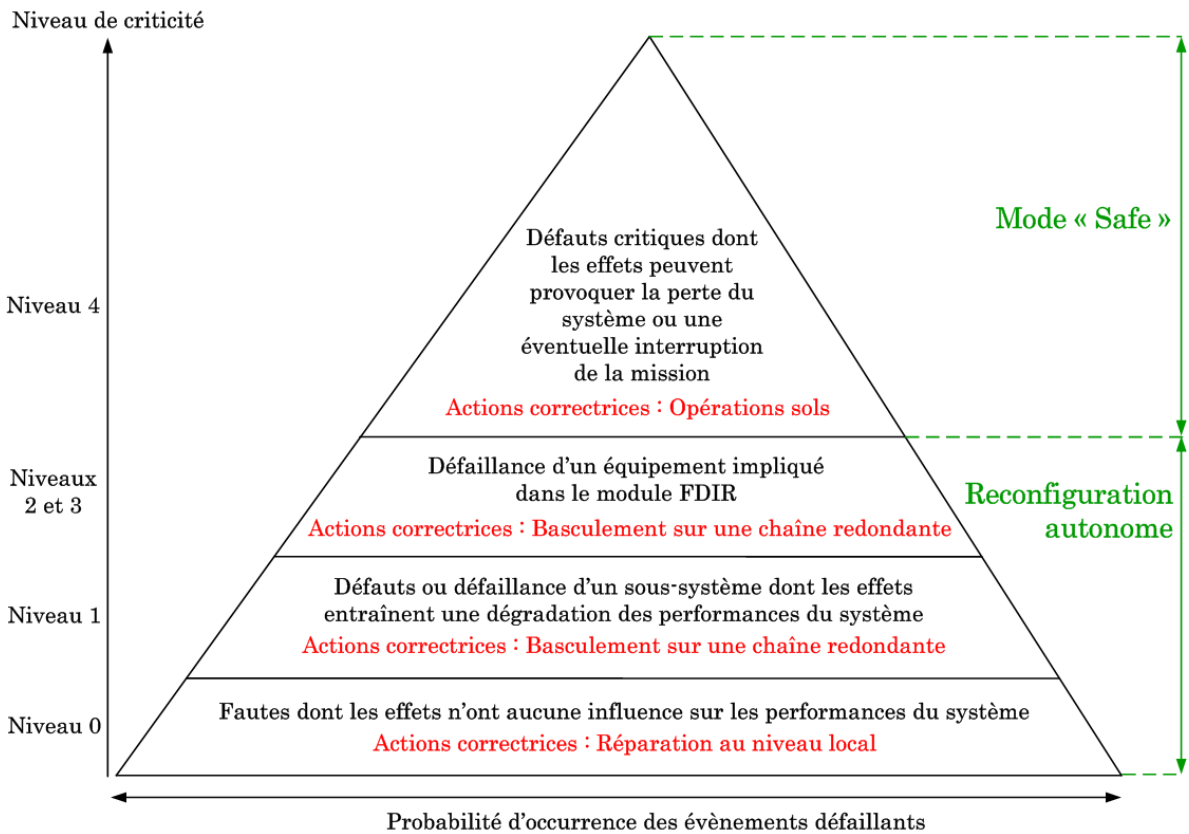
FIG. III.2 – Hiérarchisation de la stratégie FDIR
