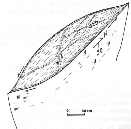
Fig. 28 : Déformation hétérogène associée au raccourcissement EW faiblement non-coaxial dans les anciens paragneiss du couloir du Bon Nant. (socle Aiguilles Rouges-Belledonne)
