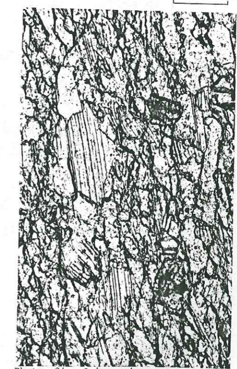
Photo. 24 : Orientation préférentielle des clivages de la calcite parallèlement à la direction de flux dans les calcaires jurassiques du col de Balme (Couloir de Chamonix) (1.m. en section \lambda_1 \lambda_3 ; nicols ouverts)
