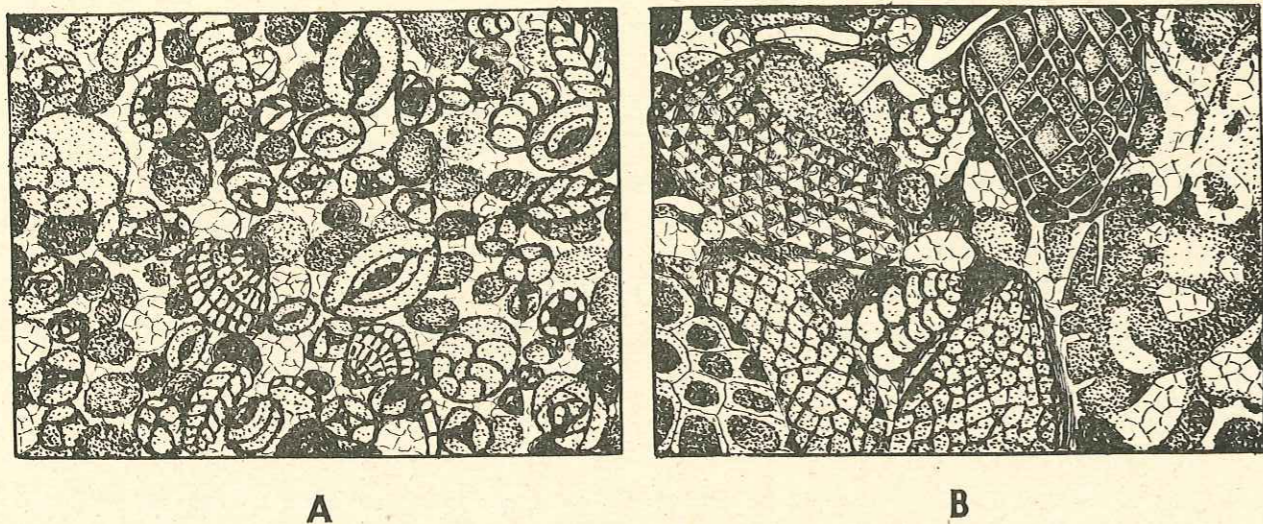
FIG. 2. — Coupes minces à travers la gangue enrobant des Spongiaires aptiens. Mas de Artis. \times 35 . A : Gangue avec sections de Miliolae. — B : Gangue avec sections d'Orbitolines.
