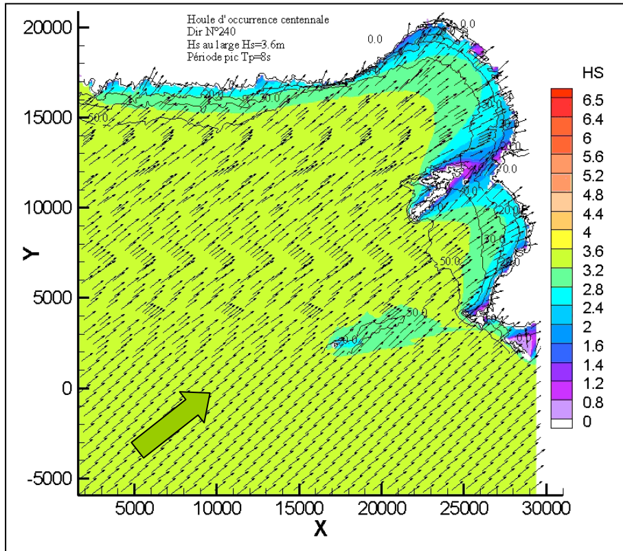
FIG IV.16 – Hauteurs significatives des vagues dans la rade de Marseille réalisée avec SWAN, pour une houle de N240° d'occurrence centennale ( H_s=3.6m et T_p=8s )
