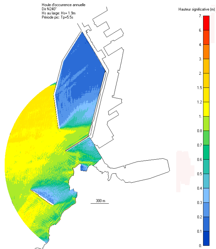
FIG IV.31 – Planche d'agitation pour la houle annuelle de N240° ( H_s=1.9\text{m} et T_p=5.5\text{s} )
