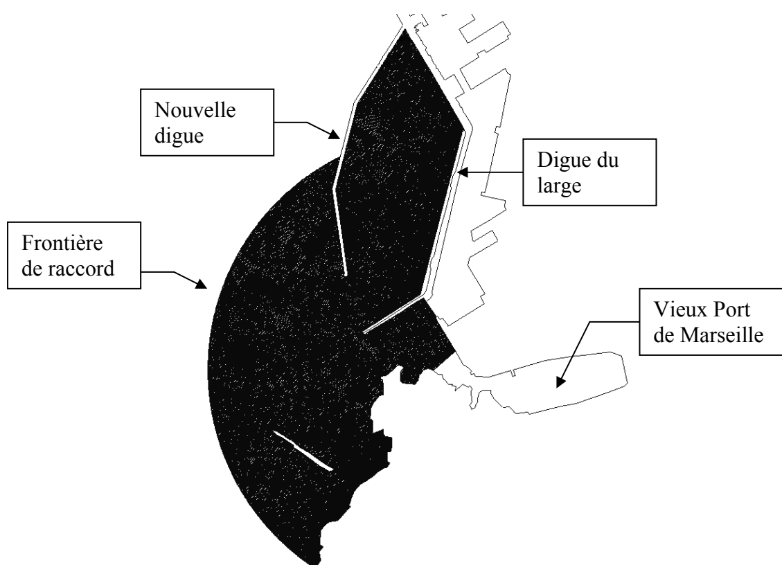
FIG IV.29 – Maillage du modèle d'agitation utilisé pour l'étude de la création d'un nouveau bassin portuaire dans le port de Marseille
