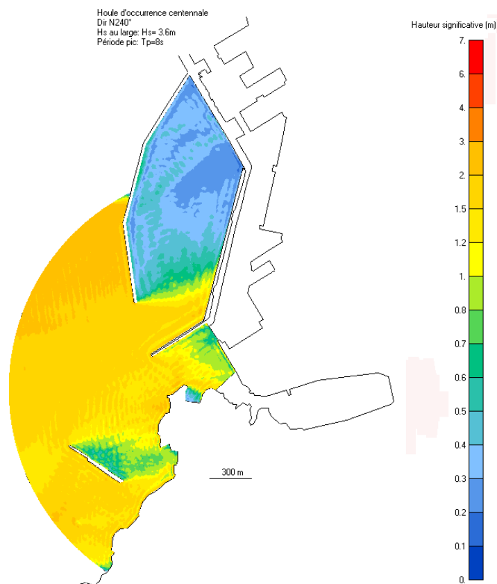
FIG IV.32 – Planche d'agitation pour la houle centennale de N240° ( H_s=3.6\text{m} et T_p=8\text{s} )
