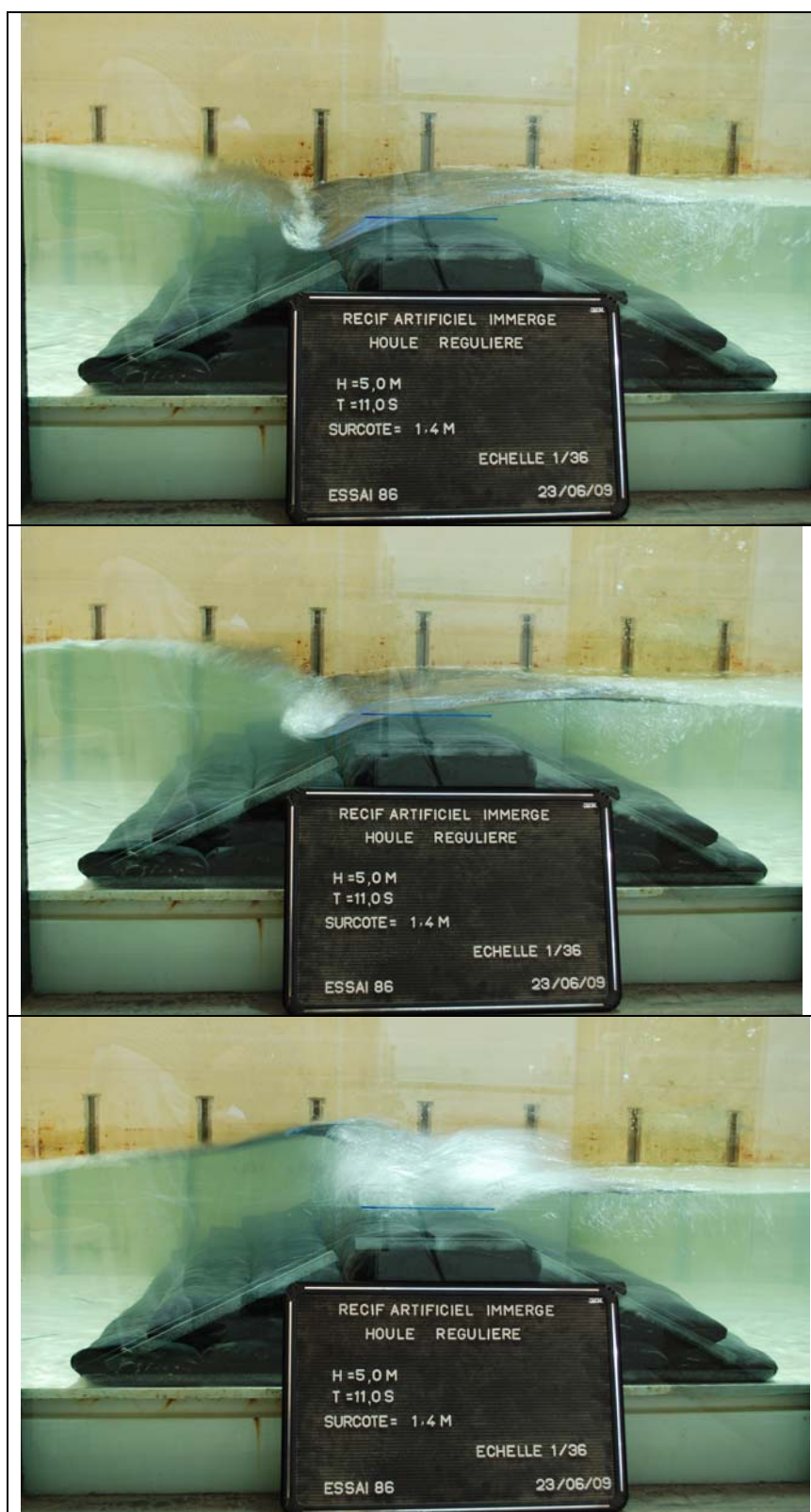
FIG VI.23 – Vue en décomposition du déferlement au dessus du récif pour une hauteur H=5m , une période T=11s et une surcote de +1.4m NGF
