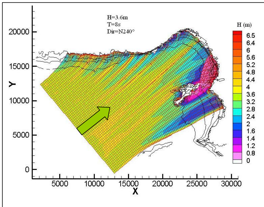
FIG IV.17 – Plan de vagues réalisé avec SIMAC-POSEIDON pour une houle monochromatique de N240°, H=3.6m et T=8s
