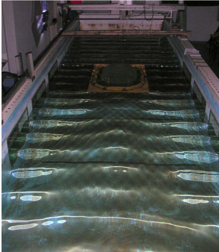
FIG III.19– Photographie de la surface libre pour le run 19
