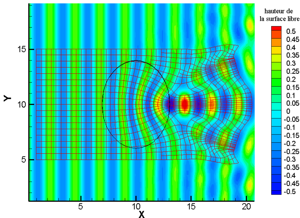
FIG IV.8 —: Superposition des plans de vagues REFDF1 et de SIMAC-POSEIDON réalisés en réfraction-diffraction, sur l'expérience de Vincent et Briggs
