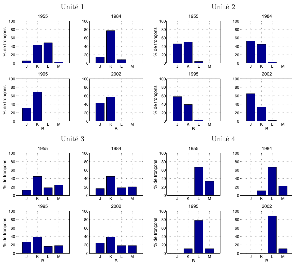
FIGURE 4.1 – Evolution dans le temps de la distribution des classes de la largeur de la bande active B en fonction des quatres unités géologiques. La définition des classes de largeur J, K, L, M est donnée dans le tableau 3.2 (la classe J correspond à la largeur la plus faible et la classe M à la largeur la plus grande).
