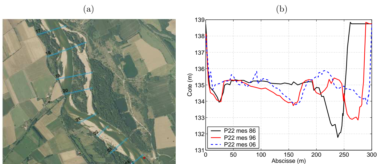
FIGURE 4.13 – (a) Localisation des profils en travers sur une photographie aérienne de 2005 et (b) évolutions du profil P22 (PK 531,1) entre 1986, 1996 et 2006.
