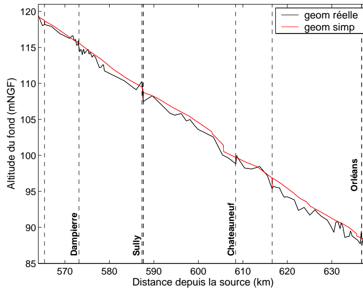
FIGURE 7.6 – Gien à Orléans : profil en long du modèle réel (basé sur les points bas des sections) et profil en long de la géométrie simplifiée. Les droites verticales en pointillées représentent les structures artificielles.
