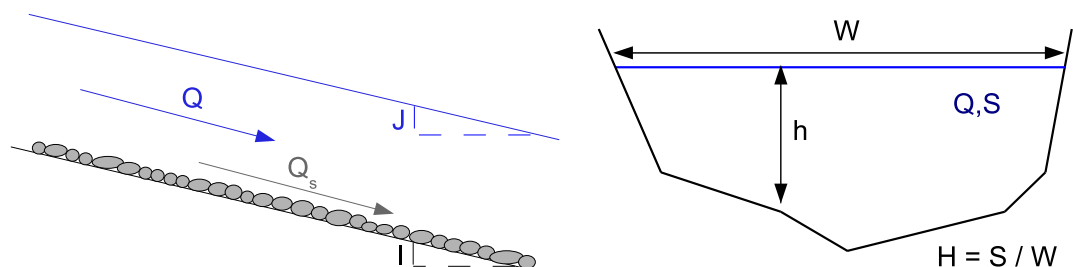
FIGURE 1.3 – Schéma des grandeurs caractéristiques des cours d'eau.
