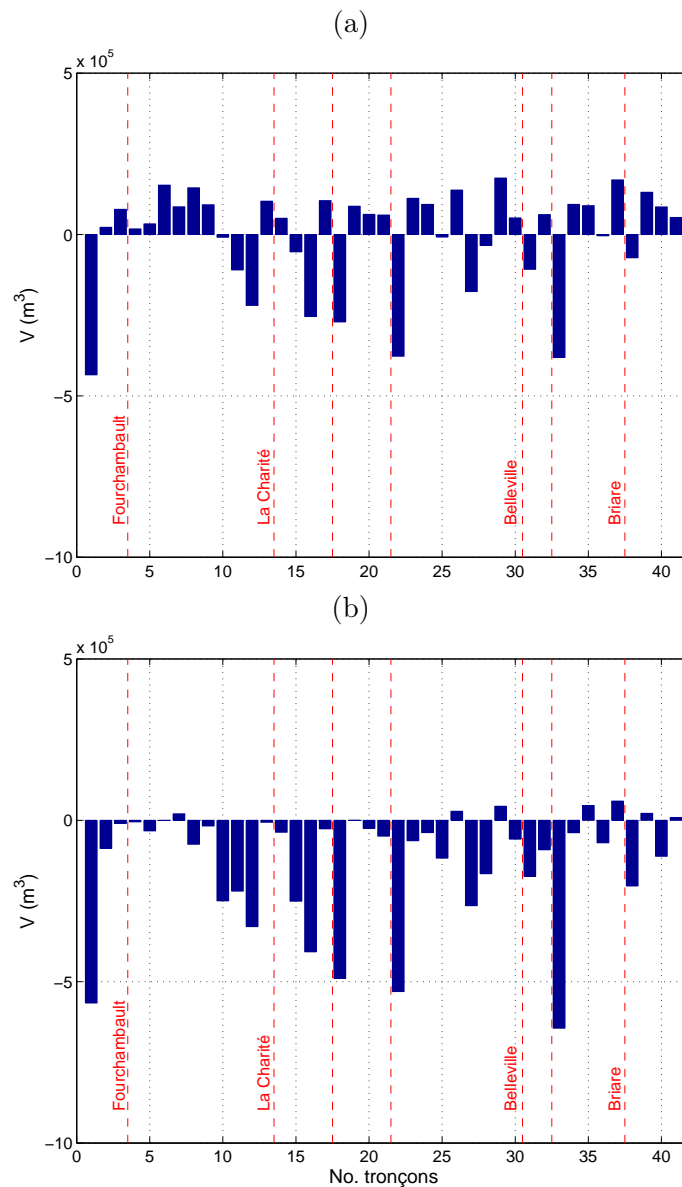
FIGURE 7.18 – Loire moyenne : bilan des volumes déposés ou érodés sur les différents tronçons localisés entre le Bec d'Allier et Gien obtenu avec (a) la chronique prédictive f1 (crués en début de chronique) et (b) la chronique prédictive f2 (crués en fin de chronique). Les droites en pointillées représentent les structures artificielles.
