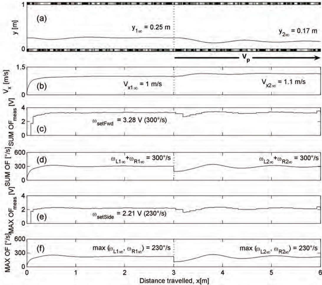
Fig. V.2.4.G. Réaction automatique à une perturbation en échelon négatif d'amplitude -115 °/s résultant de la vitesse des motifs du mur de droite V_p = +0,5 m/s. Mêmes caractéristiques de l'environnement visuel que celui de la Fig. V.2.4.D.
