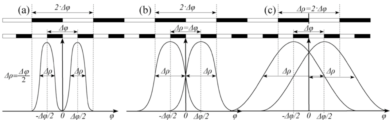
Fig. VI.2.3. Représentation de trois cas distincts de facteur de recouvrement \Delta\rho/\Delta\varphi .
