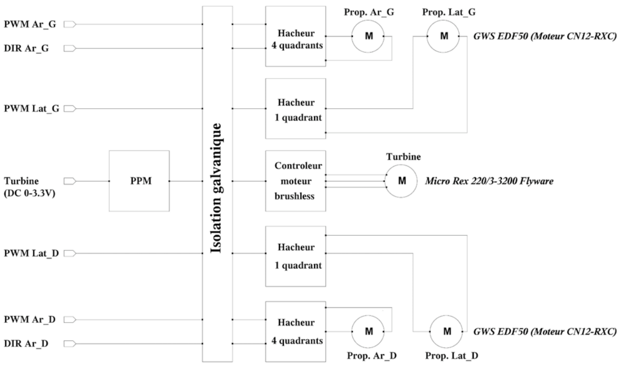
Fig. VI.4.1.3. Carte moteur distribuant l'énergie électrique aux cinq actionneurs du robot LORA.
