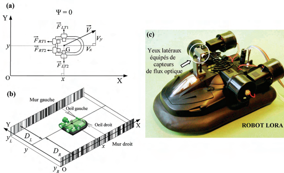
Fig. V.2.4.A. Schéma, paramétrage, et photo de l'aérogλισseur LORA (version 2 ou 3).
