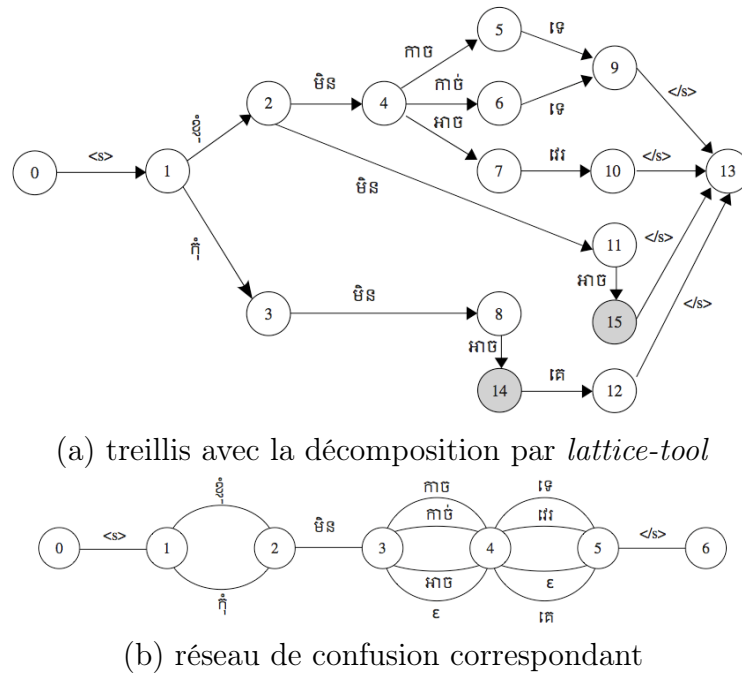
FIGURE 3.4 – Exemple de décomposition en treillis de lattice-tool
