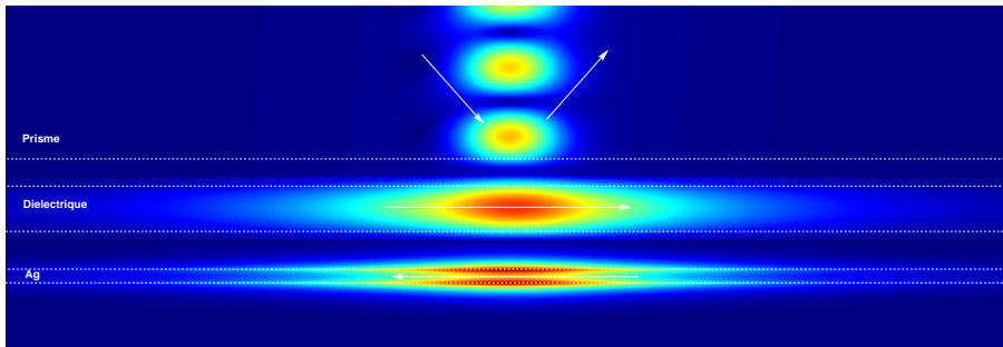
FIGURE 3.26 – Boucle de lumière excitée par couplage évanescent par un faisceau incident (angle d'incidence : 70.3^\circ , waist : 5\lambda ) dans un prisme ( \epsilon = 49 , \mu = 1 ). Le guide supérieur, constitué d'un milieu diélectrique ( \epsilon = 49 , \mu = 1 , h_1 = 0.206\lambda ), et le guide inférieur, constitué par de l'argent ( \epsilon = -4.4 , \mu = 1 , h_1 = 0.041\lambda ), sont séparés d'une distance h_1 = 0.08\lambda et entourés d'un milieu extérieur caractérisé par \epsilon = 5.5 et \mu = 1 .
