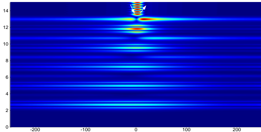
FIGURE 3.38 – Cinq boucles de lumières sont excitées dans cinq structures identiques à celle de la figure 3.34, i.e. un guide diélectrique couplé à un guide gauche, superposées et séparées par des épaisseurs de 0.6\lambda d'air. Le faisceau incident à un waist égal à 10\lambda .
