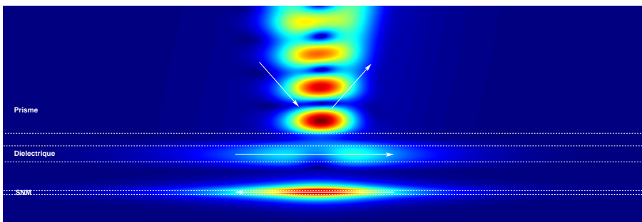
FIGURE 3.28 – Boucle de lumière excitée par couplage évanescent par un faisceau incident (angle d'incidence : 64.6^\circ , waist : 5\lambda ) dans un prisme ( \epsilon = 5 , \mu = 1 ). Le guide supérieur, constitué d'un milieu diélectrique ( \epsilon = 5 , \mu = 1 , h_1 = 0.48\lambda ), et le guide inférieur, constitué par un MEN ( \epsilon = -0.5 , \mu = 1 , h_1 = 0.057\lambda ), sont séparés d'une distance h_1 = 0.3\lambda et entourés d'un milieu extérieur caractérisé par \epsilon = 1.1 et \mu = 1 .
