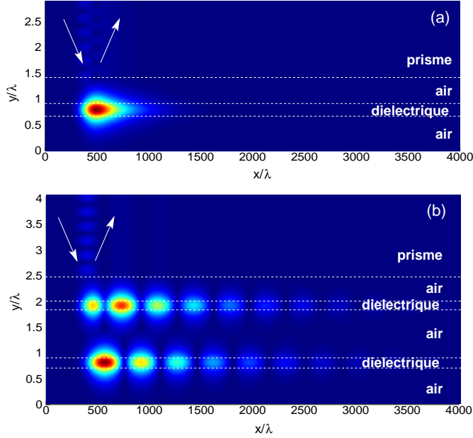
FIGURE 1.12 – Le faisceau incident (waist : 100\lambda , incidence : 36.9^\circ ) se propageant dans un prisme ( \varepsilon = 5 ) excite (a) un guide diélectrique, et (b) deux guides identiques couplés.
