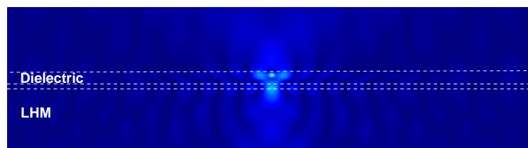
FIGURE 3.19 – Boucle de lumière excitée par une source ponctuelle située dans le guide diélectrique. La distance séparant le guide de la surface du milieu main-gauche est h_1 = 0.17\lambda .
