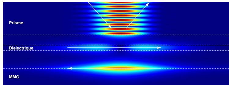
FIGURE 3.17 – Boucle de lumière excitée par un faisceau gaussien (angle d'incidence : 33.9^\circ , waist : 10\lambda ) incident dans un prisme ( \epsilon = 5 , \mu = 1 ). La distance séparant le guide de la surface du milieu main-gauche est h_1 = 0.8\lambda .
