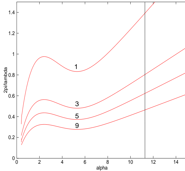
FIGURE 3.23 – Courbe de dispersion symétrique (3.27) d’un film métallique, pour différentes valeurs de \varepsilon_2 , pour |\varepsilon_1/\varepsilon_2| fixé à 0.98.
