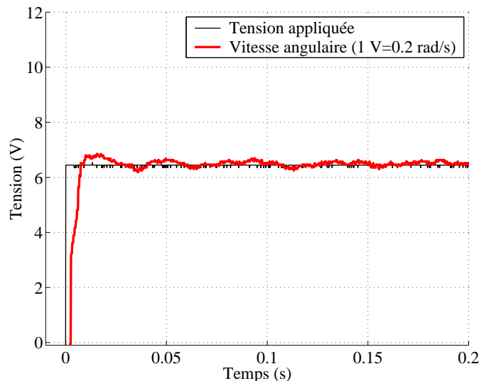
FIGURE 3.39 – Réponse à un échelon de vitesse en boucle fermée
