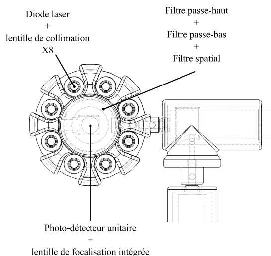
FIGURE 3.10 – Description de la tête optique
