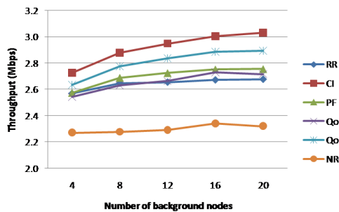
(c) Débit avec différents nombres de flux best-effort
