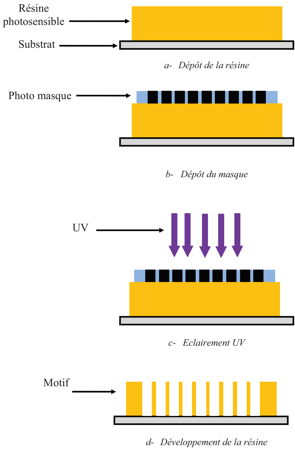
Figure II-5. Schéma de processus de lithographie optique.
