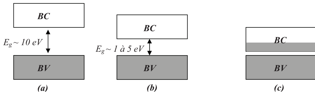
Figure IV-2. Structure de bande des matériaux isolants (a), semi-conducteurs (b) et des métaux (c).
