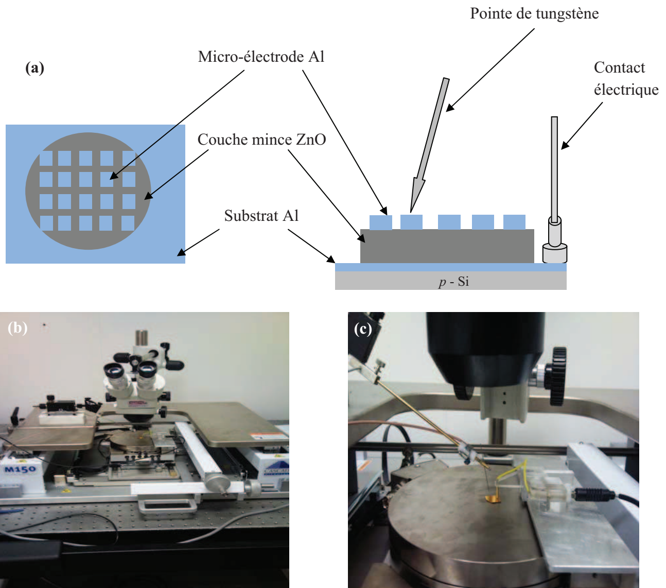
Figure IV-11. Principe de la mesure (I-V) (a). Photos du dispositif expérimental utilisé pour étude de la propriété électrique du ZnO (b) et (c).
