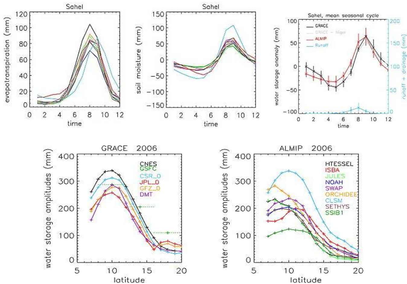
FIG. 5.2. Comparaison des simulations par neuf modèles de surface comparés dans le projet ALMIP avec les données de gravimétrie spatiale GRACE. Bande sahéenne en 2003-2007 en haut : (gauche) évaporation et humidité du sol simulées en 2003-2007 (CLSM en bleu) ; (droite) anomalie d’humidité souterraine selon GRACE et la moyenne multi-modèle. Domaine ALMIP en 2006 en bas : distribution zonale de l’amplitude des variations d’humidité souterraine selon GRACE à gauche et selon les neuf modèles de surface à droite. Source : Grippa et al. (2011) .
