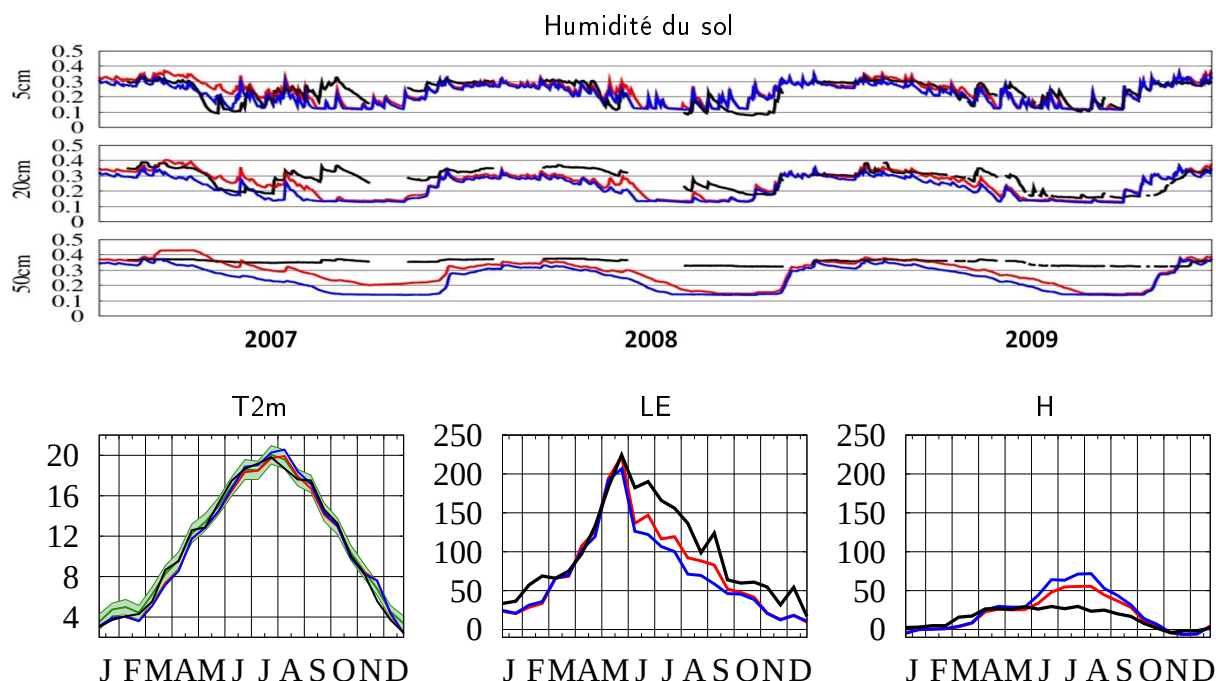
FIG. 5.4. Comparaison des simulations ORCHIDEE avec les données SIRTa 2007-2009 : (haut) Humidité du sol à trois profondeurs (en \text{m}^3 \cdot \text{m}^{-3} , les observations étant renormalisées entre les min et max des valeurs simulées sur l'ensemble de la période et du profil) ; (bas) Cycle saisonnier moyen la température de l'air à 2 m et des flux de chaleur latente et sensible. Bleu : ORCHIDEE avec F=1 ; Rouge : ORCHIDEE avec F=0 ; Noir : SIRTa ; Vert : moyenne des huit stations Météo-France dans la maille LMDz contenant le SIRTa.
