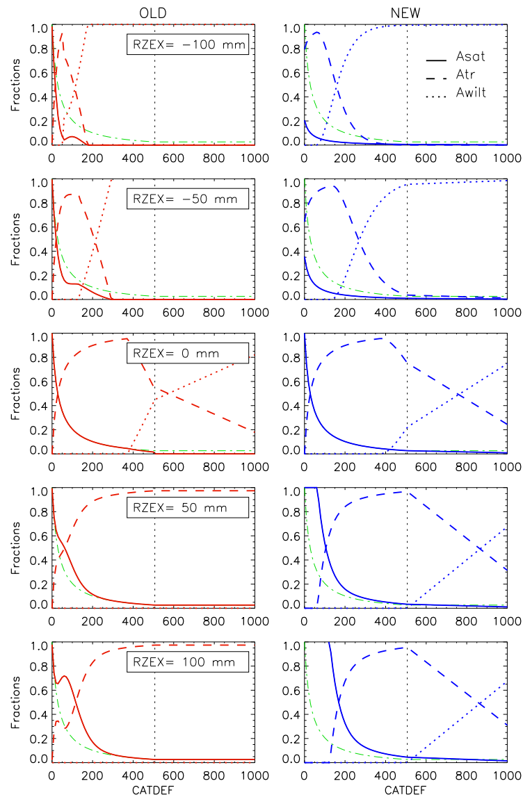
FIG. 2.4. Amélioration de la partition des BVE en trois fractions dans un BVE de la Seine. Évolution des fractions en fonction du déficit de bassin CATDEF pour cinq valeurs de M_{RZ} ( RZEX ) : paramétrisation originale de CLSM à gauche en rouge, et paramétrisation améliorée à droite en bleu. Les courbes vertes représentent les fractions saturées en situation d'équilibre (si M_{RZ}=0 mm) avec un degré de saturation au point de flétrissement \theta_w = 0.5 et une profondeur jusqu'au substratum D = 3 m, qui entraîne M_D^1 = 507 mm (ligne verticale pointillée).
