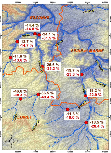
FIG. 4.14. Évolution relative du QMNA5 entre le temps présent et la fin de siècle (période 2070/2100, émissions A2) sur les principaux cours d'eau de Beauce (Loing, Essonne, Junie). Les valeurs en noir donnent l'effet direct lié à la seule diminution de la recharge des aquifères et les valeurs en rouge l'effet conjugué de la diminution de la recharge et de l'augmentation des prélèvements pour l'irrigation (à surface irriguée et assolement constant par rapport à l'actuel). D'après Ducharne et al. (2009).
