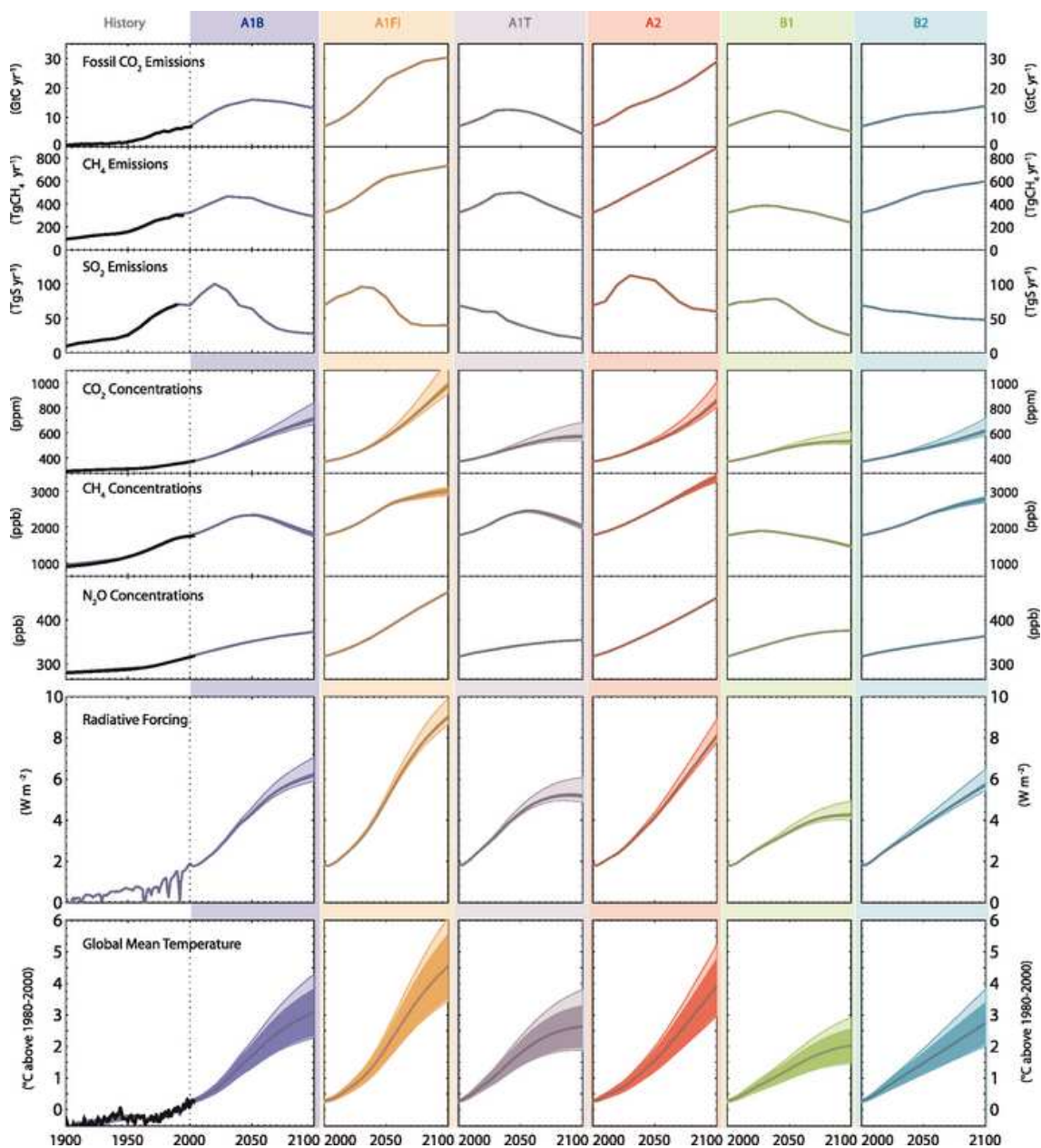
FIG. 4.1. Les six grands scénarios d'émission SRES. Du haut en bas : émissions puis concentrations en GES ( \text{CO}_2 , méthane et \text{SO}_2 ), résultantes en termes de forçage radiatif et de température moyenne du globe. Les observations sont indiquées par une ligne noire quand disponibles, pour la période historique 1900-2000. Sur les panels de température, les enveloppes colorées en foncé représentent la moyenne \pm 1 écart-type sur l'ensemble des 19 modèles climatiques considérés. L'enveloppe plus claire illustre le changement de cette marge d'incertitude si les rétroactions liées au cycle du carbone sont supposées plus faibles ou plus fortes que les hypothèses moyennes choisies. Source : IPCC (2007)
