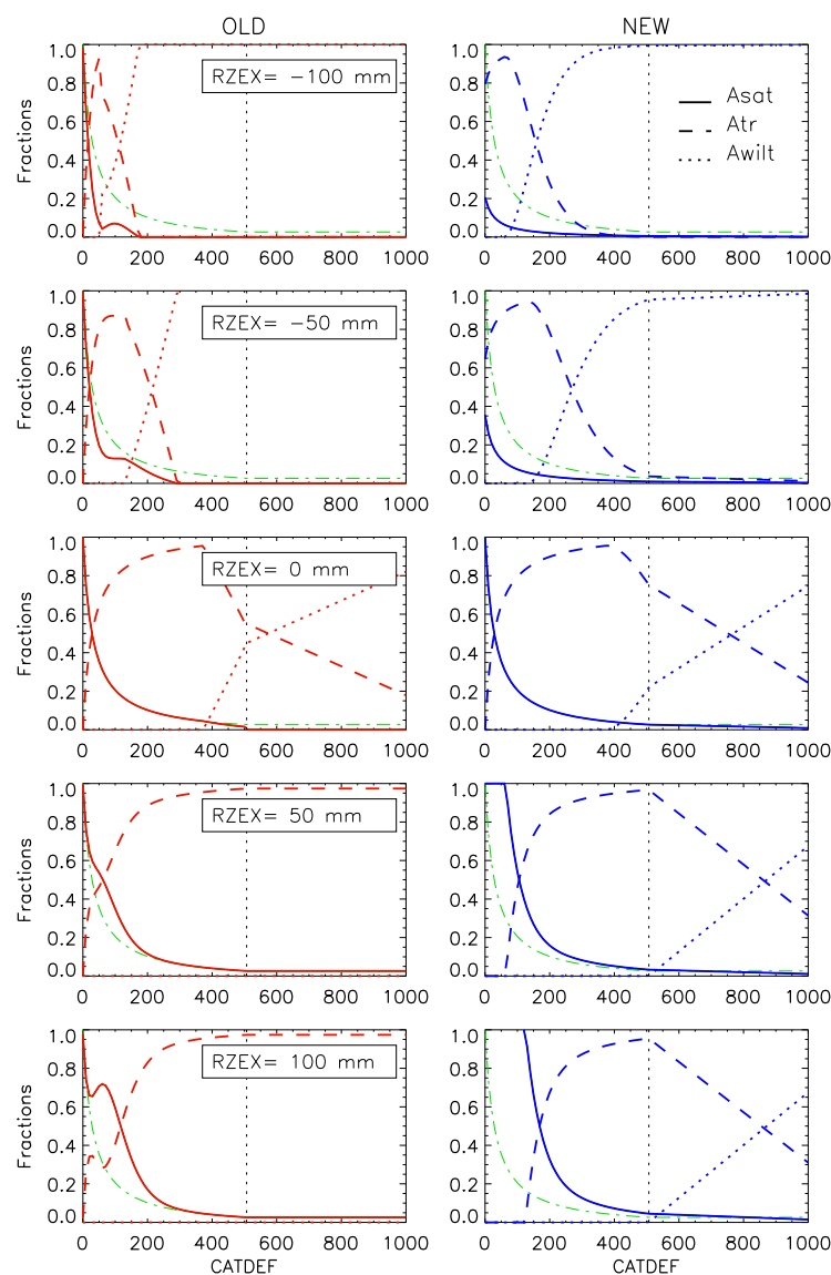
FIG. 2.4. Amélioration de la partition des BVE en trois fractions dans un BVE de la Seine. Évolution des fractions en fonction du déficit de bassin CATDEF pour cinq valeurs de M_{RZ} (RZEX) : paramétrisation originale de CLSM à gauche en rouge, et paramétrisation améliorée à droite en bleu. Les courbes vertes représentent les fractions saturées en situation d'équilibre (si M_{RZ}=0 mm) avec un degré de saturation au point de flétrissement \theta_w = 0.5 et une profondeur jusqu'au substratum D = 3\text{m} , qui entraîne M_D^1 = 507\text{mm} (ligne verticale pointillée).
