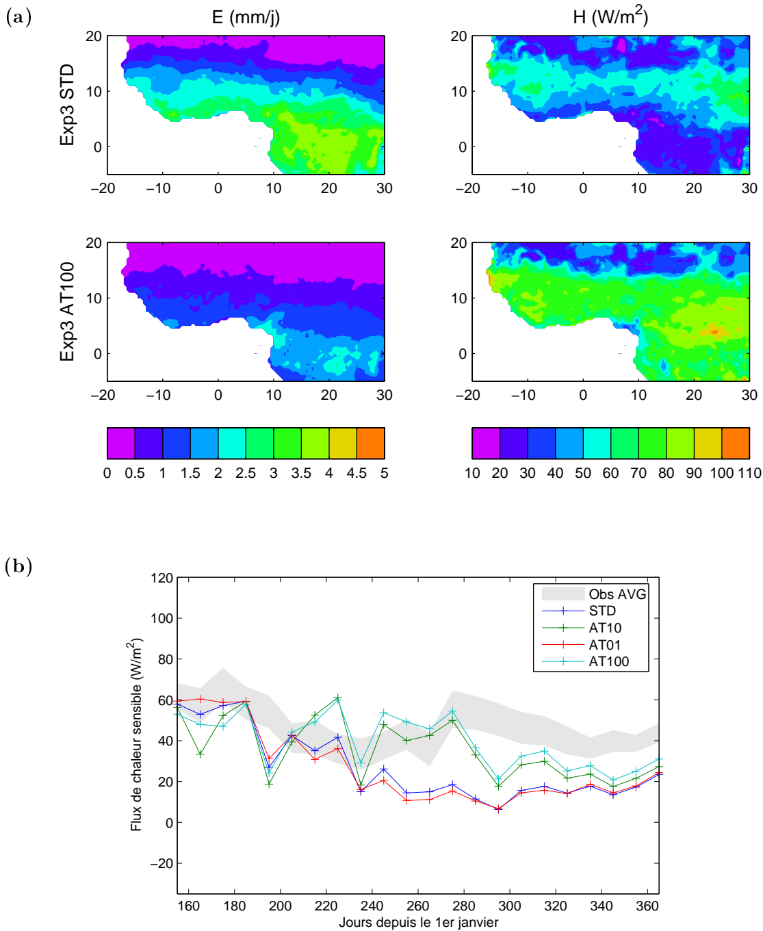
FIG. 2.9. Effet de \tau_2 sur les flux turbulents simulés en Afrique de l'Ouest, d'après Gascoïn (2009). (a) Évapotranspiration et flux de chaleur sensible dans l'ensemble du domaine ALMIP, en moyenne sur 2003-2007. Dans la simulation Exp3-STD les valeurs de \tau_2 sont les valeurs standards, alors qu'elles sont multipliées par 100 dans la simulation Exp3-AT100. Les moyennes sont calculées sur la période couvrant les années 2003 à 2007. (b) Flux de chaleur sensible journalier moyen simulé sur la période 2005-2007 dans la maille de coordonnées (1.5 °W ; 15.5 °N). Nous nous sommes limités aux 220 jours où les données de Timouk et al. (2009), représentées par la plage grise, sont disponibles sur les trois ans. La courbe bleue correspond à la simulation standard et les courbes verte, rouge, turquoise à des simulations où \tau_2 a été multiplié par 10, 0.1 et 100 respectivement.
