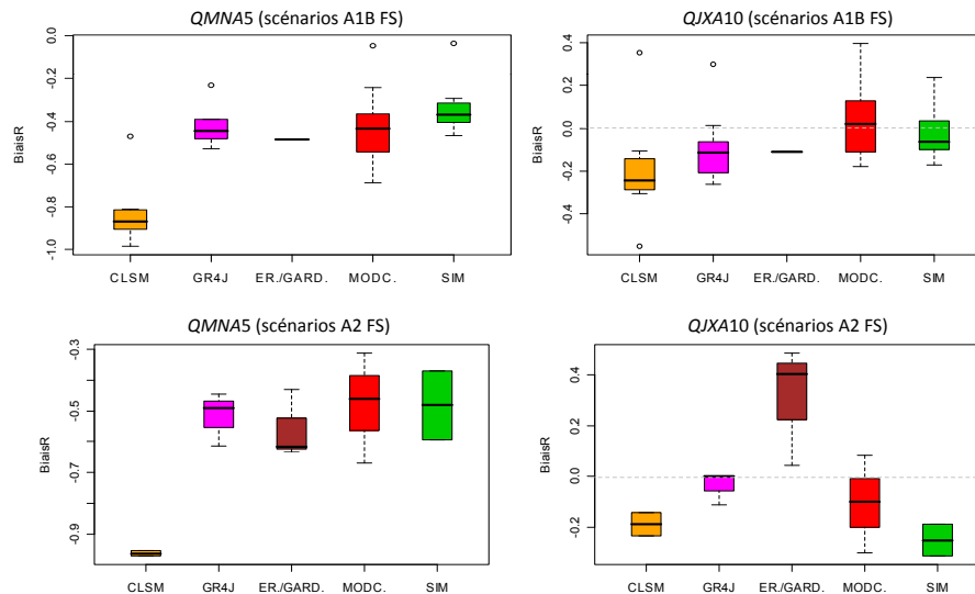
FIG. 4.12. Changements relatifs entre les QMNA5 et QJXA10 Temps Présent et Fin de Siècle dans le bassin de la Seine (valeurs dans [-1,1] ). Pour chaque modèle hydrologique, on calcule la médiane de ces changements relatifs pour chaque scénario désagrégé sur l'ensemble des stations traitées, et les boîtes à moustache représentent la distribution de cette médiane sur l'ensemble des scénarios désagrégés. D'après Sauquet et al. (2009) .
