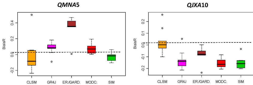
FIG. 4.6. Biases relatifs [-1,1] des quantiles de débits simulés par les différents modèles hydrologiques du projet RExHySS, sur l'ensemble des stations des bassins de la Seine et de la Somme : a) médiane des biais relatifs entre les quantiles simulés sous forçage SAFRAN et les quantiles déduits des débits observés, b) boîtes à moustaches des biais relatifs entre les quantiles simulés sous scénarios régionalisés temps présent et les quantiles simulés sous forçage SAFRAN. D'après Sauquet et al. (2009) .
