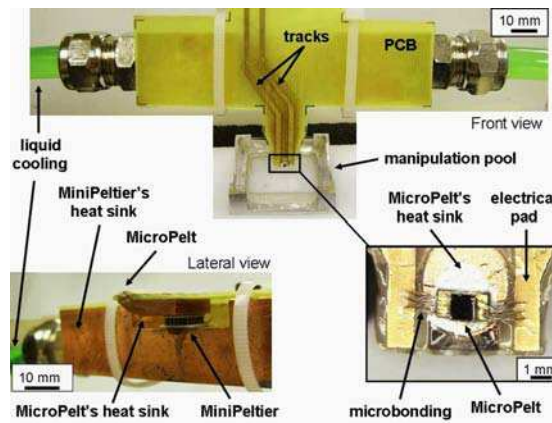
FIGURE 4.8 – Dispositif expérimental de préhension par changement de phase immergé
