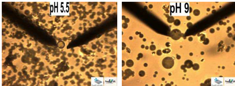
(a) Ouverture d'une pince fonctionnalisée à pH_5 : l'adhésion empêche le lâcher de la bille. (b) Ouverture d'une pince fonctionnalisée à pH_9 : la répulsion induit le lâcher de la bille qui apparaît donc floue sur l'image
