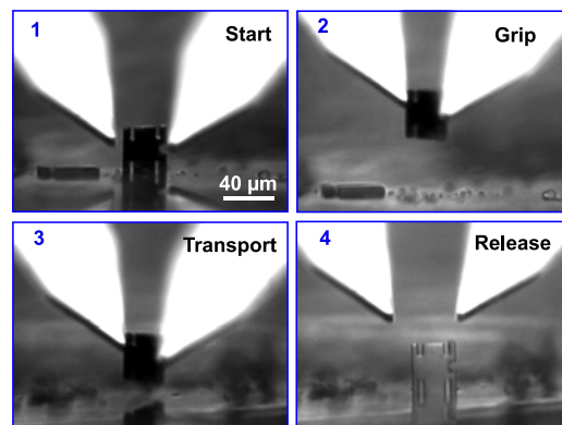
FIGURE 4.21 – Opération de prise-dépose d’un objet de taille 40 \times 40 \times 5 \mu m^3 .
