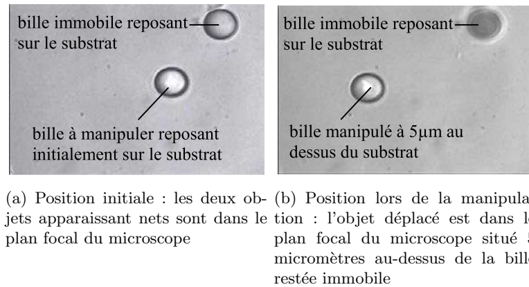
FIGURE 2.2 – Manipulation tridimensionnelle de bille de polystyrène de 7 micromètres de diamètre par laser trapping (Department of Bioengineering and Robotics, Tohoku University, Japon)
