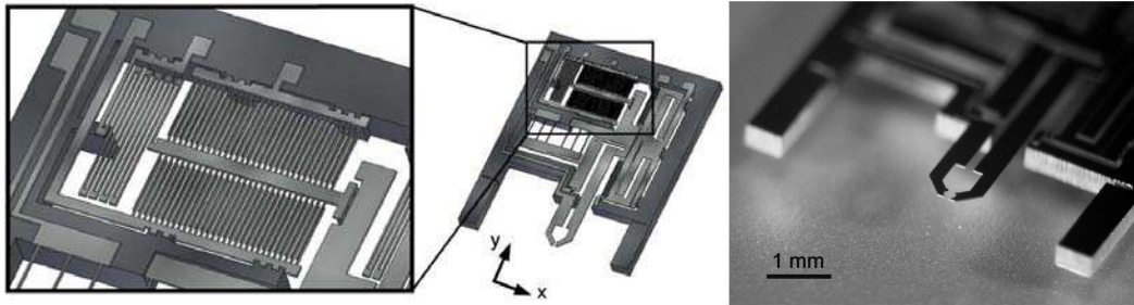
FIGURE 2.13 – Micropinche actionnée électrostatiquement et réalisée par microfabrication (LIMMS, [191]).
