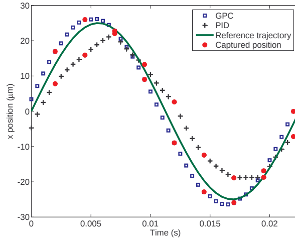
FIGURE 4.4 – Evolution de la position du micro-objet commandé par la commande GPC et un correcteur PI en réponse à une consigne sinusoïdale d’une période de 2.5\text{ms} , et d’une amplitude de 25\mu\text{m} .
