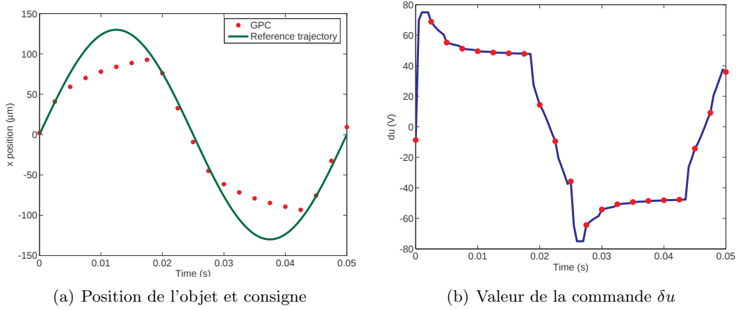
FIGURE 4.5 – Illustration du comportement du système bouclé dans la zone non linéaire : réponse à une consigne sinusoïdale d’amplitude 130 \mu m et de période 100 ms considérant une période d’échantillonnage T_c = 2,5 ms .
