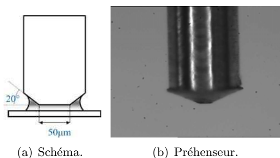
FIGURE 2.25 – Préhenseur capillaire conique tronqué de 300\ \mu\text{m} de diamètre, proposé par Schmid et al. [161] (École Polytechnique Fédérale de Lausanne, Suisse).
