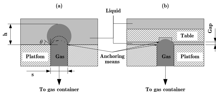
FIGURE 3.11 – Configurations types des transducteurs fluidiques capillaires
