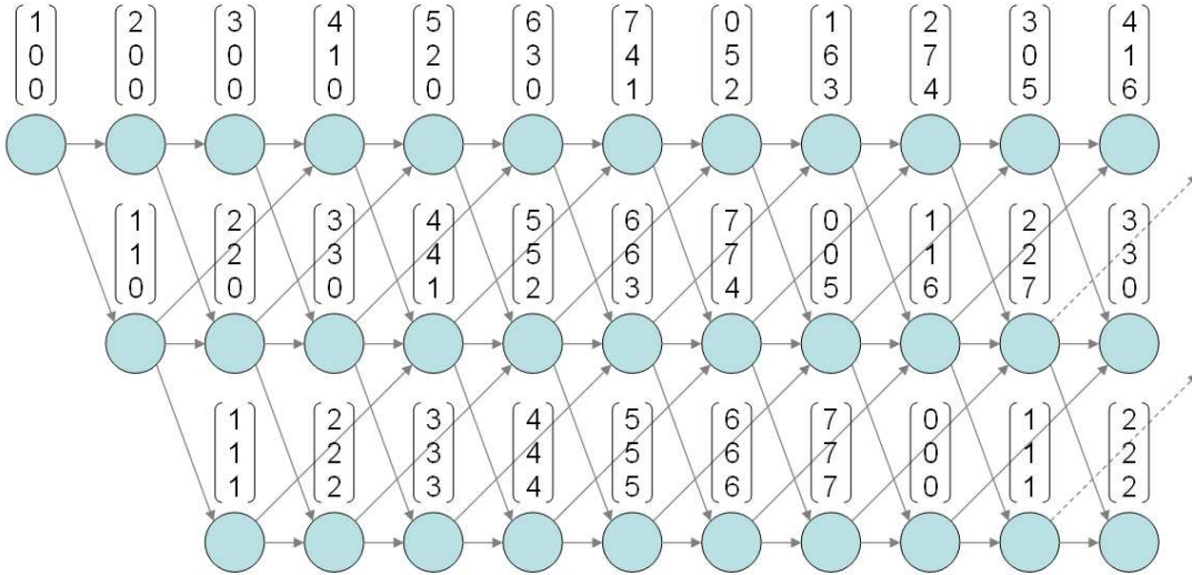
FIGURE 4.2 – Ordre partiel d'exécution et numérotation vectorielle (repliée) associée pour un pipeline à trois étages.
