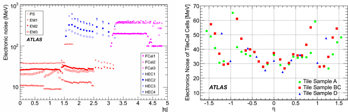
Figure 3.10 – Bruit électronique mesuré par sous-détecteur en fonction de la pseudo-rapidity \eta , pour les calorimètres à argon liquide à gauche [115], et pour le calorimètre à tuiles à droite [122]. Pour ce dernier, les compartiments A, BC, et D correspondent aux compartiments 1, 2, et 3 dans ce document (cf annexe B).
