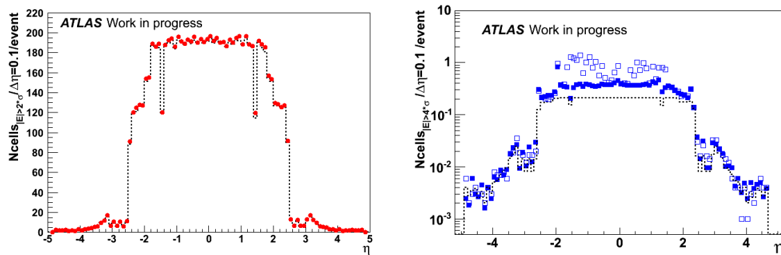
Figure 4.3 – Nombre de cellules passant la coupure |E| > n * \sigma_{bruit} , avec n = 2 (à gauche) ou 4 (à droite), normalisé à un événement de déclenchement aléatoire, par intervalle de \Delta\eta = 0.1 . La ligne pointillée représente la valeur attendue. A gauche, les points rouges représentent les données. A droite, les points bleus ouverts et fermés représentent les données avec la description du bruit dans les tuiles par une simple gaussienne et une double gaussienne respectivement.
