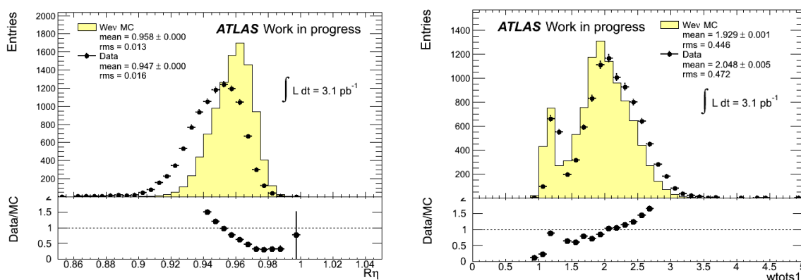
Figure 5.4 – Variables d'identification des électrons ( R_\eta à gauche et w_{tot s1} à droite) pour des électrons issus de bosons W , satisfaisant les coupures d'identification tight , sauf la variable concernée. Les points correspondent aux données, tandis que l'histogramme jaune pâle correspond à la simulation Monte-Carlo d'événements W \rightarrow e\nu .
