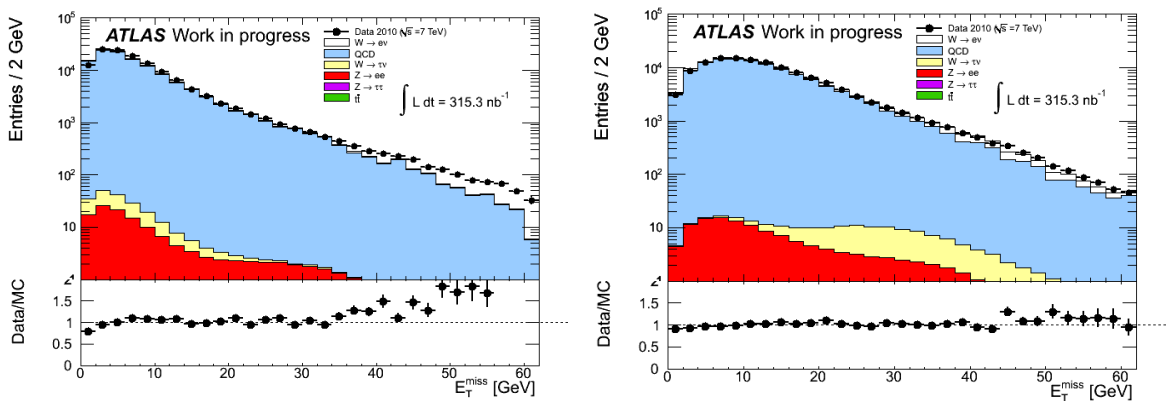
Figure 4.30 – Distributions de E_T^{miss} calculées uniquement avec les cellules du calorimètre à l'avant (à gauche), ou en enlevant les cellules du calorimètre à l'avant (à droite) [153].
