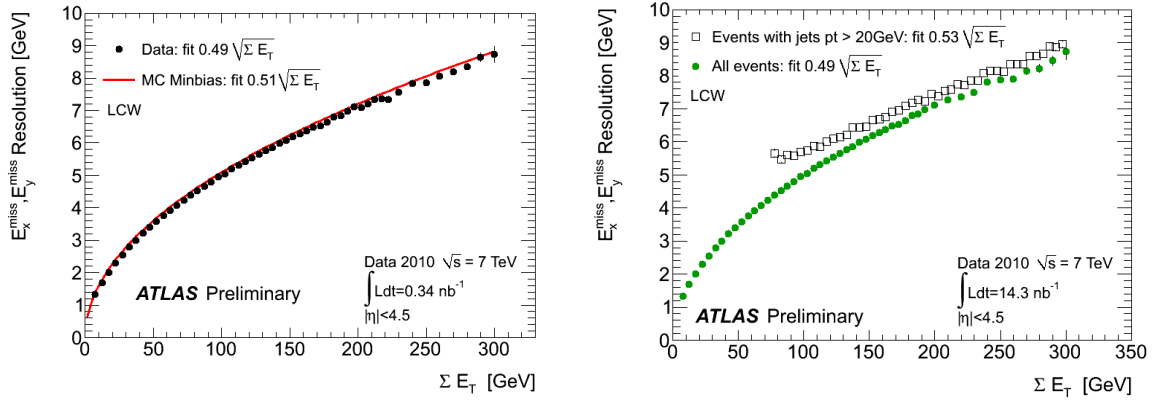
Figure 4.27 – Résolution de E_x^{miss} et E_y^{miss} calibrées en fonction de \Sigma E_T pour des événements de biais minimum, pour des collisions à 7 TeV. A gauche, les ronds noirs correspondent aux données et la ligne représente le fit de la résolution obtenu avec la simulation Monte-Carlo. A droite, les points verts représentent tous les événements de biais minimum et les carrés noirs les événements contenant au moins un jet avec p_T > 20 GeV [128].
