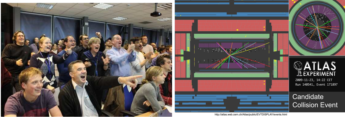
Figure 2.2 – A gauche, photo prise dans la salle de contrôle d’ATLAS au moment du retour des premiers faisceaux en 2009. A droite, affichage d’évènement d’une collision à une énergie dans le centre de masse de 900 GeV enregistrée le 23 novembre 2010 où le champ solénoïdal était éteint.
