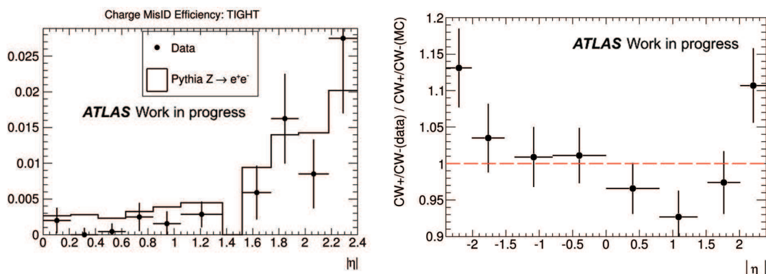
Figure 7.18 – A gauche, més-identification de la charge en fonction de la pseudo-rapacité, pour les données et la simulation. A droite, double rapport (\epsilon^+/\epsilon^-(données))/(\epsilon^+/\epsilon^-(MC)) de l'efficacité d'identification des électrons [251].
