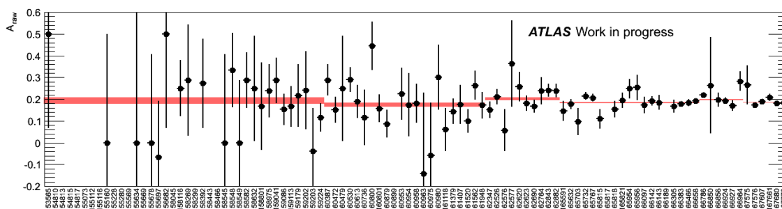
Figure 7.15 – Asymétrie de charge brute en fonction du temps, pour les périodes B à I. Chaque point correspond à un run avec son erreur statistique, et les rectangles rouges correspondent à la moyenne par période, de largeur égale à l'erreur statistique.
