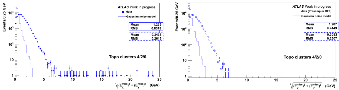
Figure 4.9 – Distribution de E_T^{miss} mesurée avec la méthode des topoclusters, avec des événements de déclenchement aléatoire du run de référence. Les points représentent les données, la ligne le jouet Monte-Carlo. A gauche, tout le système calorimétrique est considéré, à droite les cellules du pré-échantillonneur du calorimètre électromagnétique ne sont pas prises en compte.
