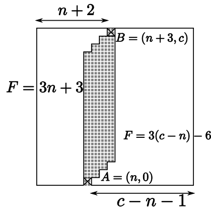
FIG. X.25. Nombre de frontières dans les bottes.
