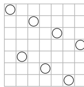
FIG. I.2. Configuration produite avec la stratégie du cavalier.
