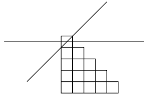
FIG. B.1. Exemple d'un convexe où 2 droites différentes engendrent la même frontière.
