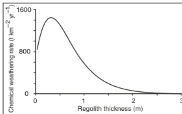
Figure I.6 : Représentation du taux d'altération chimique ( t/km^2/an ) en fonction de l'épaisseur de sol (m), d'après Gabet and Mudd (2009).
