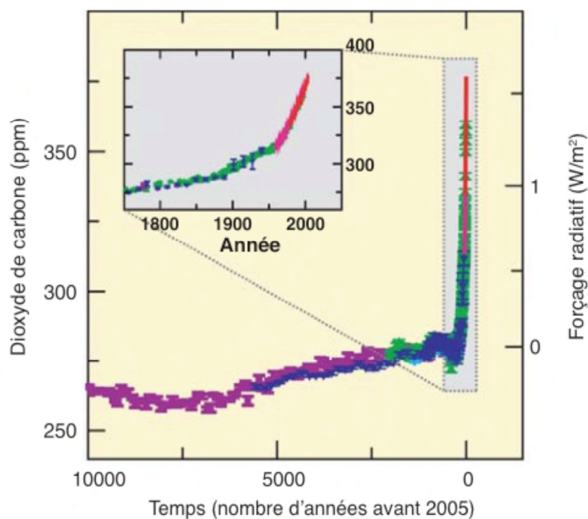
Figure I.8 : Concentration atmosphérique de CO 2 durant les 10 000 dernières années (grand graphique) et depuis 1750 (médaillon). Les mesures proviennent des carottes de glace (symboles de couleurs correspondant aux diverses études) et d'échantillons atmosphériques (lignes rouges), modifié d'après IPCC (2007).
