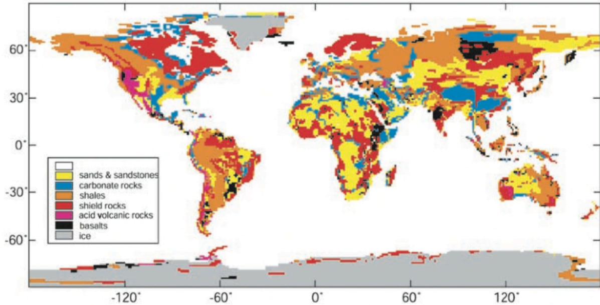
Figure II.4 : Représentation des différents types de lithologie (résolution de 1^\circ \times 1^\circ ), d'après Amiotte-Suchet et al. (2003).
