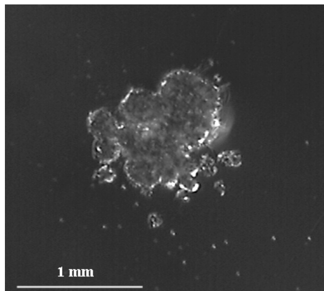
Figure 78 : Image en microscopie optique d'un dommage laser fait à une fluence comprise entre 30 et 40 \text{J}/\text{cm}^2 à 3\omega .
