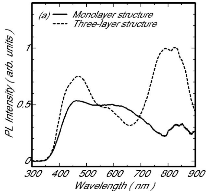
Figure 30 : Spectre de luminescence des échantillons de silice ; en trait plein, le spectre correspondant à la structure monocouche et en pointillé celui correspondant à la structure à trois couches [44].
