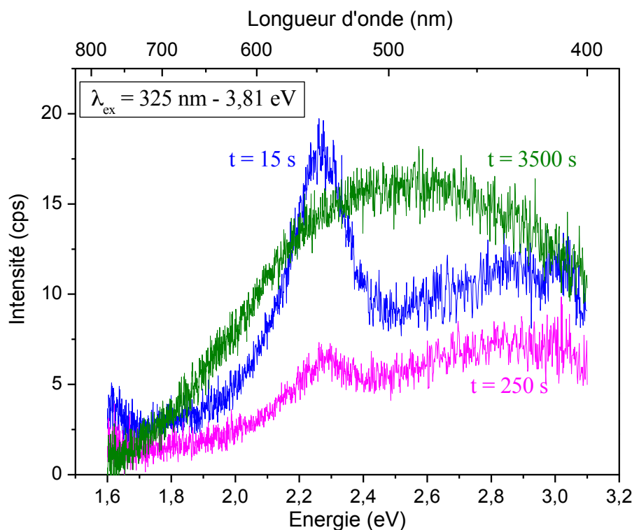
Figure 123 : Comparaison des spectres de luminescence obtenus sur une indentation en fonction du temps d'irradiation.
