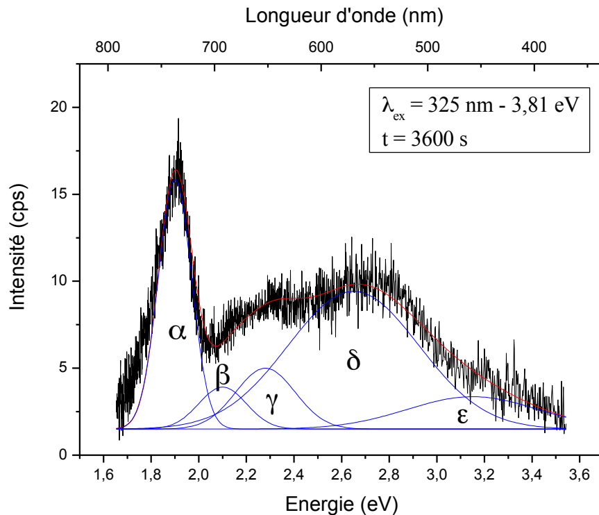
Figure 126 : Spectres de photoluminescence pour un dommage laser sous excitation à 3,81 eV (325 nm). (a) temps d'irradiation 45 secondes. (b) temps d'irradiation 250 secondes. (c) temps d'irradiation 3600 secondes. En noir : données expérimentales ; En rouge : décomposition du signal ; En bleu : Composantes gaussiennes du signal.
