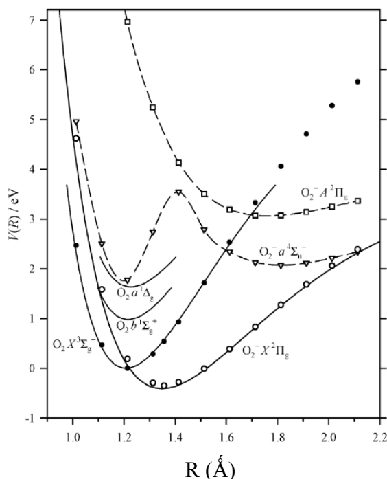
Figure 52. Energies potentielles calculées pour l'état fondamental de la molécule de dioxygène ( O_2 X^3\Sigma_g^- , -.-), pour l'état fondamental de l'ion O_2^- ( O_2^- X^2\Pi_g , -o-), et pour les états excités de l'ion O_2^- ( a^4\Sigma_u^- , -∇- et O_2^- A^2\Pi_u , -□-), correspondant aux deux premières transitions électroniques [76].
