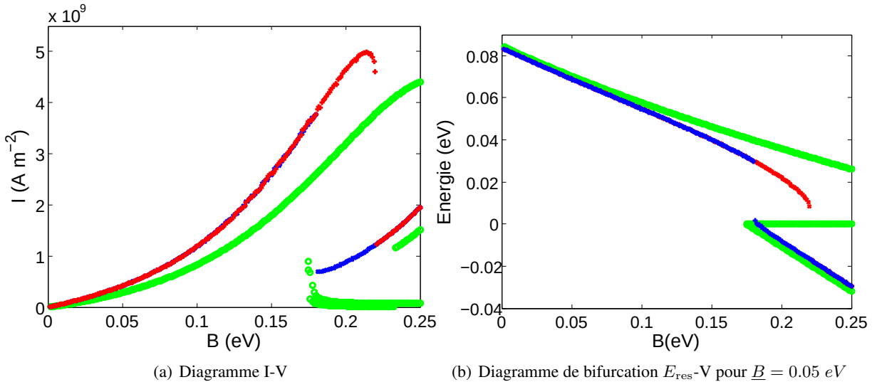
FIGURE 2.3 – Comparaison du modèle réduit et d'un modèle complet : modèle réduit (o), méthode de continuation en augmentant la DDP (+) et en la diminuant (x).
