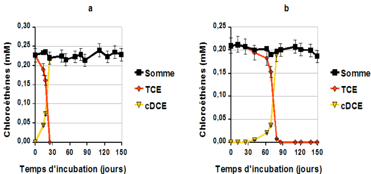
FIGURE 11.4 – Evolution des concentrations en chloroéthènes avec deux concentrations en sulfates différentes, (a) 100 \text{ mg.L}^{-1} et (b) 250 \text{ mg.L}^{-1}
