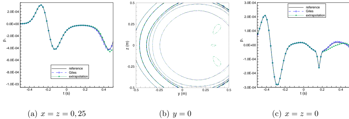
FIG. 2.33 – Résultats de la propagation de l'onde. Contours : fin : p = \Delta p_{min}/2 , épais : p = \Delta p_{max}/2 , intermédiaire : p = 0 . (—) résultats numériques sur domaine infini, (--) et (○○○) solutions numériques sur domaine tronqué : méthode de Giles, (····) et (△△△) solutions numériques sur domaine tronqué : méthode d'extrapolation.
