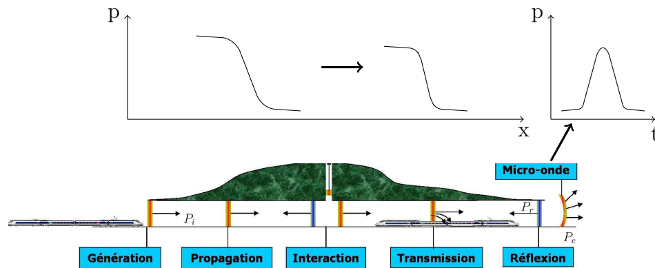
FIG. 1.1 – Ondes de pression dans un tunnel ferroviaire.
