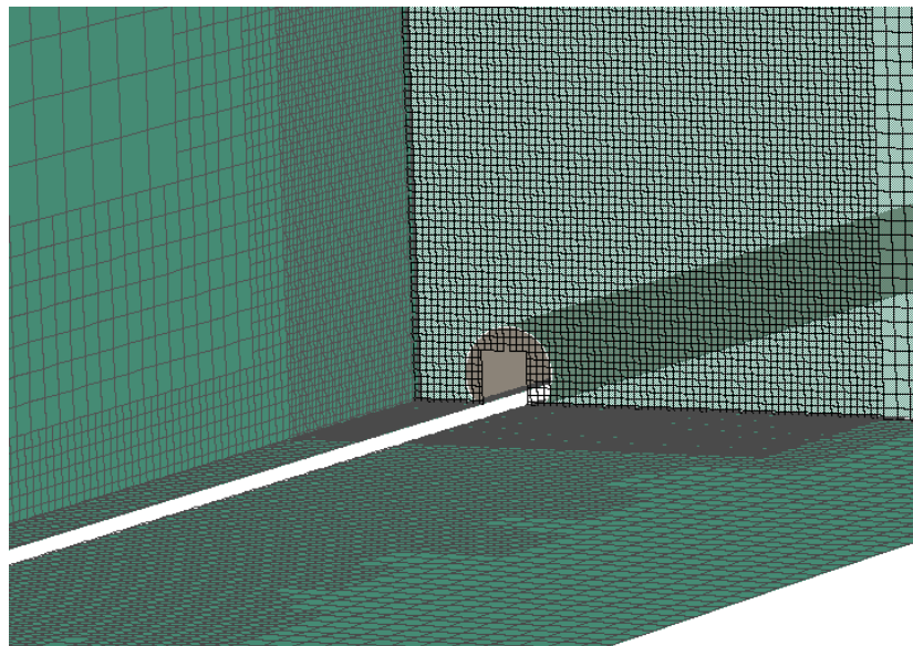
FIG. 2.3 – Maillage du domaine restant.
