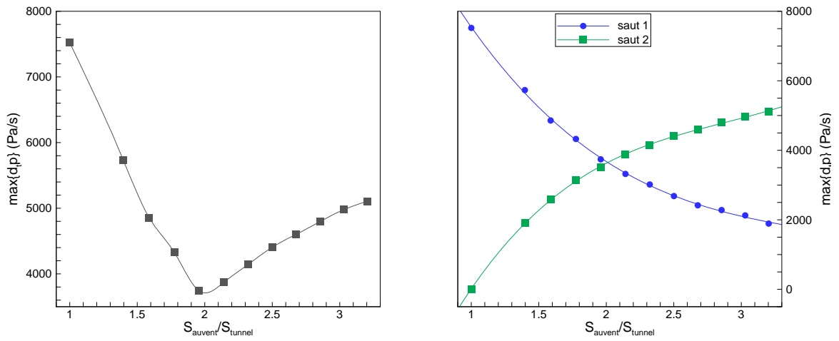
(a) maxima du gradient de pression
