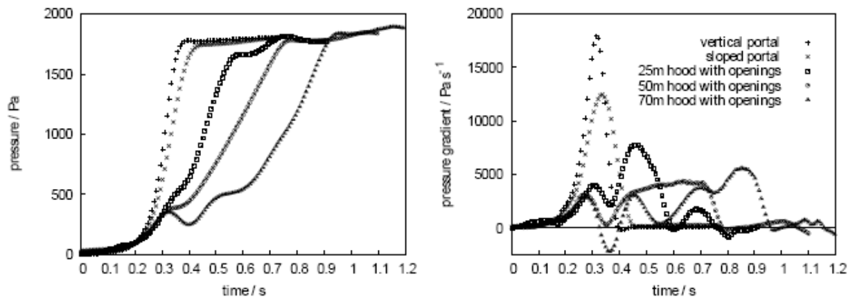
FIG. 1.9 – Résultats expérimentaux et numériques [4].
