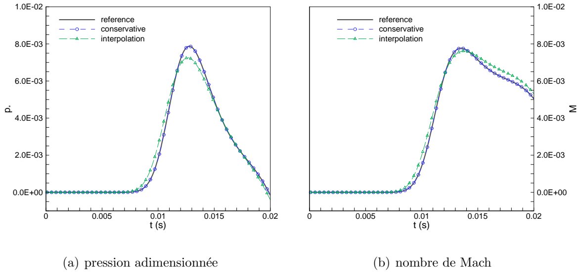
FIG. 2.21 – Effet de la communication des variables entre deux domaines, capteur B, V_e = 0 \text{ m.s}^{-1} .
