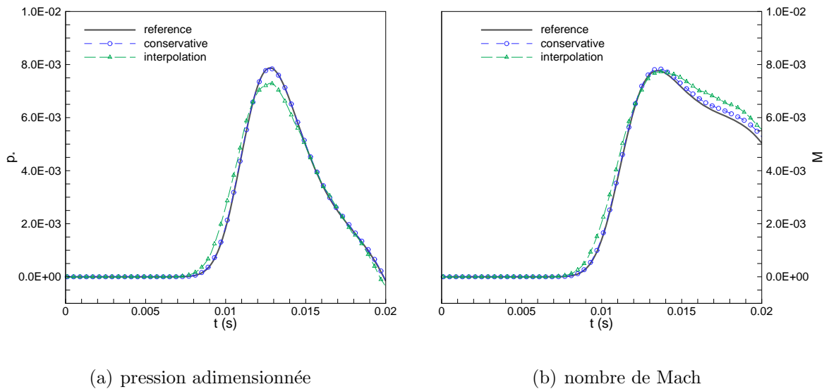
FIG. 2.22 – Effet de la communication des variables entre deux domaines, capteur B, V_e = 70 \text{ m.s}^{-1} .
