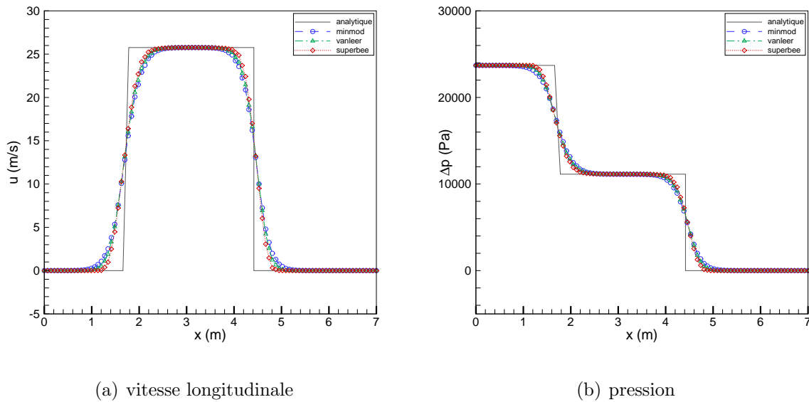
FIG. 2.10 – Effet des limiteurs.
