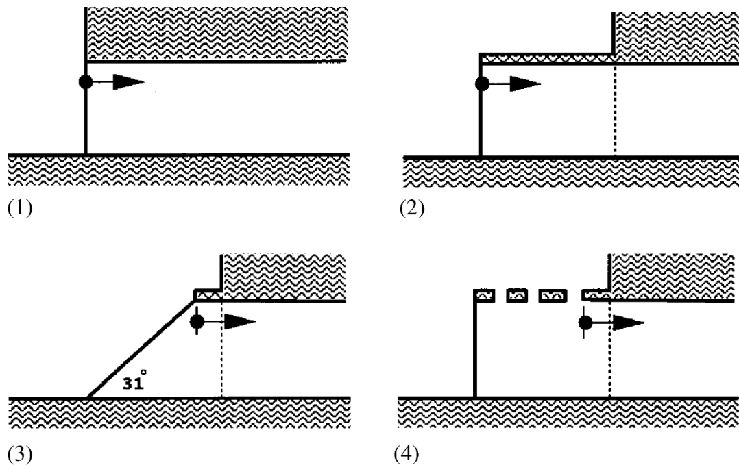
FIG. 1.6 – Exemples d'auvent [2]
