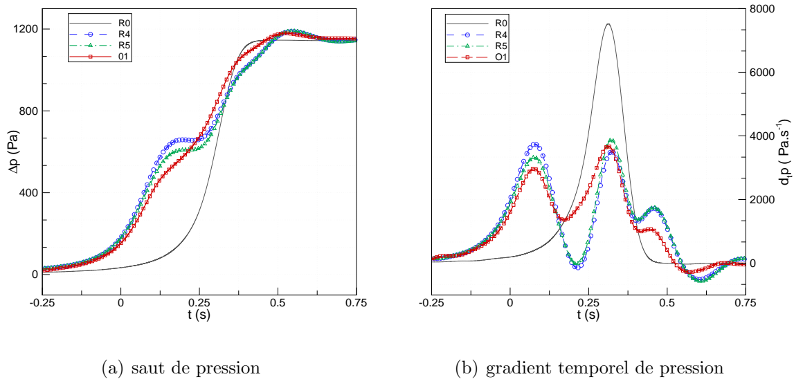
FIG. 4.29 – Sauts et gradients de pression.
