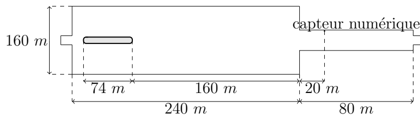
FIG. 3.13 – Dimensions du calcul.
