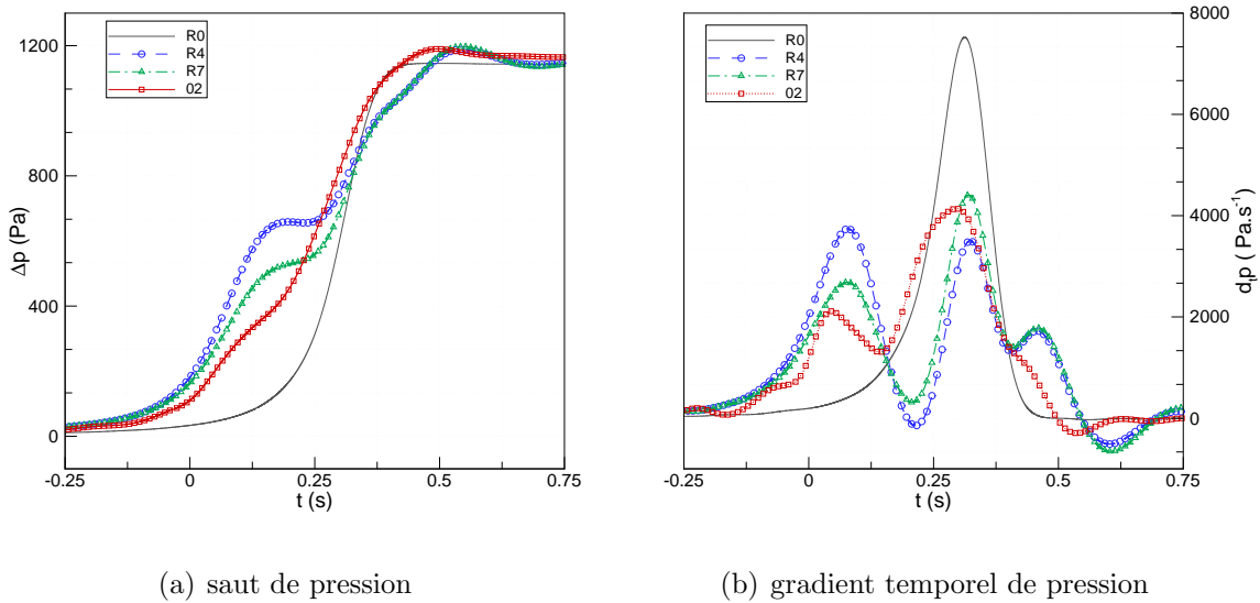
FIG. 4.31 – Sauts et gradients de pression.
