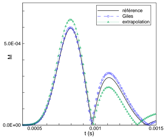
(a) capteur unidimensionnel
