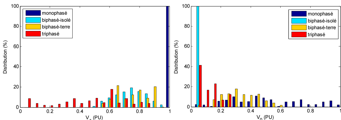
Figure 19-3 – Répartition des valeurs des tensions directes et homopolaires en présence de différentes classes de défauts pour différentes configurations d'un réseau impédant (extrait de la base de données simulées)
