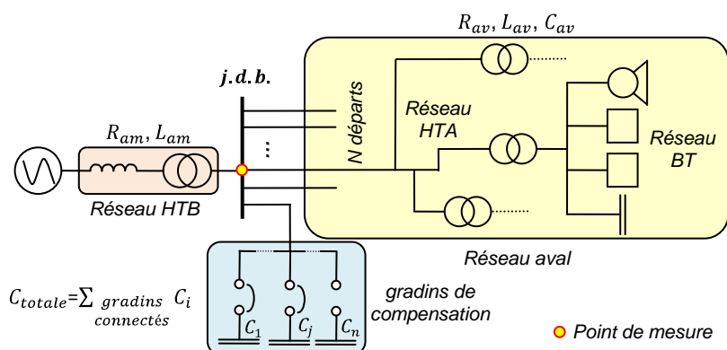
Figure 2-10 – Schéma monophasé équivalent présentant les principaux paramètres conditionnant les perturbations d'enclenchements d'un gradin observé du jeu de barres du poste HTB-HTA
