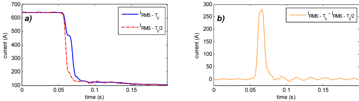
Figure 14-6 – Evolution de l'écart des valeurs efficaces d'un courant de ligne pendant le transitoire d'apparition d'un défaut biphasé
