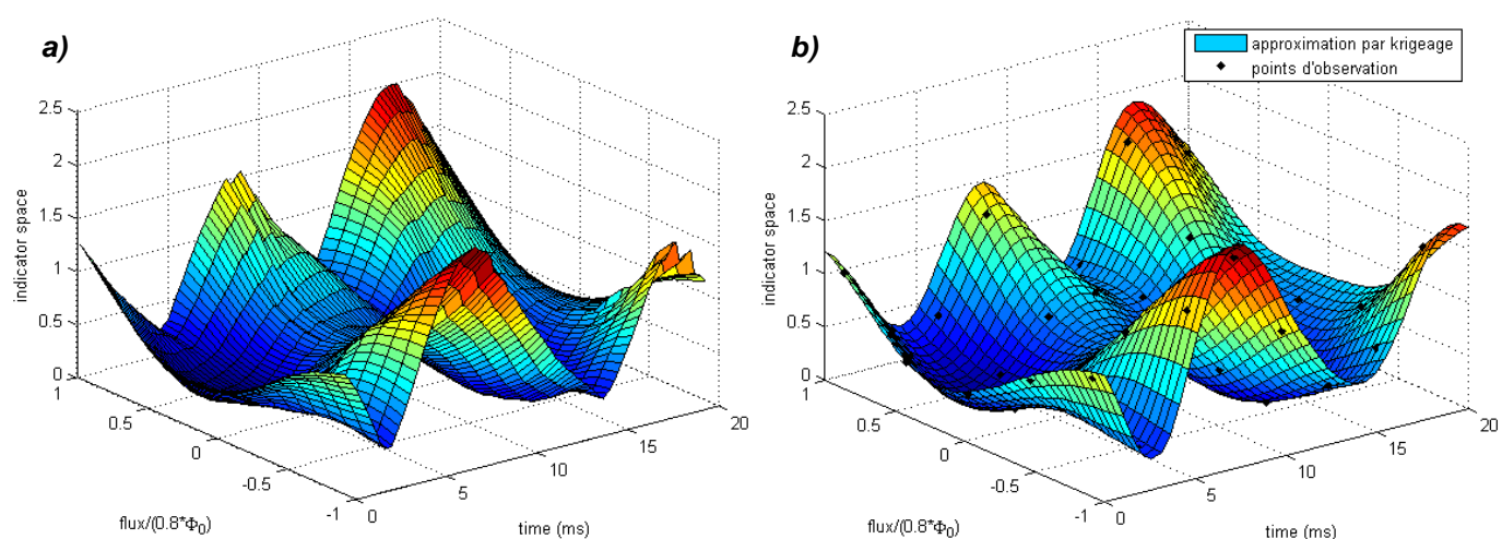
Figure 18-5 – Comportement d'un indicateur lié à l'intensité de l'appel de courant à l'enclenchement pour des instants d'enclenchement et des valeurs de flux rémanent différents
