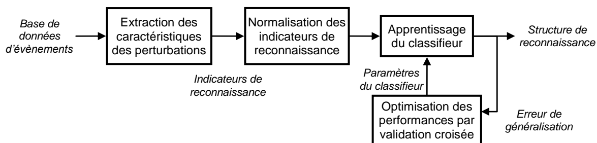
Figure 3-8 – Schéma générique d'apprentissage des méthodes à apprentissage supervisé
