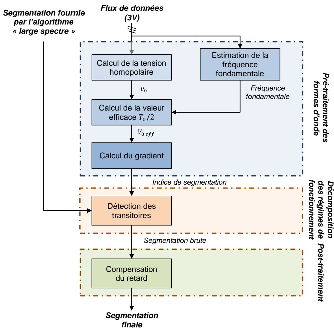
Figure 10-2 – Architecture du procédé d'identification des régimes de fonctionnement
