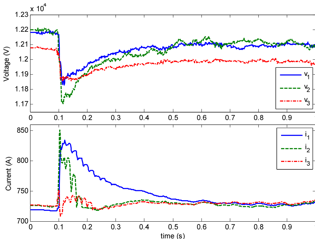
Figure 20-2 – Exemple de perturbations « atypiques »
