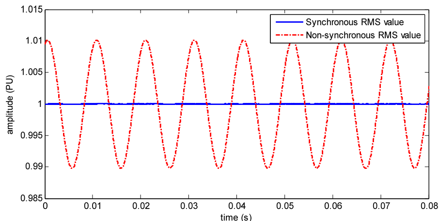
Figure 7-1 – Comportement de la valeur RMS d'un signal à 49 Hz pour une fenêtre synchrone (adaptée à f_0 = 49\text{ Hz} ) et une fenêtre non synchrone (adaptée à f_0 = 50\text{ Hz} )
