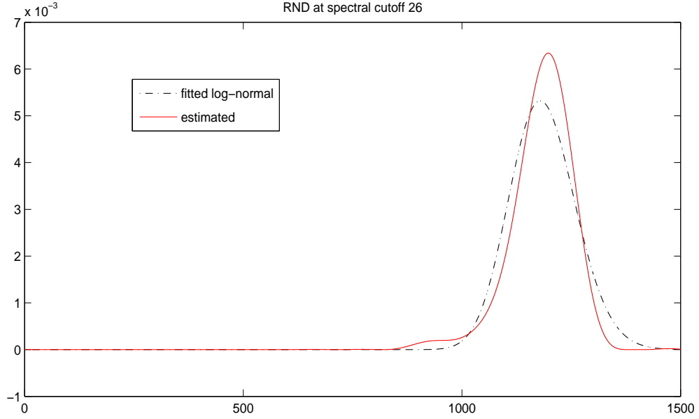
FIGURE 1.11 – Cette figure représente la RND q_{26}^{\star} (ligne continue) estimée à partir de prix d'options de vente réels (bid et ask) sur le S&P500. On choisit B = 1.4 * F_0 = 1.4 * S_0 * e^{(r-\delta)\tau} = 1660 . De plus, on représente la meilleure approximation log-normale de q obtenue par moindres carrés par rapport aux prix d'options cotés moyens (ligne pointillée).
