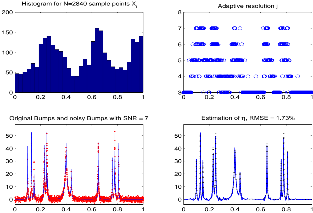
FIGURE 1.2 – Dans le sens des aiguilles d’une montre à partir de la figure en haut à gauche, on représente : un histogramme des points X_i qui constituent le design ; le niveau de résolution choisit de manière adaptative par la méthode de Lepski en chaque point X_i du design ; le vrai signal f (points noirs) ainsi que l’estimateur f^\circledast (ligne bleue continue) en chaque point X_i ; et finalement le signal original f (ligne bleue continue) accompagné de sa version bruitée Y_i aux points X_i (points rouges).
