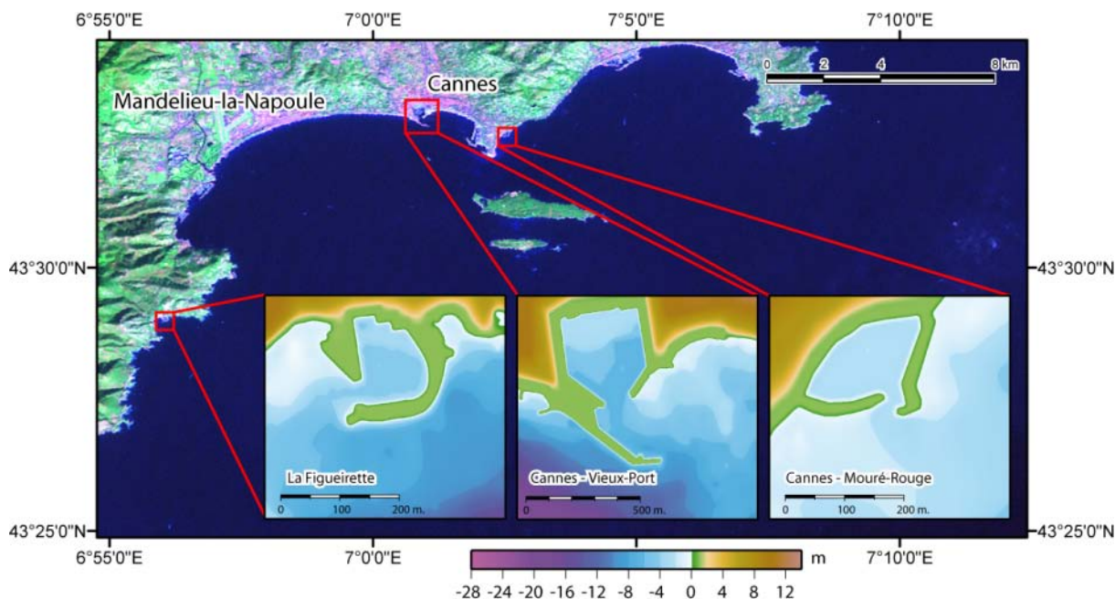
Figure 93. Cartographie et bathymétrie des trois ports retenus pour la modélisation (fond de carte Landsat).
