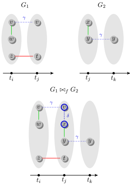
Figure 44 – Exemple de jointure de filiation entre G_1 = (V_1, E_1, T_1) et G_2 = (V_2, E_2, T_2) tel que \rho_f[t, y] , avec t \in X(t_i) \subseteq V_1 , y \in X(t_i) \subseteq V_2 , et \rho_f une relation de dérivation dans \Phi .
