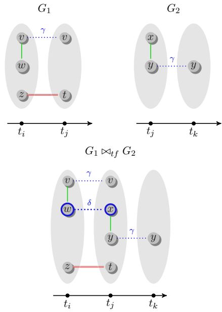
Figure 45 – Exemple de jointure de filiation temporelle, entre G_1 = (V_1, E_1, T_1) et G_2 = (V_2, E_2, T_2) tel que \rho_f[w, x] , avec w \in X(t_i) \subseteq V_1 , x \in X(t_j) \subseteq V_2 , t_i < t_j , et \rho_f \in \Phi .
