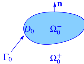
FIGURE 5.2 – Objet diffractant D_0 (sans cavité).
