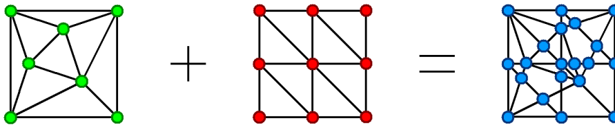
FIG. 28. – Dès la dimension 2, la création d’un maillage union à partir des maillages en présence n’est pas aisée : de nouveaux nœuds et de nouvelles mailles peuvent apparaître.
