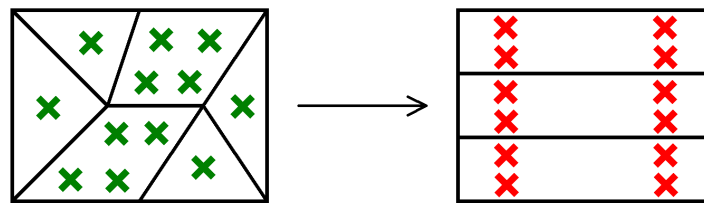
Le champ connu aux points de Gauss du maillage initial (à gauche) doit être transféré aux points de Gauss du maillage final (à droite).
