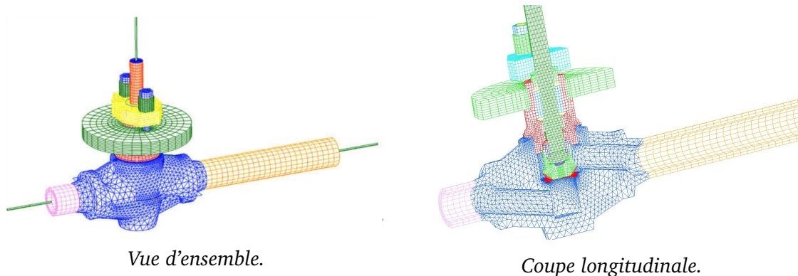
FIG. 3. – Maillage du robinet à soupape et de quelques éléments attenants, contenant plus de 140 000 éléments (crédit EDF).
