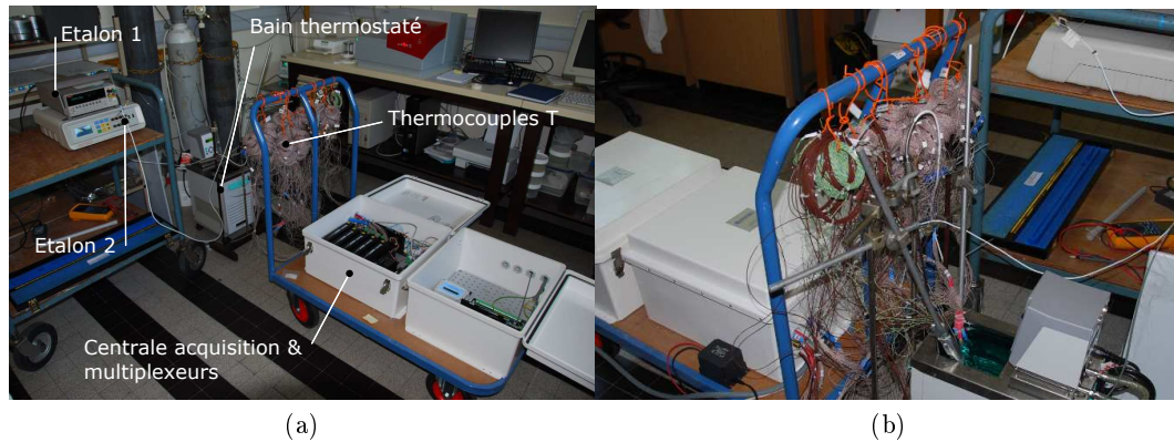
FIGURE 3.2 – Dispositif d’étalonnage en température (thermocouples et fluxmètres).
