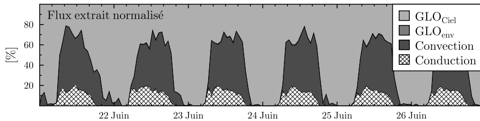
FIGURE 3.23 – Contribution normalisée des modes de transferts au rafraichissement de la peau extérieure pour la période du 21 au 27 Juin.
