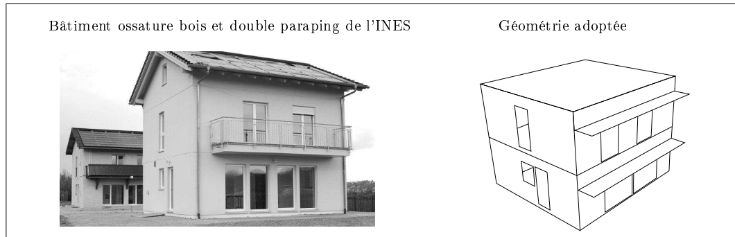
FIGURE 2.5 – Photo des bâtiments expérimentaux de l'INES et modèle géométrique simplifié.
