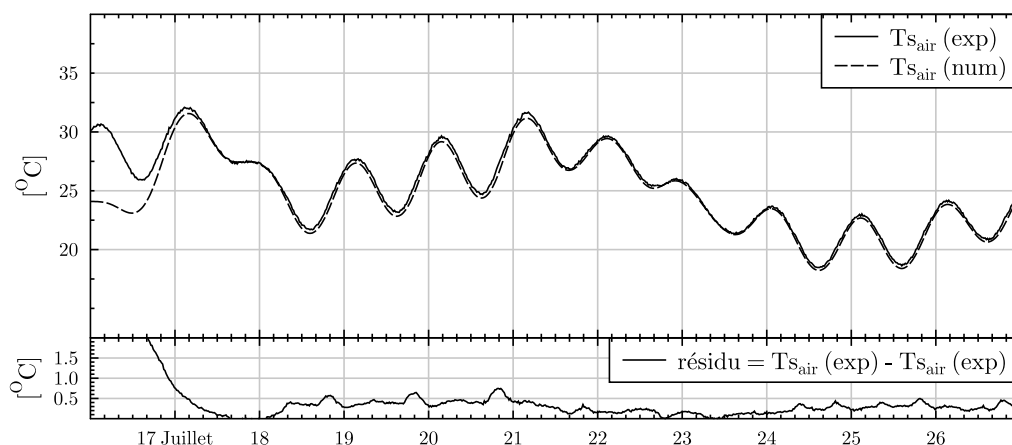
FIGURE 4.5 – Fonctionnement permanent, résultats après calibration du modèle pour la période du 16 Juillet au 27 Juillet 2010 ( hc = 11.8 \text{ W.m}^{-2}.\text{K}^{-1} et Li = 18.5 \text{ cm} ).
