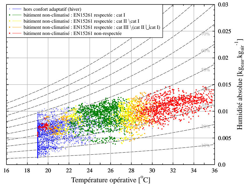
FIGURE 1.6 – Zone de confort calculées selon le standard adaptatif de la norme NF-EN-15251 sur le diagramme psychrométrique.
