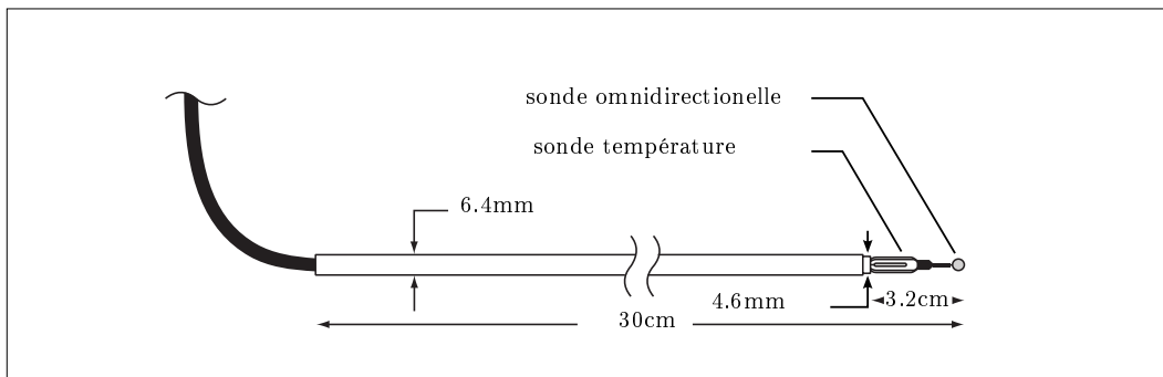
FIGURE 3.6 – Anémomètre TSI 8475
