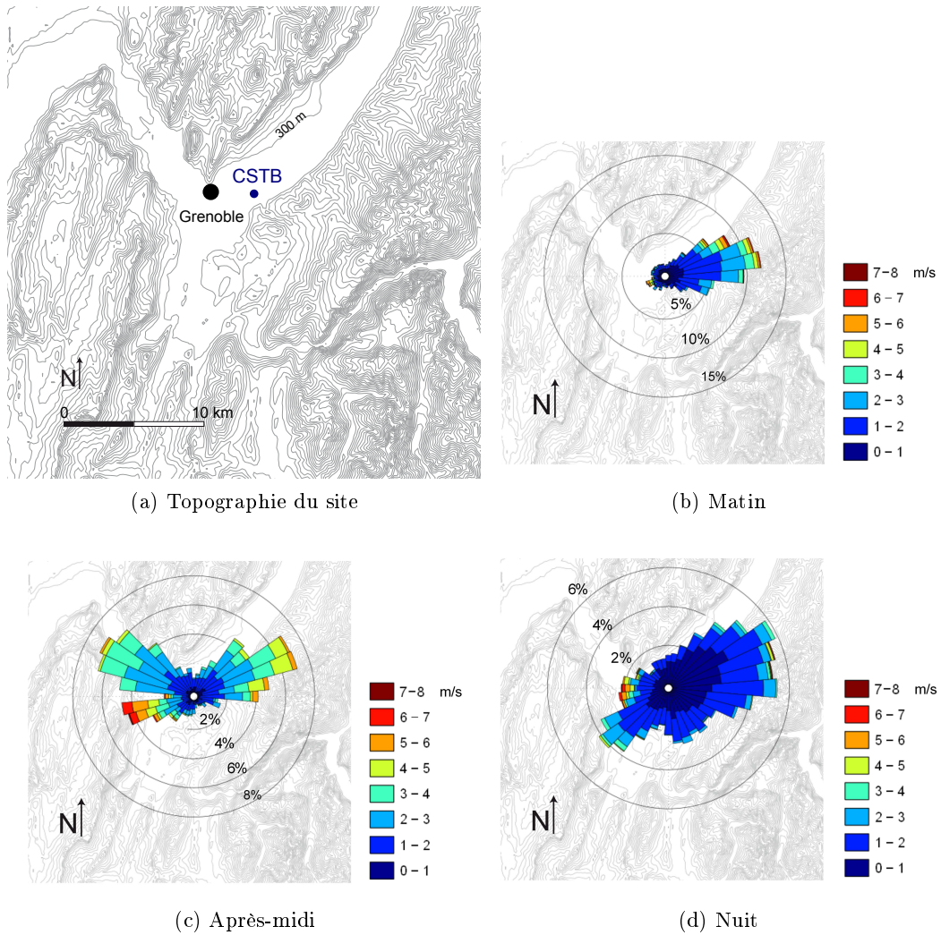
FIGURE 3.10 – Rose des vents du mois d’Avril 2010 (provenance ( \angle ), fréquence (%)) et gamme de vitesse ( m.s^{-1} )).
