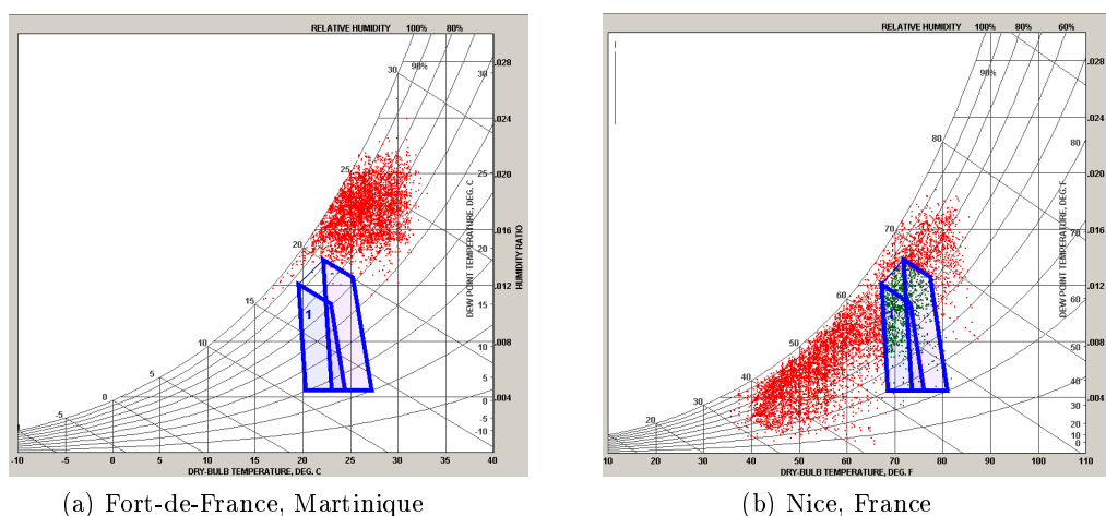
(a) Fort-de-France, Martinique (b) Nice, France FIGURE 1.17 – Sollicitations en climat chaud-humide et méditerranéen
