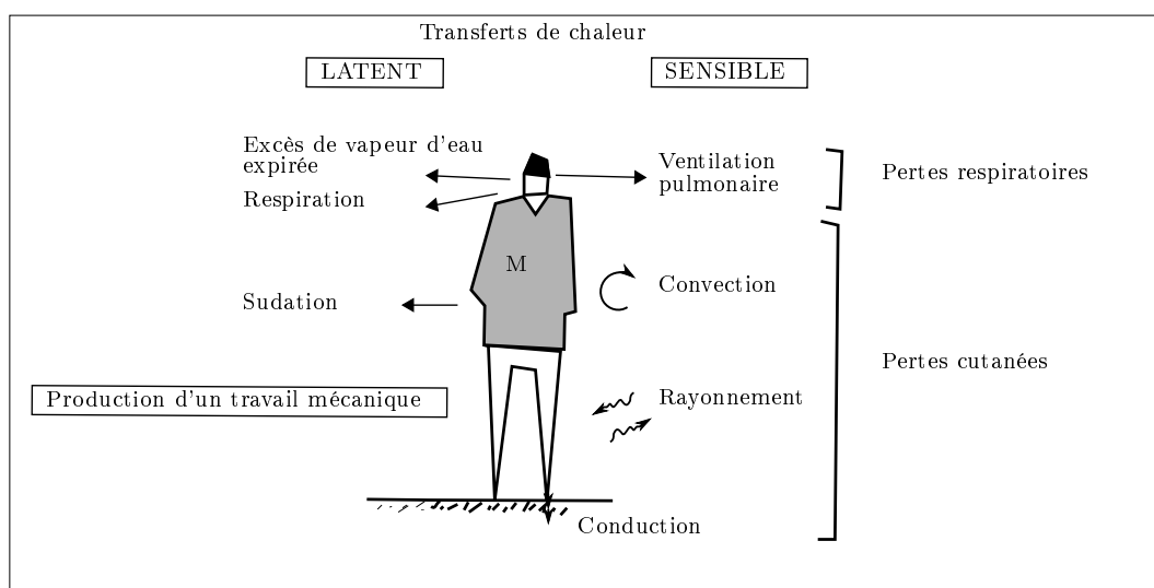
FIGURE 1.2 – Représentation des vecteurs de transfert de chaleur entre l'homme et son environnement.
