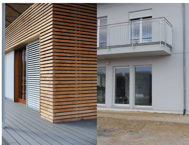
(a) Bardage à clair-voie. (b) Complexe de crépis collé.
