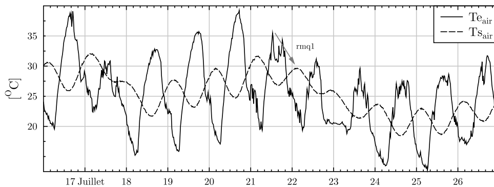
FIGURE 3.34 – Évolution d'entrée et de sortie de l'air relevées pour un fonctionnement permanent du ventilateur .
