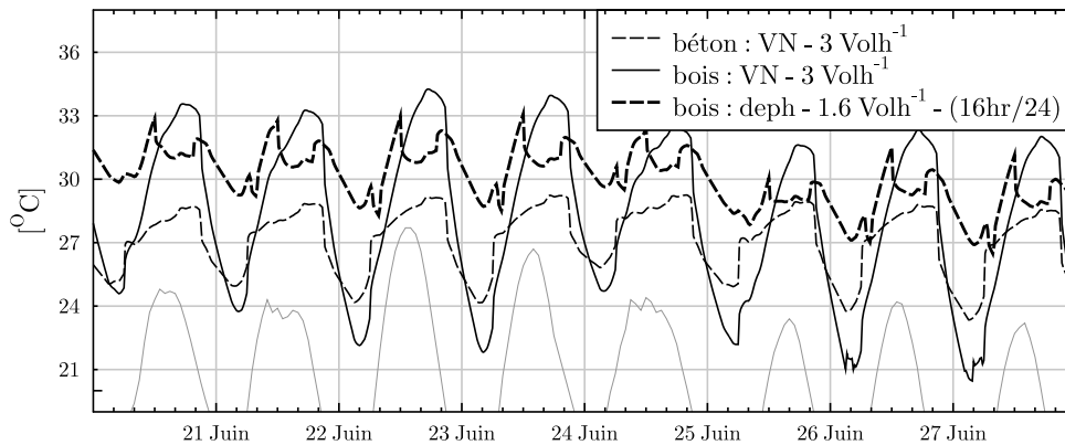
FIGURE 4.14 – Comparaison de la configuration bois utilisant stock thermique ou ventilation nocturne à celle d’une configuration béton ventilée la nuit.
