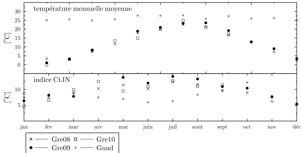
FIGURE 2.36 – Contraste thermique jour/nuit mensuel pour le site de Grenoble ainsi que pour une année en Guadeloupe.
