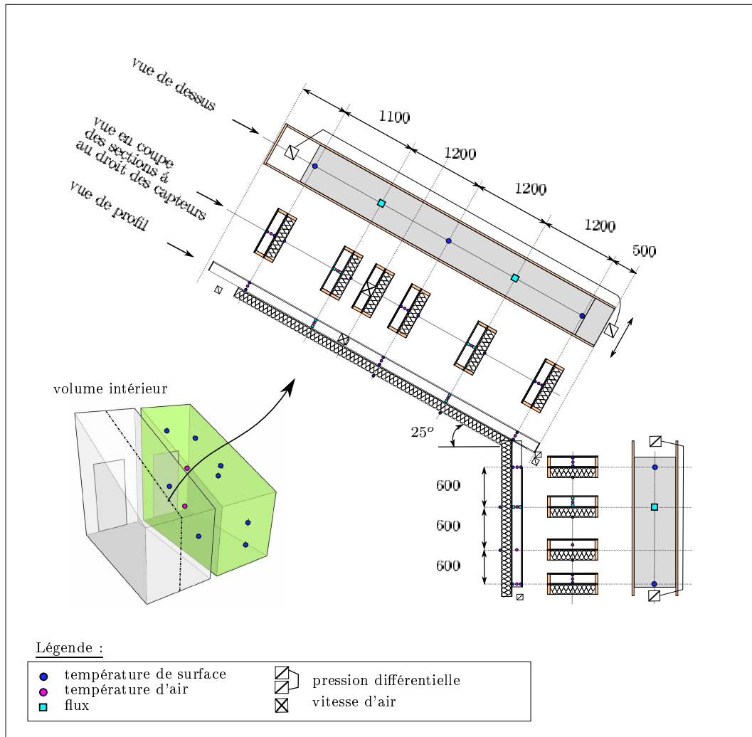
FIGURE 3.14 – Plan d'instrumentation du demi-volume Est
