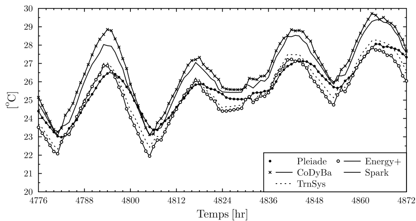
FIGURE 2.6 – Évolution des températures durant la période estivale pour les 5 outils de simulation dynamique.
