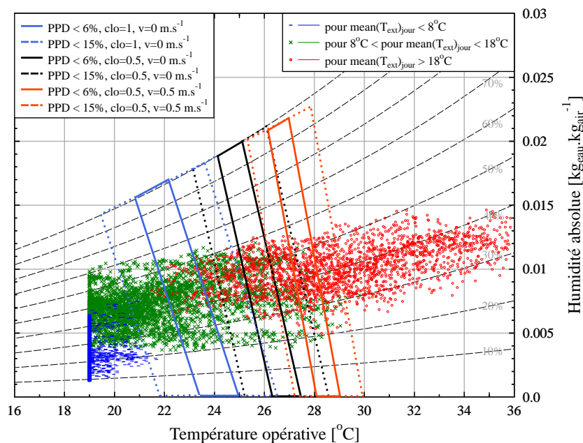
FIGURE 1.3 – Calcul des zones respectant le critère de confort selon FANGER pour un habillement d'hiver et d'été ainsi que pour une vitesse de l'air augmentée.
