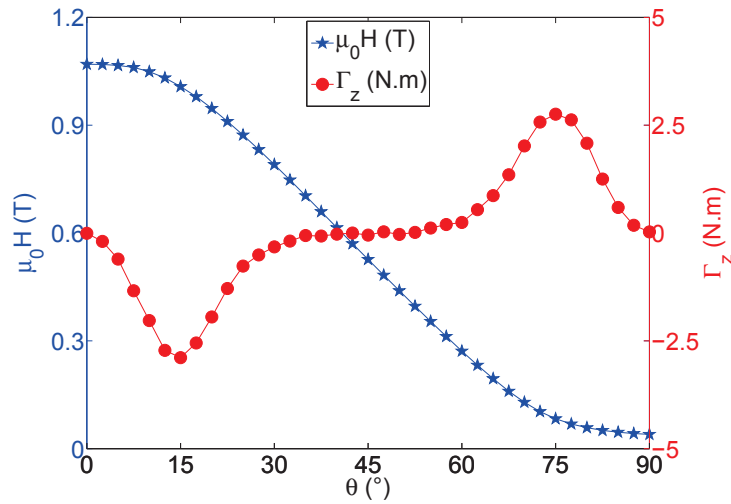
Fig. 4.21 – Évolution de la force et du champ moyen en fonction de la position.
