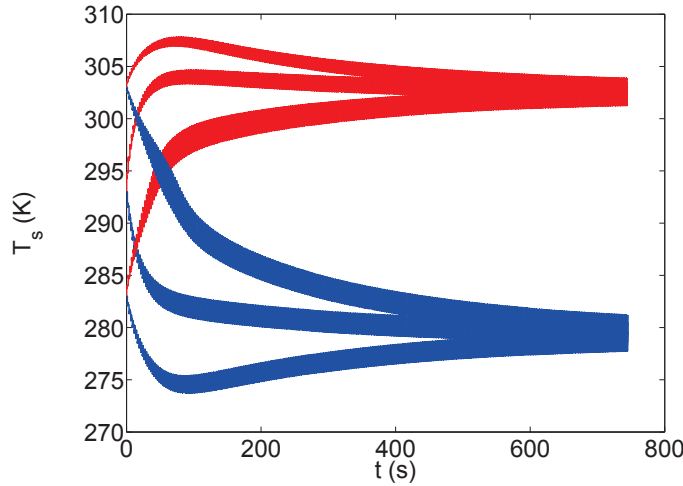
Fig. 3.15 – Évolution temporelle de la température dans le solide à puissance nulle, pour différentes conditions initiales ( T_0 = 303\text{ K} , T_0 = 293\text{ K} et T_0 = 283\text{ K} ).
