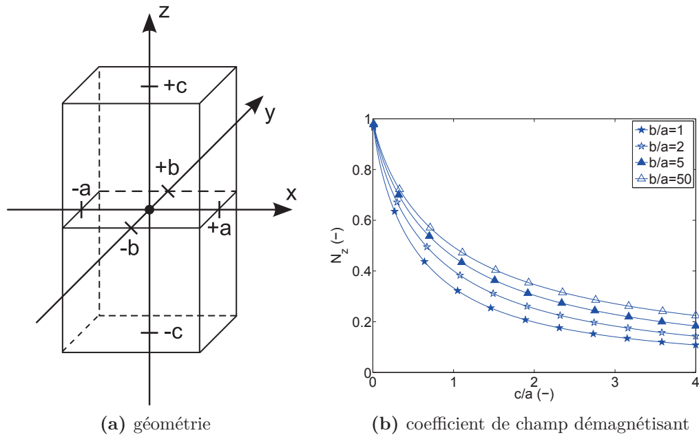
Fig. 5.17 – Prisme rectangulaire.
