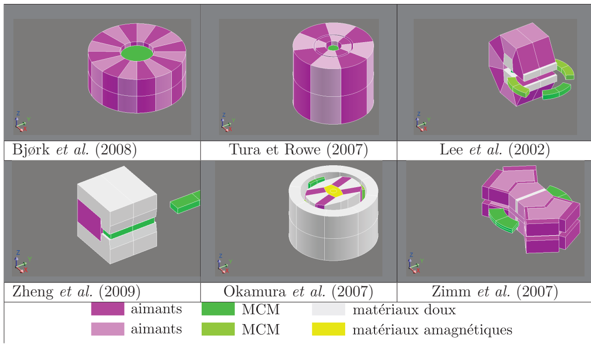
Fig. 4.11 – Structures d'aimants étudiées.
