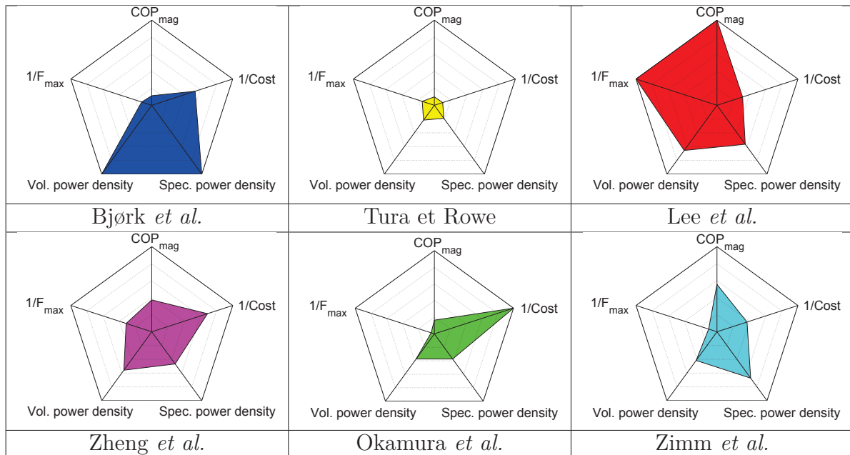
Fig. 4.37 – Comparaison des performances des différentes structures.
