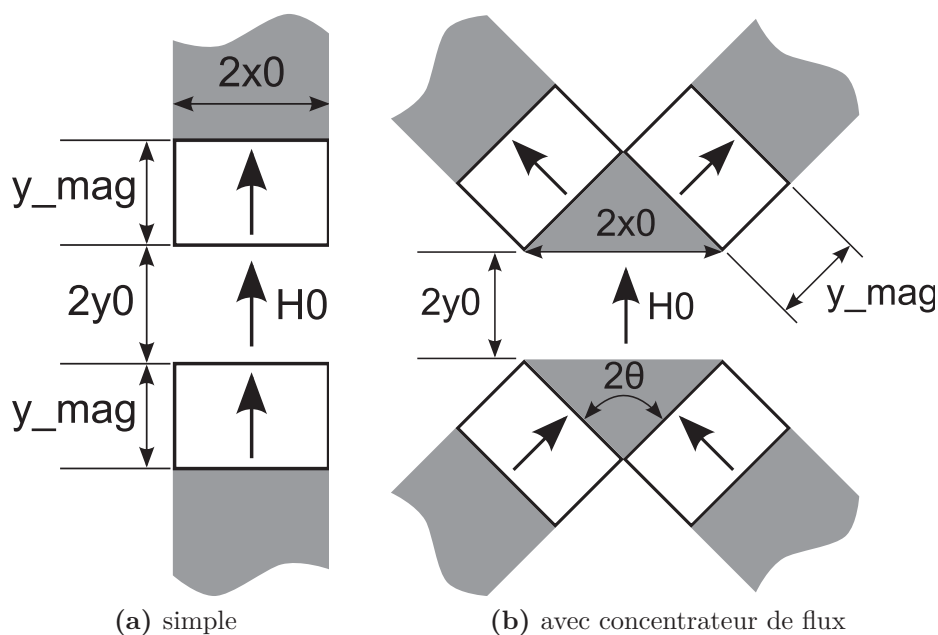
Fig. 5.11 – Circuit magnétique.
