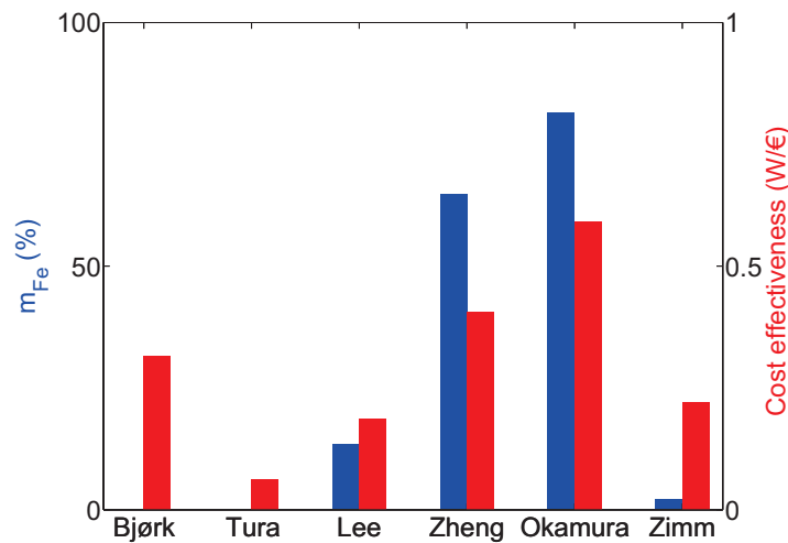
Fig. 4.40 – Corrélation entre la masse relative de fer et le prix des structures.
