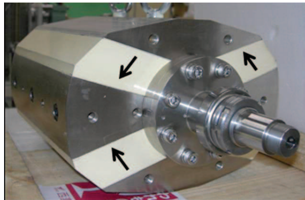
Fig. 4.10 – Géométrie de la structure d'aimants de Okamura et al. [Okamura et al. , 2007].
