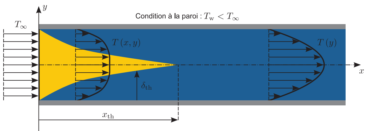
Fig. 3.7 – Évolution de la couche limite hydrodynamique pour un écoulement bidimensionnel dans une conduite, en régime laminaire.
