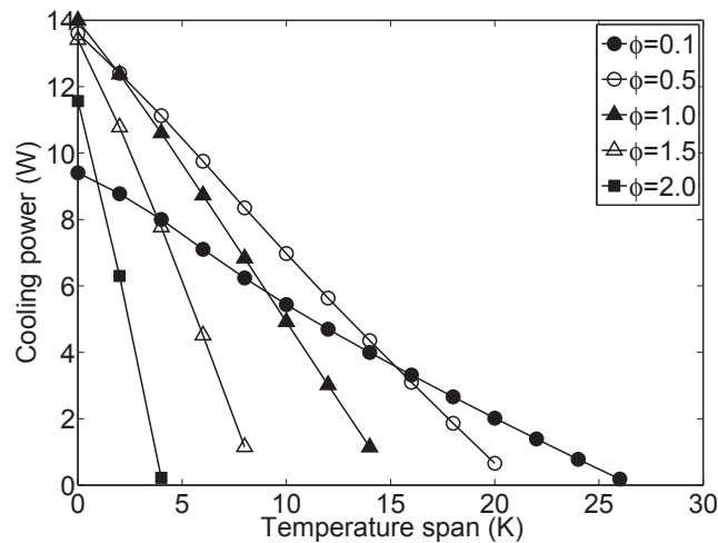
Fig. 3.21 – Puissance froide en fonction de l'écart de température et de \phi ( NTU = 50 ).
