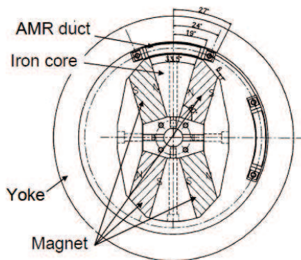
Fig. 4.10 – Géométrie de la structure d'aimants de Okamura et al. [Okamura et al. , 2007].
