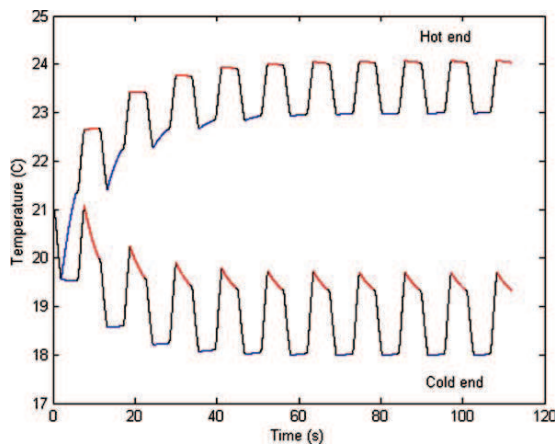
(a) Modèle de Shir et al. .
