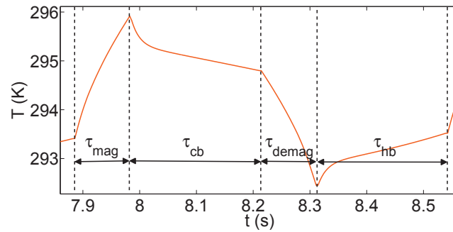
Fig. 3.19 – Zoom sur l'évolution temporelle de la température au centre du régénérateur durant une période du cycle.
