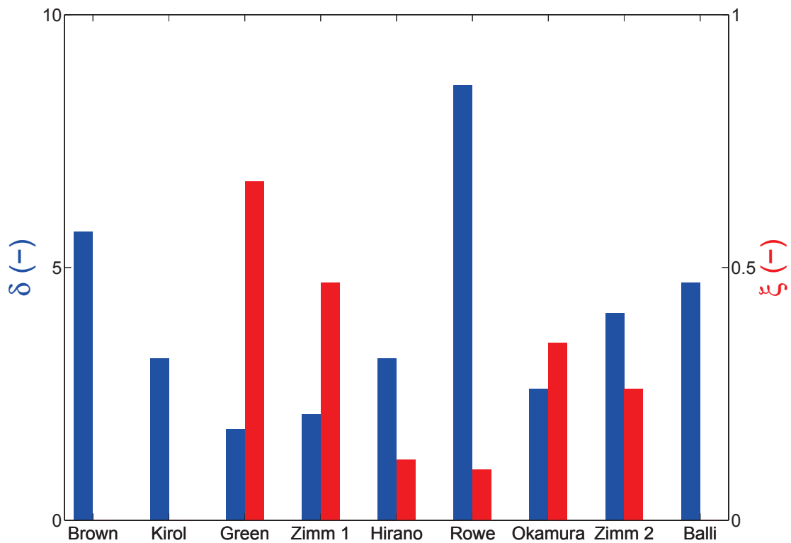
Fig. 2.25 – Comparaison des prototypes de réfrigération magnétique.
