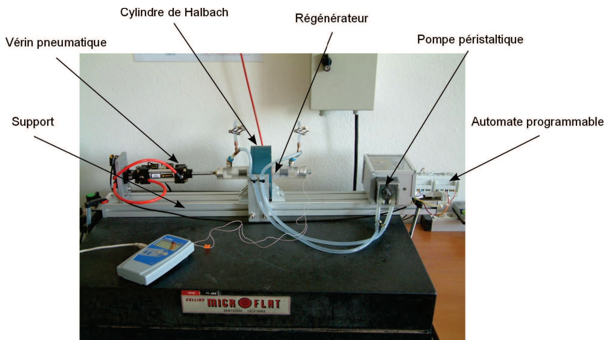
Fig. 5.1 – Photo du démonstrateur du G2Elab.
