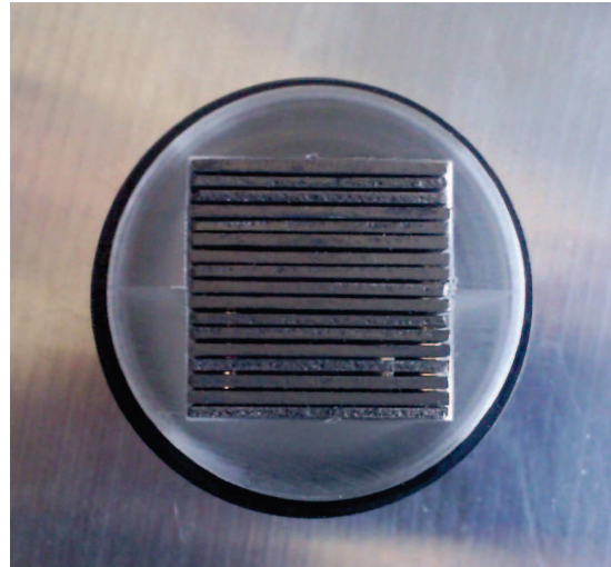
(b) Photo du régénérateur modifié
