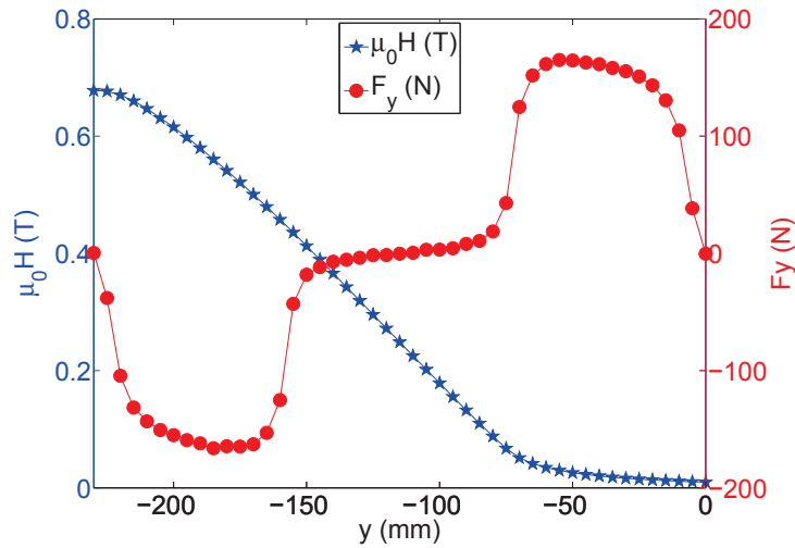
Fig. 4.25 – Évolution de la force et du champ moyen en fonction de la position.
