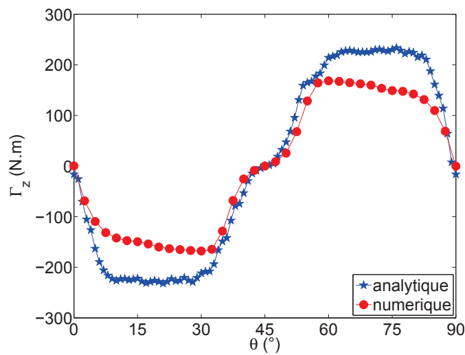
Fig. 4.30 – Calcul numérique et semi-analytique du couple \Gamma_z .
