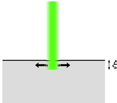
FIGURE I.14 – Régime thermoélastique : le faisceau laser pénètre dans le matériau sur la profondeur optique \xi et crée une source acoustique compressive parallèle à la surface.
