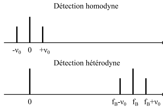
FIGURE I.17 – Principe de l'hétérodynage : le signal utile est transposé autour de la fréquence f_B (fréquence de Bragg) pour s'affranchir des bruits basses fréquences.
