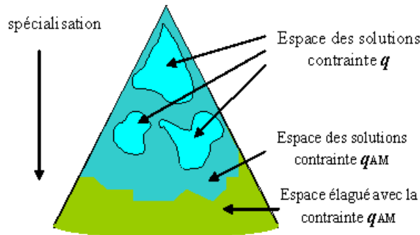
FIG. 5.4 – Les espaces de solutions dans le cas d'une relaxation
