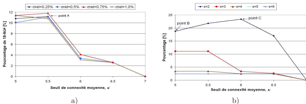
FIG. 6.29 – a) Le pourcentage de pixels purs couverts par les 18-MSFG en fonction du seuil de connexité moyenne, \kappa , et du seuil du support relatif \sigma_{rel} , pour s = 3 et b) Le pourcentage de pixels purs couverts par les 18-MSFG en fonction du seuil de connexité moyenne, \kappa , et du nombre de symboles, s , pour \sigma_{rel} = 0,5\% .
