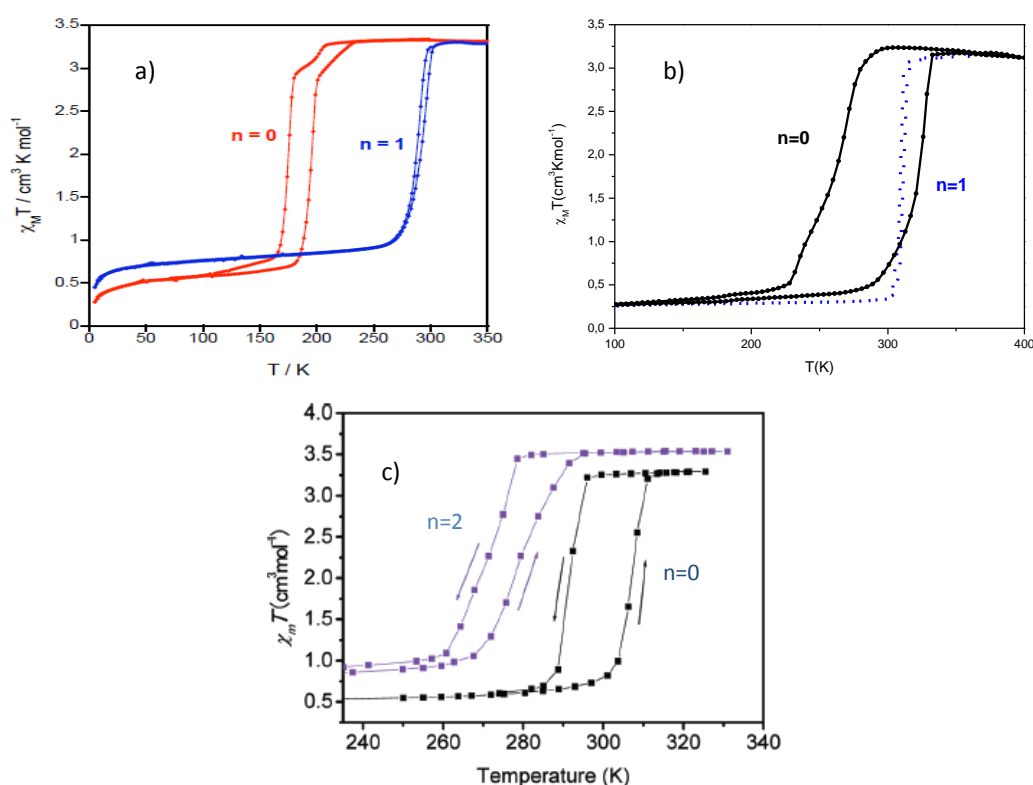
Figure B.3.2.1.- Dépendance thermique de \chi T pour les complexes Fe(L)Pt(CN)_4.nH_2O ( L = azpy (a), bpac (b) et pz (c))
