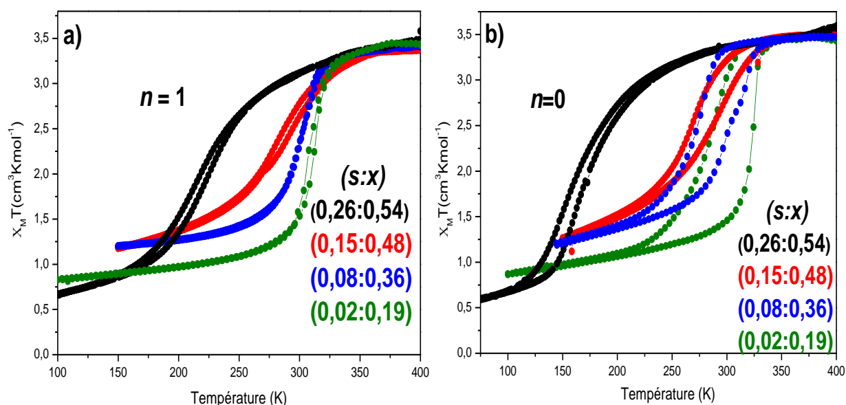
Figure B.2.7.3 - Étude du changement de comportement magnétique en fonction de s pour x variant peu sous a) forme hydratée ( n = 1 ) et b) forme déshydratée ( n = 0 ).
