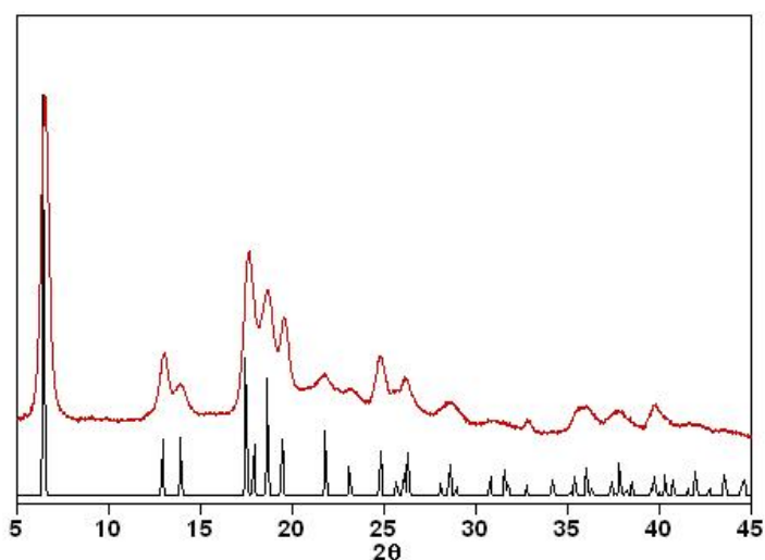
Figure B.2.4.3.- Spectre de diffraction expérimental obtenu à partir des mesures sur la poudre BI (rouge) et simulé obtenu à partir des mesures DRX sur monocristal (noire).
