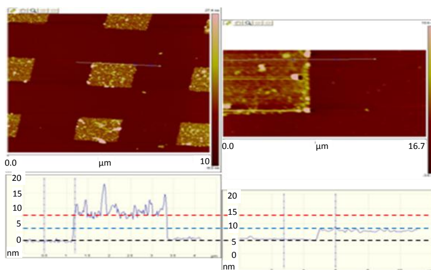
Figure C.1.5.10 - Images AFM et étude du profil du système \{\text{Fe}(\text{pz})[\text{Pt}(\text{CN})_4]\} après 5 cycles de dépôt sur des motifs de 20 \mu\text{m} (à droite) et après 10 cycles de dépôt sur des motifs de 2 \mu\text{m} (à gauche). Les lignes pointillées représentent les épaisseurs théoriques.
