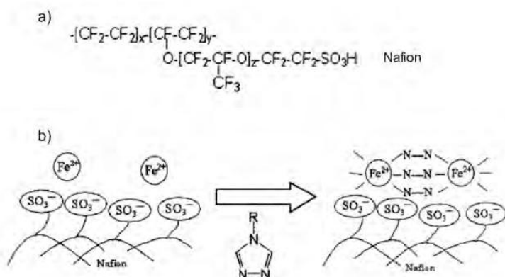
Figure A.3.4.5.- a) Formule moléculaire générale du Nafion, utilisé comme couche d'accrochage et b) Procédé d'élaboration des couches minces à partir du Nafion comme contre-ion (où N-N = R-trz).
