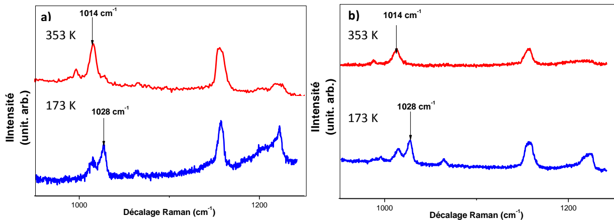
Figure C.2.4.2 – Spectre Raman des couche minces (1) (a) et (2) (b) à 173 et 353 K.
