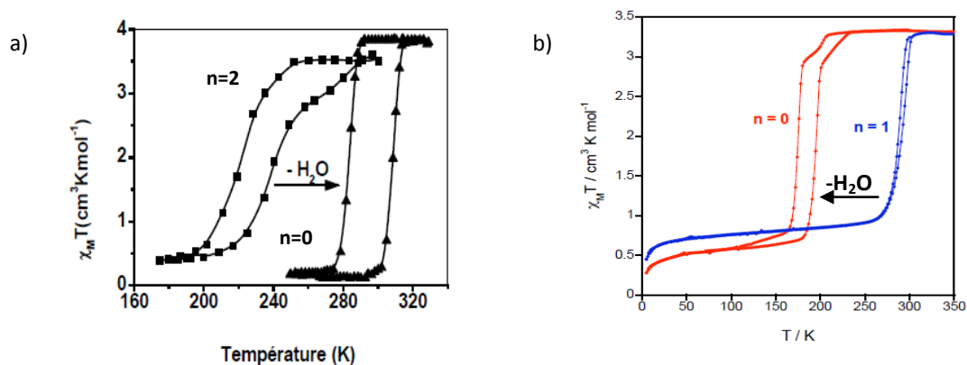
Figure B.2.1.1.- Courbes \chi_M T vs T pour les polymères a) \text{Fe}(\mathbf{pz})\text{Pt}(\text{CN})_4 \cdot n\text{H}_2\text{O} et b) \text{Fe}(\mathbf{azpy})\text{Pt}(\text{CN})_4 \cdot n\text{H}_2\text{O} .
