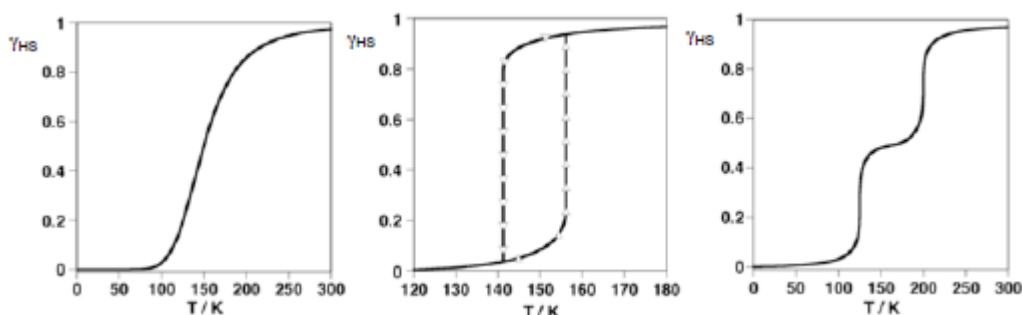
Figure A.1.7- Principaux types de courbes de transition de spin : graduelle (à gauche), abrupte avec hystérésis (au centre) et en deux étapes (à droite)
