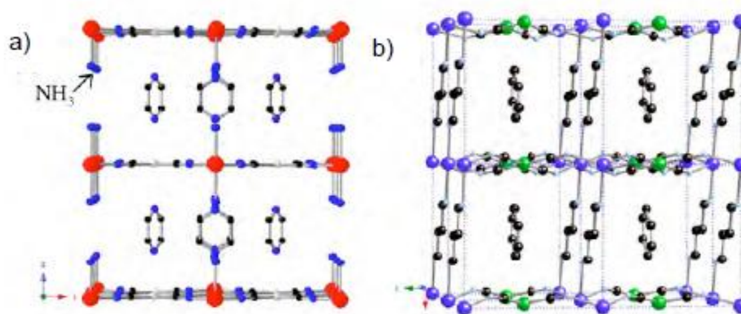
Figure A.2.2.4.-a) Perspective du clathrate d'Hofmann 2D \{\text{Ni}(\text{NH}_3)_2[\text{Ni}(\text{CN})_4]\} \cdot \text{benzène} b) Perspective du clathrate d'Hofmann 3D \{\text{Co}(1,4\text{-diaminobutane})[\text{Ni}(\text{CN})_4]\} \cdot \text{benzène}
