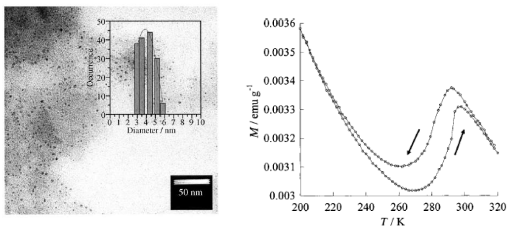
Figure A.3.4.9.- Image TEM et étude magnétique des nanoparticules de 4 nm du composé \text{Fe}(\text{pz})[\text{Ni}(\text{CN})_4] .
