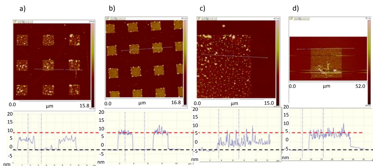
Figure C.1.5.11- Images AFM et étude du profil pour des motifs du système \{Fe(pz)[Pt(CN)_4]\} élaborés après 15 cycles de dépôt a) taille = 2 \mu\text{m} , [ ]_{réactifs} = 5\text{mM} , b) taille = 2 \mu\text{m} , [ ]_{réactifs} = 50\text{mM} , c) taille = 20 \mu\text{m} , [ ]_{réactifs} = 5\text{mM} et d) taille = 20 \mu\text{m} , [ ]_{réactifs} = 50\text{mM} .
