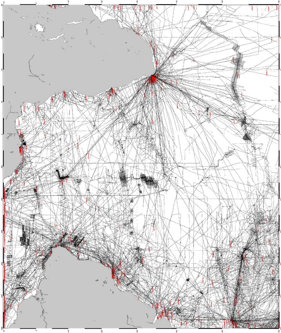
FIGURE 3.0.1: Carte A0 de localisation des points de données des campagnes disponibles dans la base de données du NGDC. A noter, l'irrégularité de distribution des campagnes, la concentration des données au large des grands ports et quelques vides au centre sud de l'océan.
