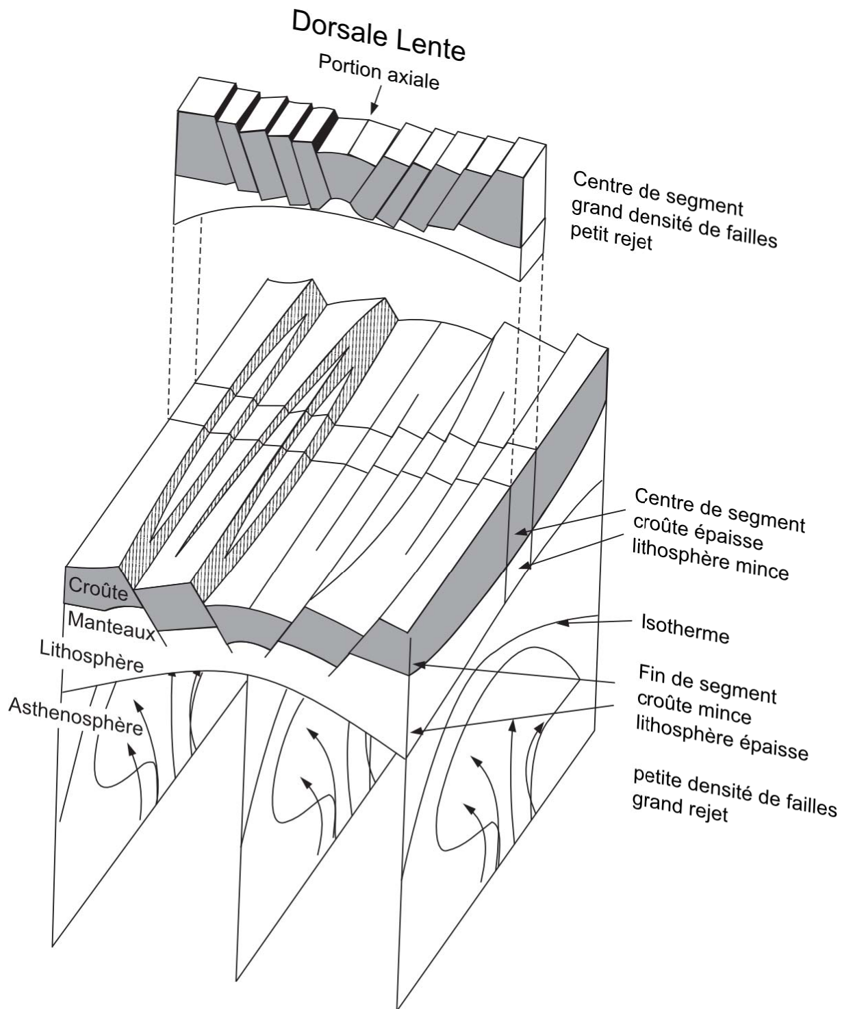
FIGURE 1.1.8: Schéma géologique d'un segment de dorsale lente montrant la variation le long de l'axe du centre vers les zones de fracture. L'apport magmatique est plus intense au centre du segment - l'effet de focalisation. D'après Macdonald (1998).
