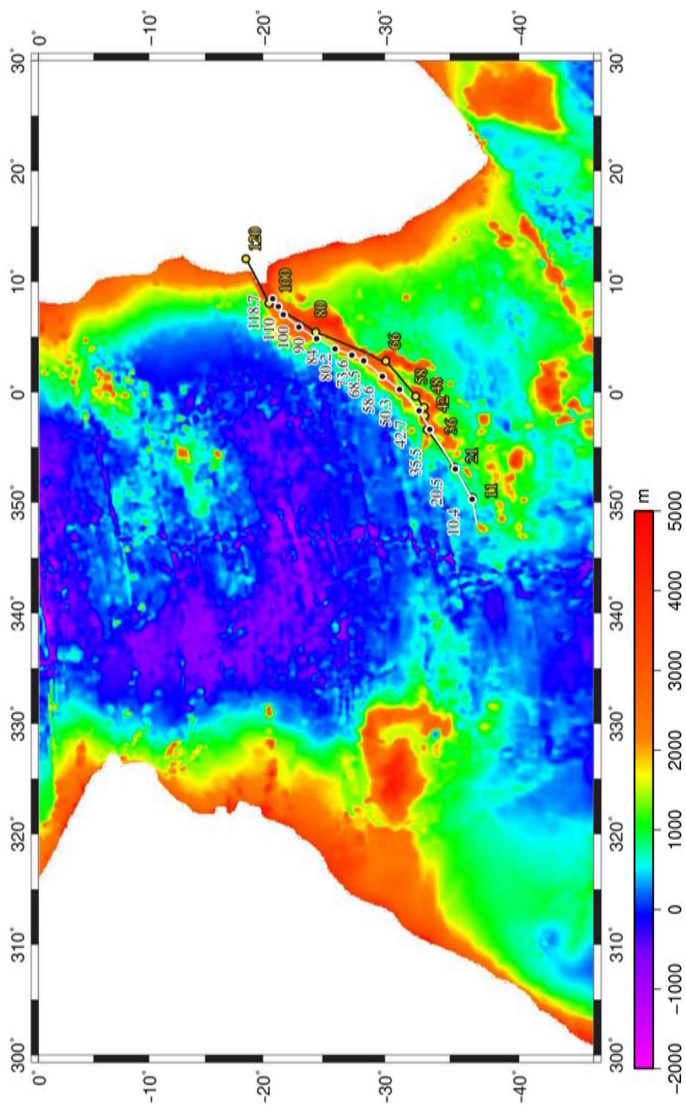
FIGURE 7.0.13: Carte de bathymétrie résiduelle avec la trace du point chaud de Tristan da Cunha selon les calculs avec les pôles de Duncan et Richards (1991) en noir et jaune et Muller et al. (1993) en blanc et noir. Pour chaque paléo position du point chaud est montré l'âge admis en Ma.
